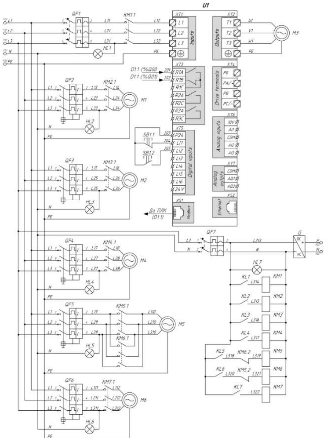
Рис. 5.1. Система автоматичного керування шахтною зерносушаркою
