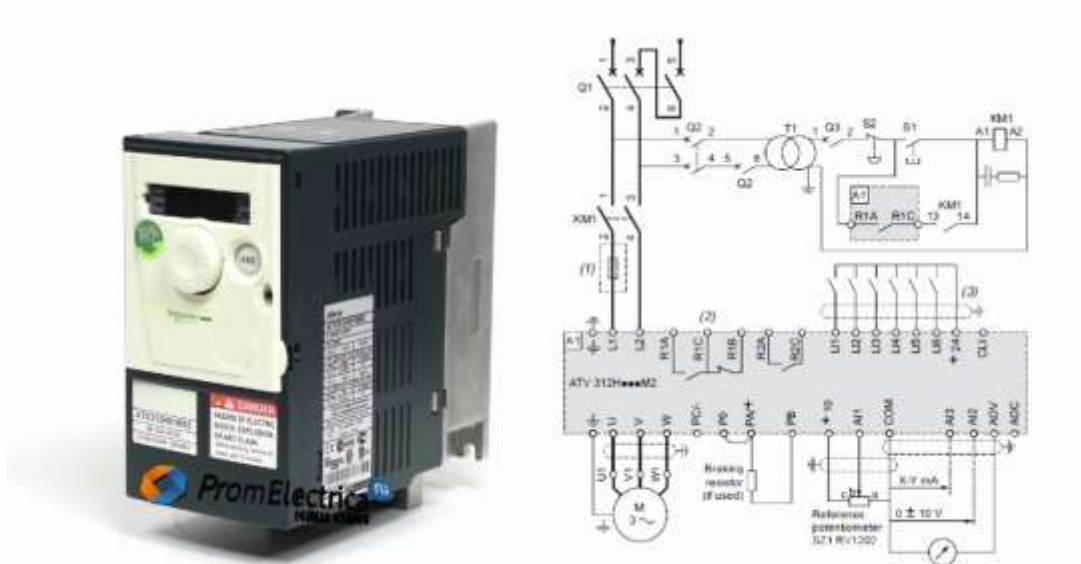
Рис. 3.6. Зовнішній вигляд перетворювача частоти Altivar ATV312 фірми Schneider Electric
