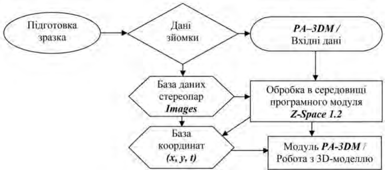
Рис. 3.2. Технологічний ланцюг отримання тримірної теплофізичної моделі
