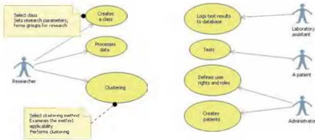
Рисунок 1. Use case діаграма системи кластеризації
