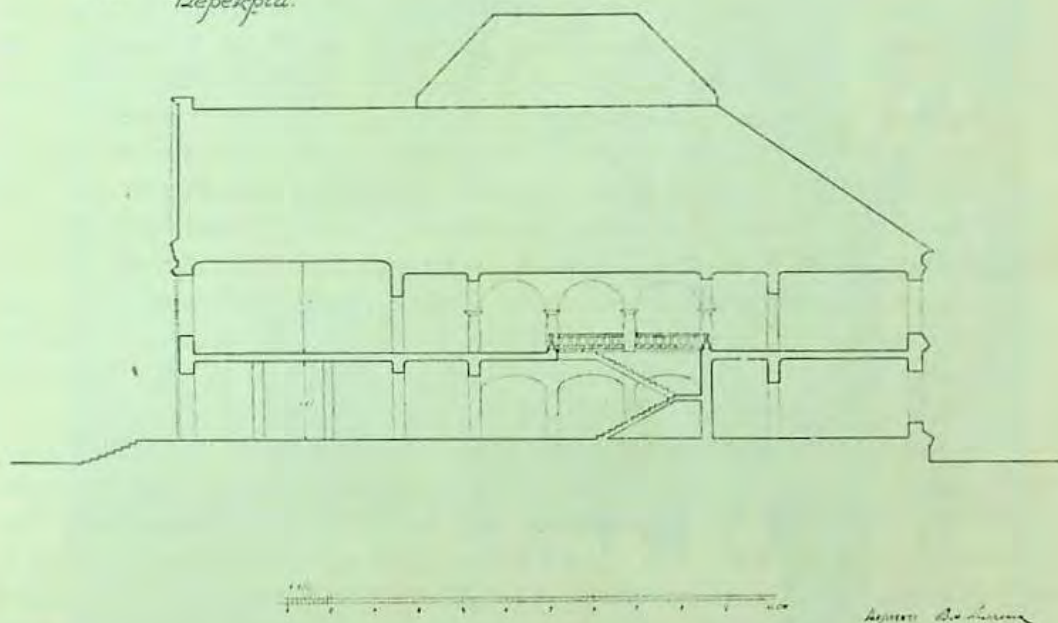
Проект лісфаку КСГІ. Перекрій.
