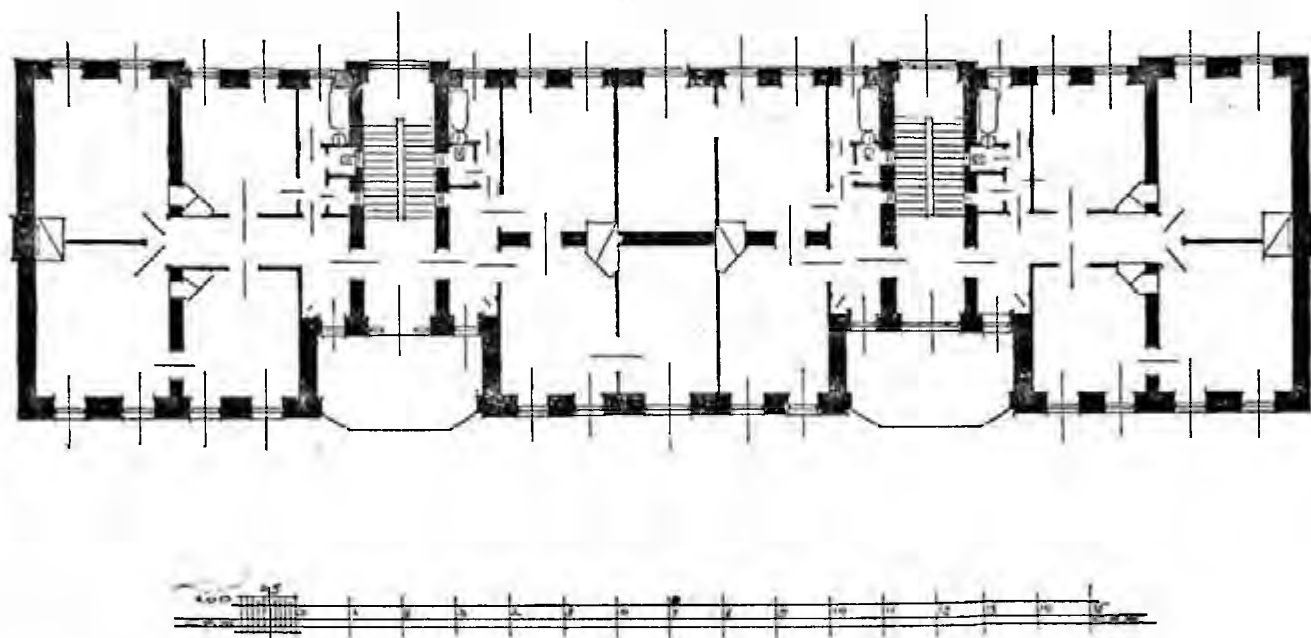
Житловий будинок для професури на 12 помешкань (варіант). План I—III поверху.
