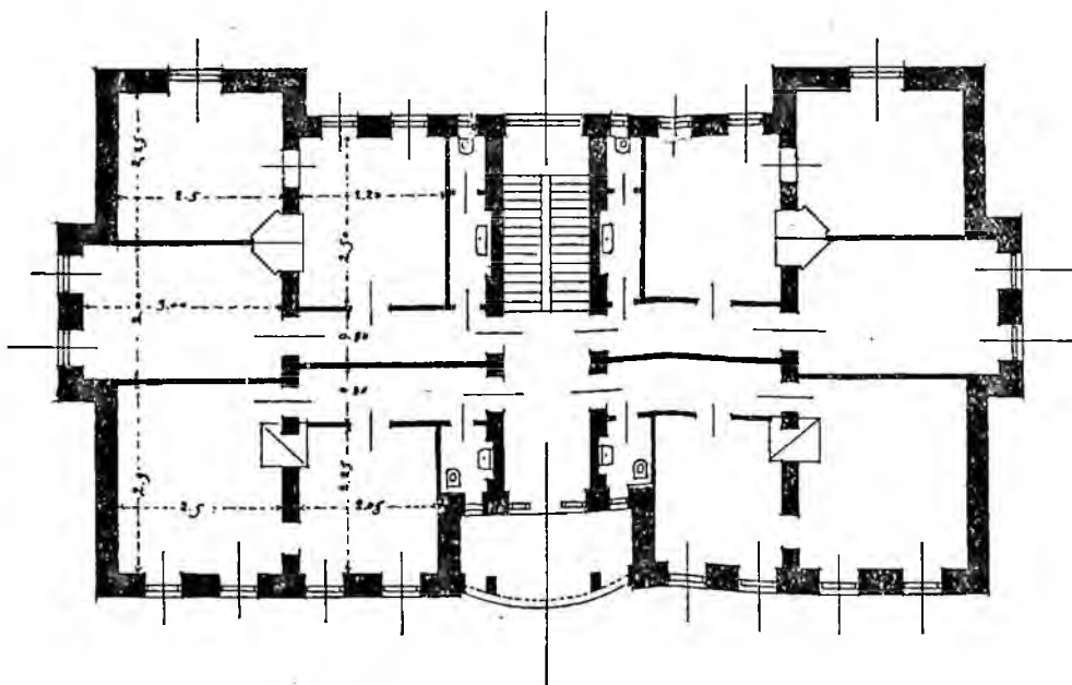
Житловий будинок для професури на 8 помешкань— план I—II поверху.
