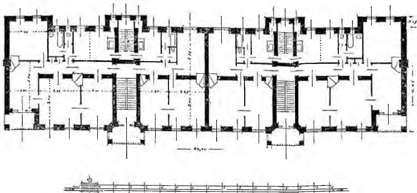
Житловий будинок для професури на 12 помешкань. План I—III поверху.
