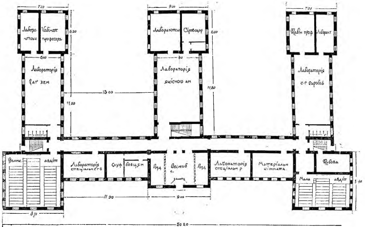
Будинок с.-г. хемії—план I-го поверху
