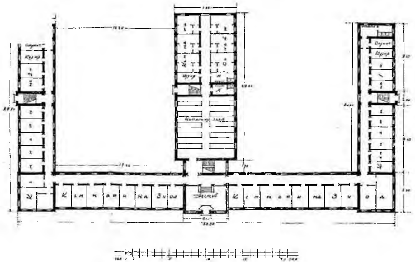
Бурса студенська—план I поверху.
