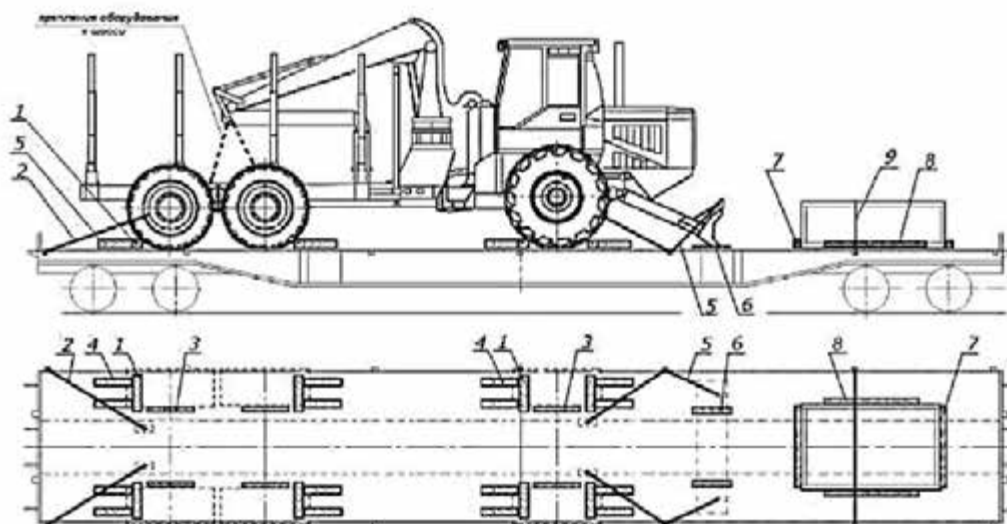
Рис. 2.4. Розміщення та кріплення на платформі техніки з навісним обладнанням
