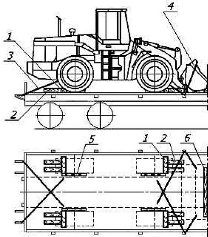
Рис. 2.5. Схема комбінованого кріплення техніки на платформі:
