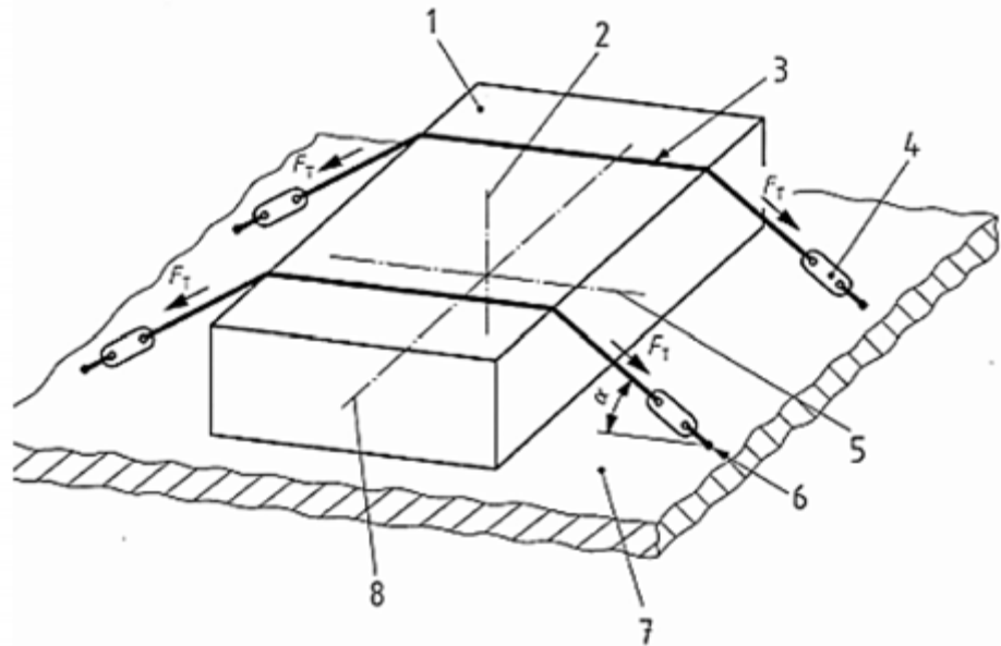
Рис. 3.9. Кріплення вантажу силовим способом
