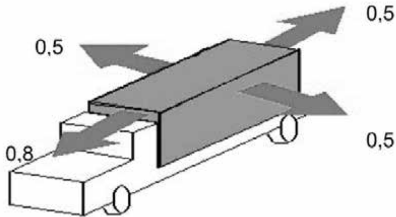
Рис. 3.8. Розподіл сил, що діють на вантаж
