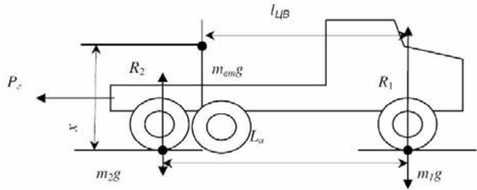
Рис. 3.14. Схема для розрахунку максимального навантаження
