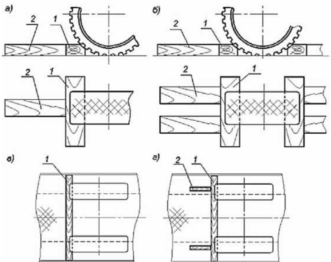
Рис. 2.3. Схеми блокування коліс
