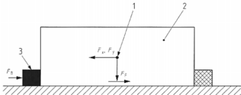
Рис.3.10. Кріплення вантажу блокуванням
