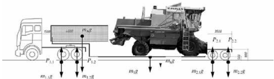
Рис.3.7. Схема дії сил і реакцій авто потяга:
