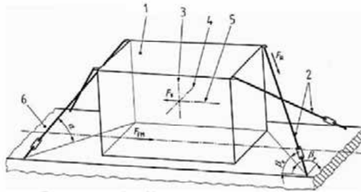
Рис. 3.11. Кріплення по діагоналі
