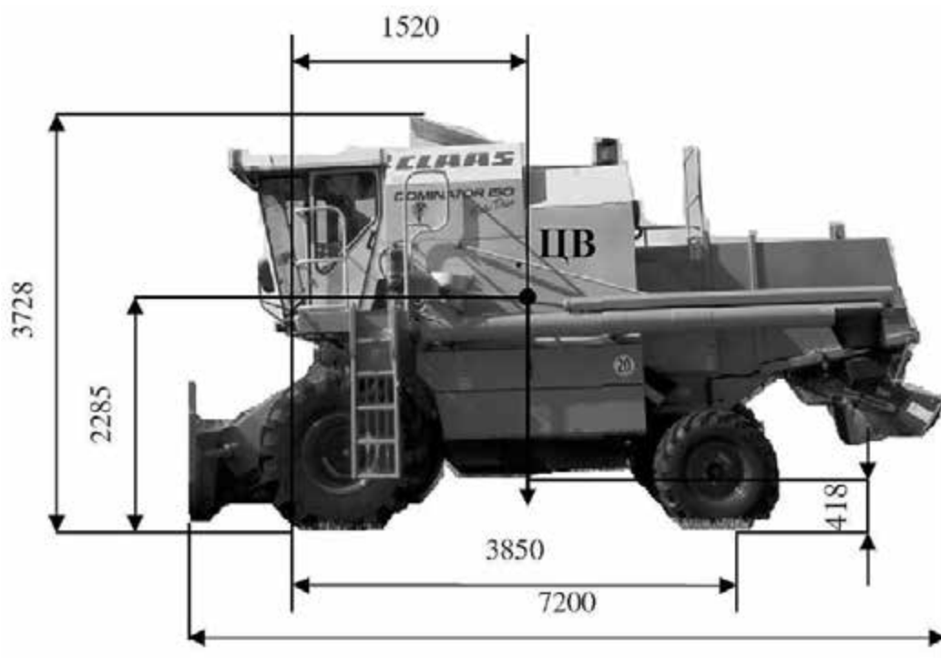
Рис. 3.6. Транспортні розміри зернозбирального комбайна Claas
