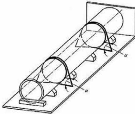
Рис. 3.12. Кріплення петлею
