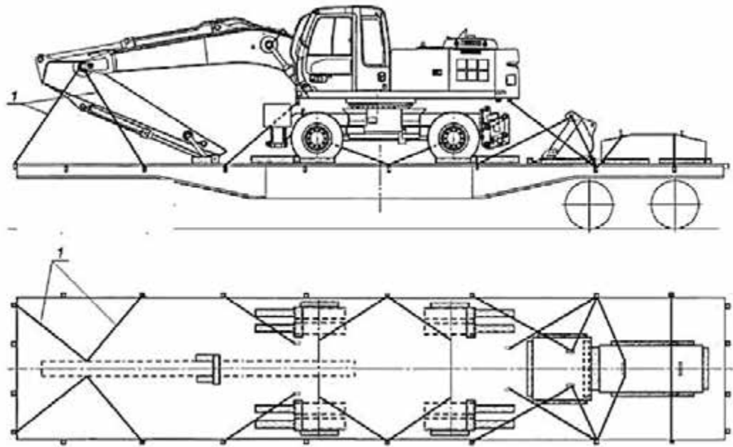
Рис. 1.2. Схема розміщення і кріплення спецтехніки з поворотними частинами до напівпричепу
