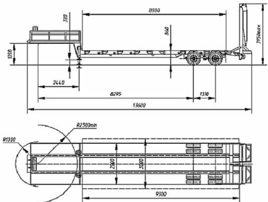
Рис. 3.2. Основні розміри причепа ОДА3-830030
