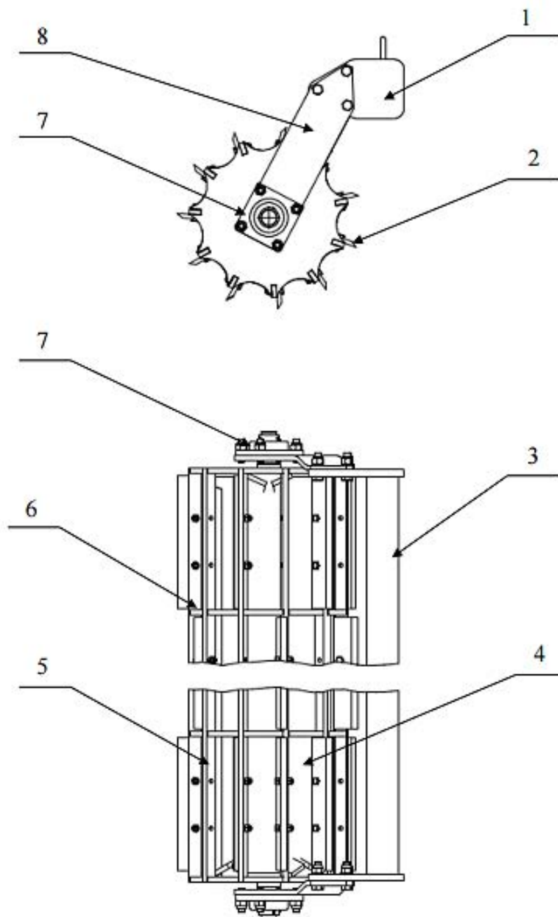
Рис. 3.4. Загальний вид розробленої конструкції катка-подрібнювача:
