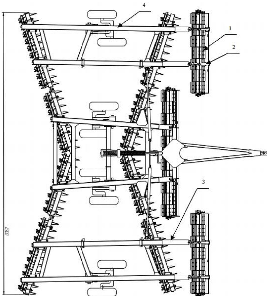
Рис. 3.1. Удосконалена конструкція дискової борони John Deere 637:
