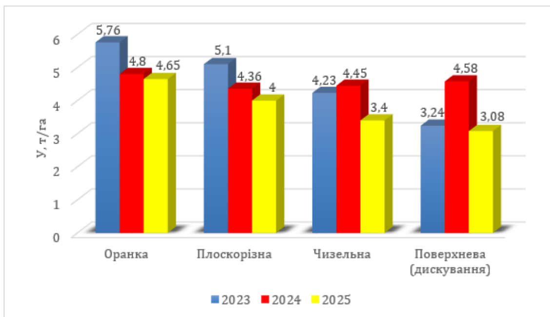
Рис. 2.5. Вплив методу обробітку ґрунту на врожайність ярого ячменю
