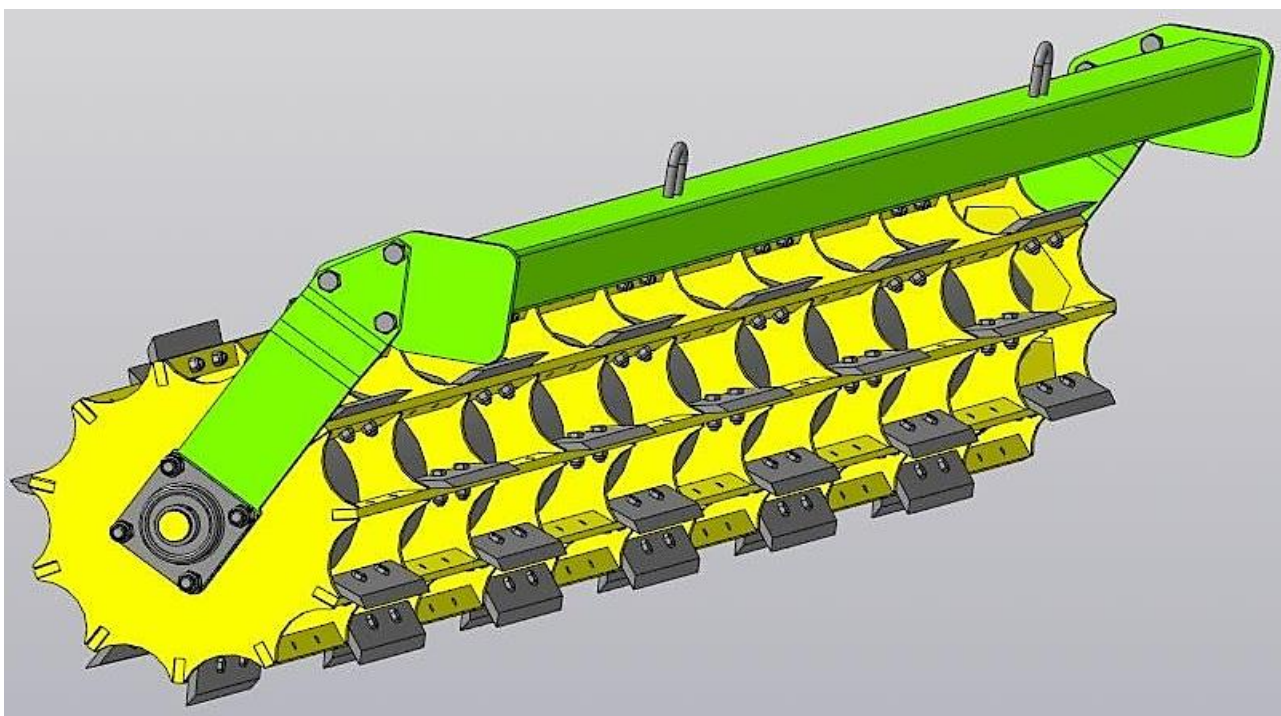
Рис. 3.2. Каток-подрібнювач
