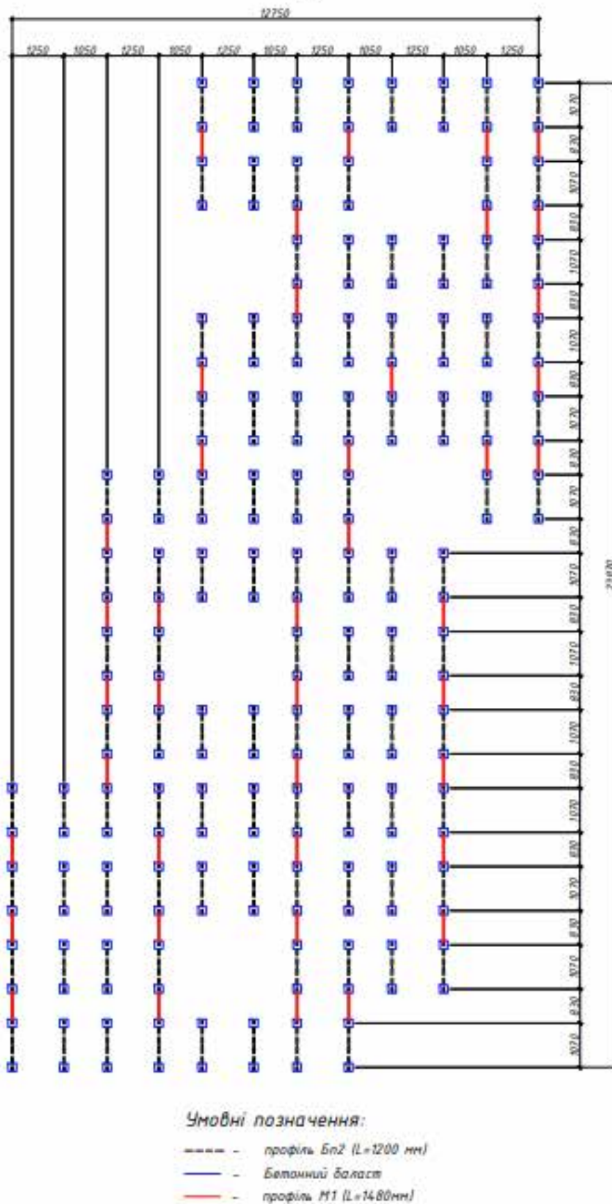
Рис. 3.8. Схема розташування баластів та роз'єднувачів М1
