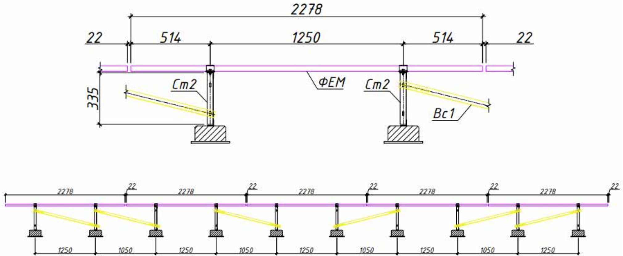
Схематичне зображення розкосів Вс1.
