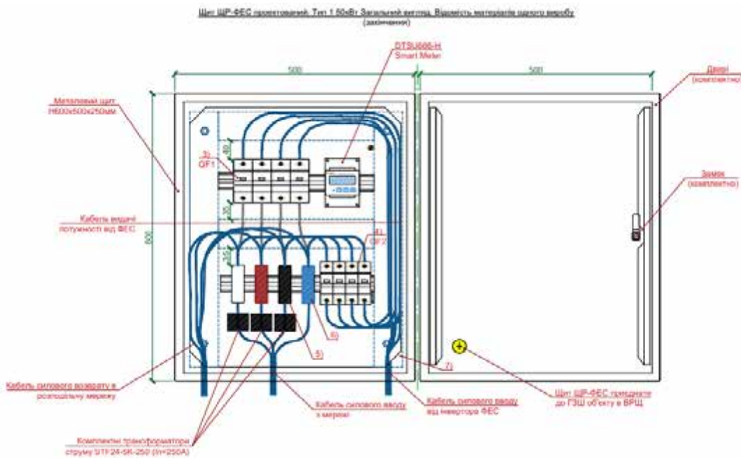
Рис. 3.12. Щит РЩ-ФЕС
