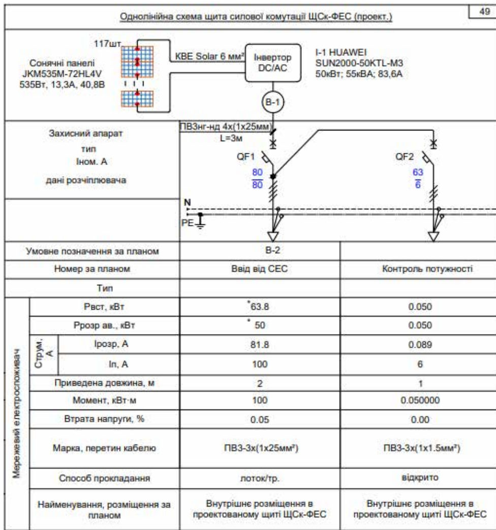
Рис. 3.11. Однолінійна схема щита силової комутації ЩСк-ФЕС
