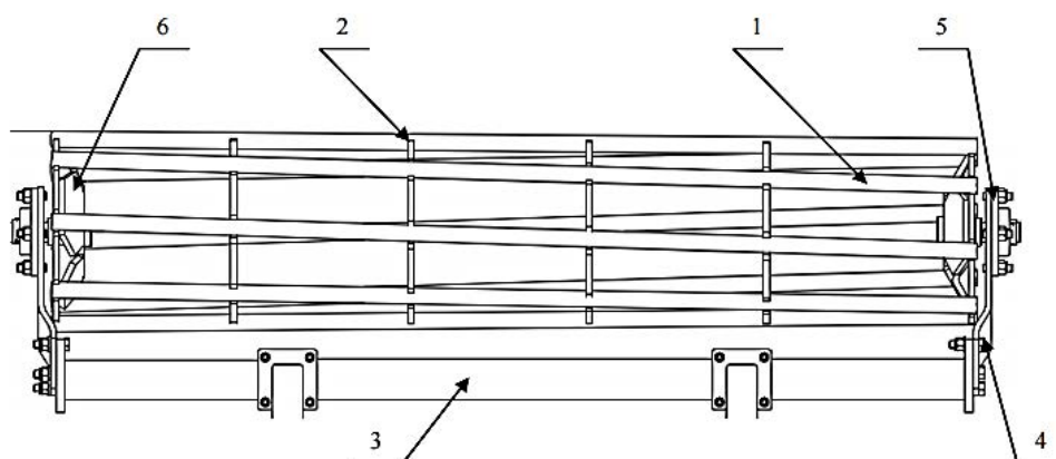
Рис. 3.3. Коток секція 2 м:
