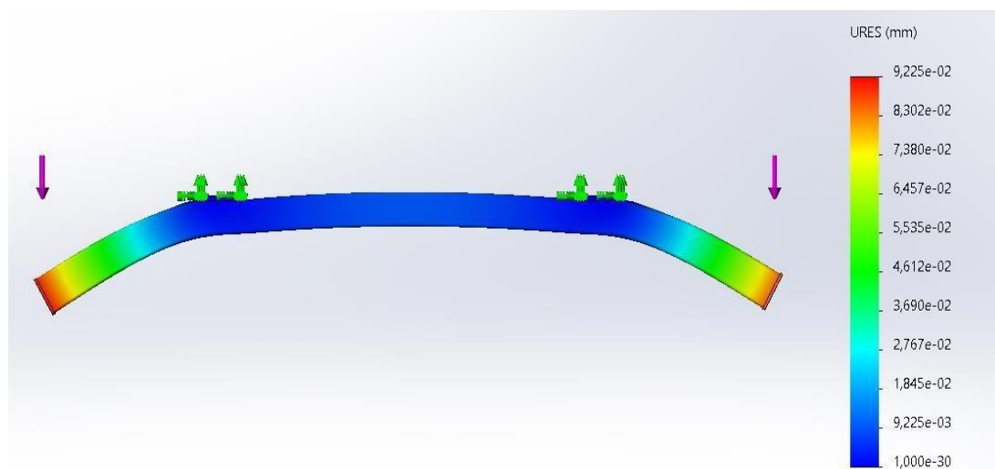
Рис. 3.7. Переміщення під дією прикладеної сили до досліджуваної балки
