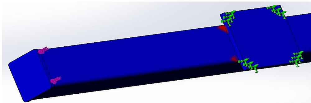
Рис. 3.6. Місце (позначене червоним) втрати міцності при перевищенні запасу для обраного матеріалу у 30 разів
