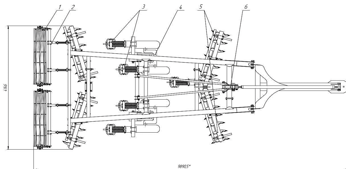
Рис. 3.2. Загальний вид удосконаленого розпушувача John Deere 512
