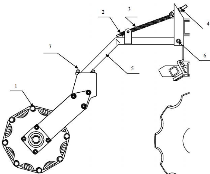
Рис. 3.4. Прикочуючий каток із механізмом його захисту від перевантажень та регулювання:
