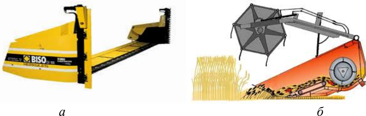
Рис. 2.11 – Жниварки для збирання ріпаку а – ріпаковий стіл фірми «Biso»; б – схема жниварки Power Flow комбайнів Massey Ferguson
