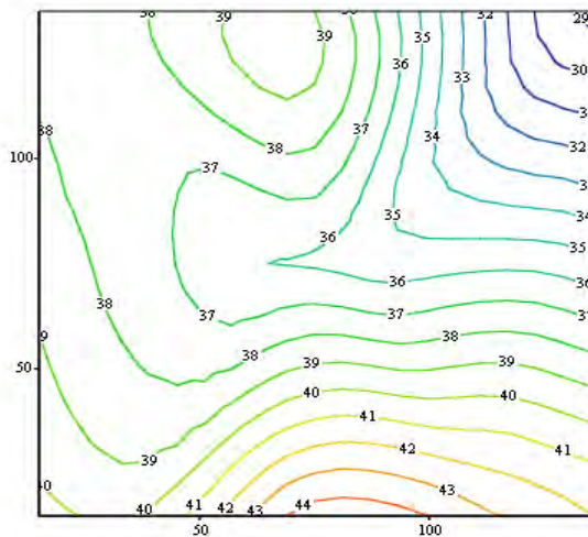
Рис. 2.9. Градієнт температури для поверхні теплообміну на виході з ТА: а – графік поверхні градієнта; б – графік ізотерм
