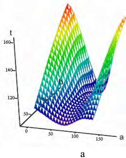
Рис. 2.8. Градієнт температури для поверхні теплообміну на вході в ТА: а – графік поверхні градієнта; б – графік ізотерм
