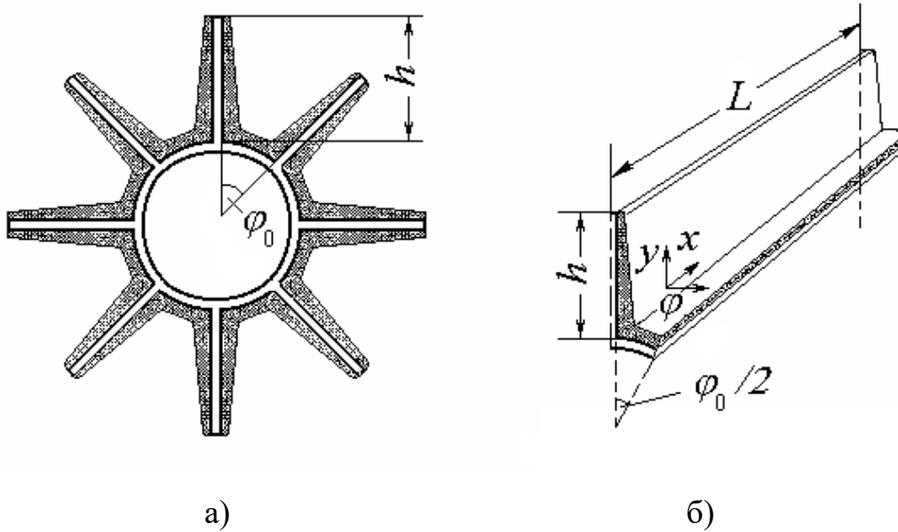
Рис. 4.23. Розрахункова схема ребреної труби з нерівномірними відкладеннями: а) поперечний переріз труби; б) елементарна ділянка ребрення
