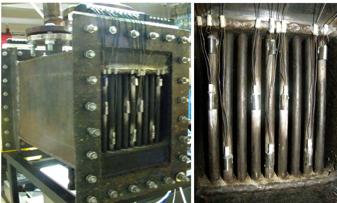
Рис. 2.6. Розташування термопар на вході в ТА
