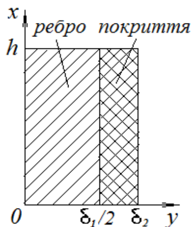
Рис. 4.14. Розрахункова схема ребра з покриттям
