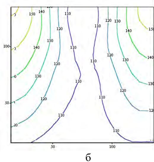
Рис. 2.8. Градієнт температури для поверхні теплообміну на вході в ТА: а – графік поверхні градієнта; б – графік ізотерм
