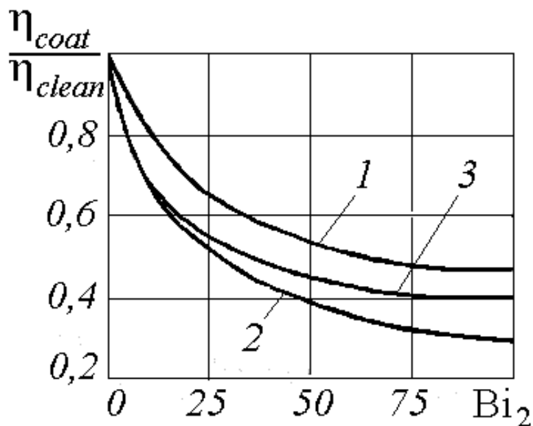
Рис. 4.15. Залежність \eta_{coat} / \eta_{clin} від числа Біо покриття Bi_2 для ребер різного типу при \psi_{Bi} = 0,04 : 1 – повздовжнє ребро; 2 – кільцеве ребро; 3 – циліндричний шип
