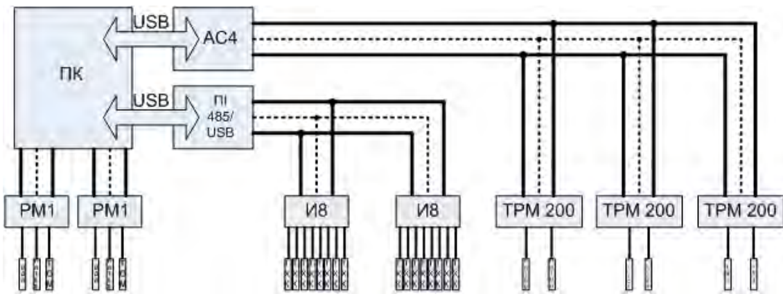
Рис. 2.5. Схема підключення приладів вимірювання і устаткування
