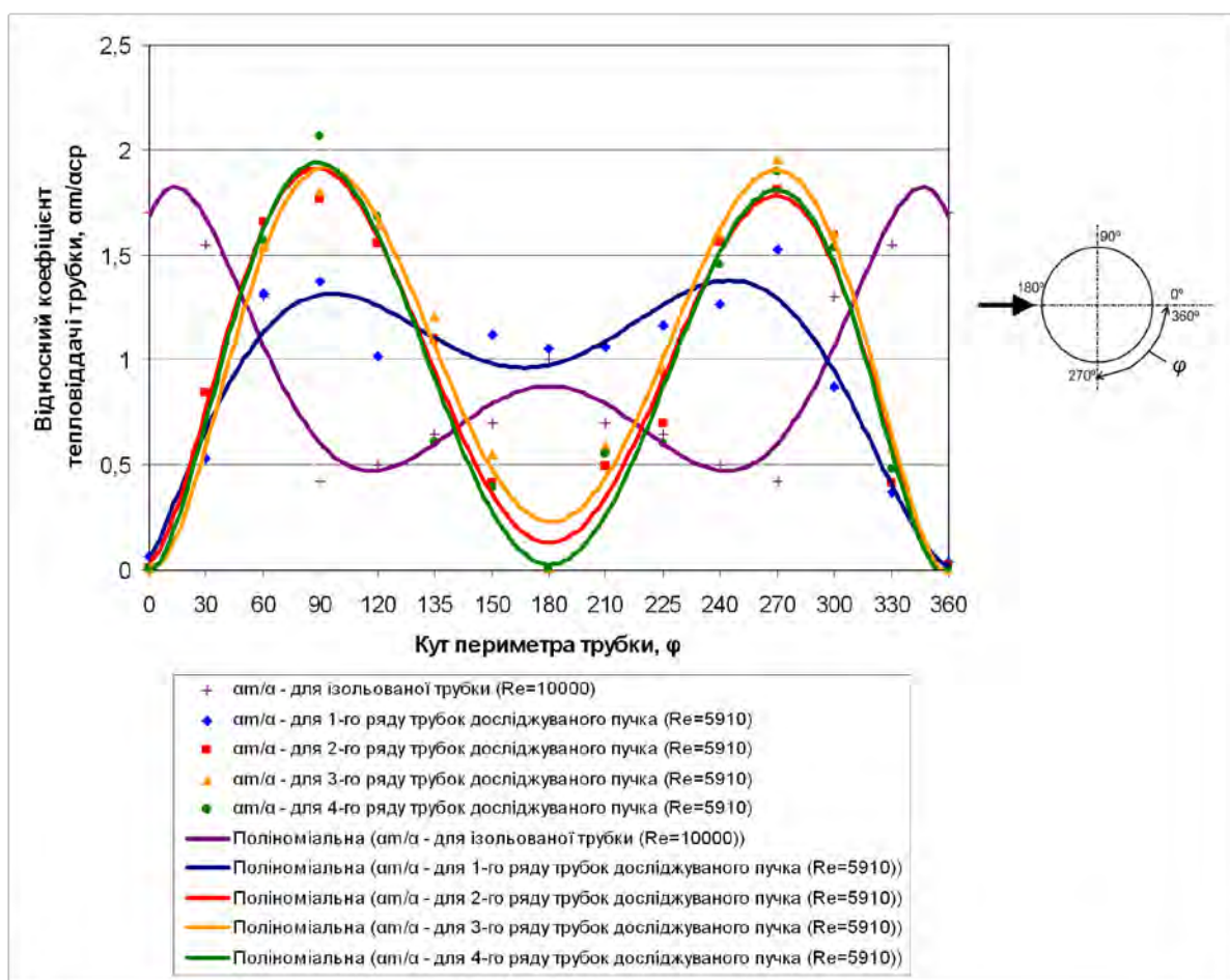
Рис. 3.28. Порівняльний графік апроксимуючих поліноміальних функцій розподілу відносного коефіцієнта тепловіддачі \alpha_m/\alpha на поверхні перших чотирьох труб поздовжнього ряду досліджуваного пучка a \times b = 1,5 \times 1,0 при Re = 6044 ; Pr = 0,692 ( n = 1500 \text{хв}^{-1} ) і
