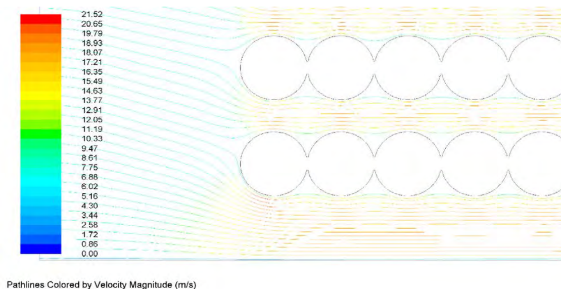
Рис. Б.6. Лінії течії, що відображають значення швидкостей відпрацьованих газів в каналах пучків трубок, м/с
