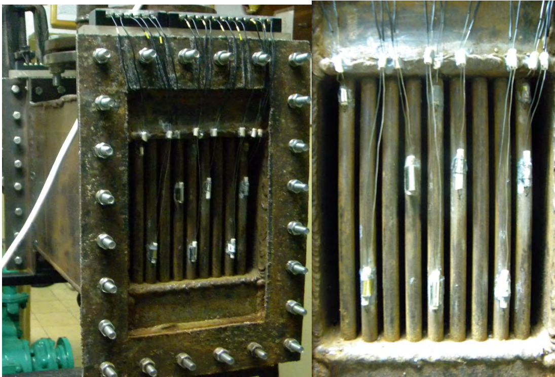
Рис. 2.7. Розташування термопар на виході з ТА
