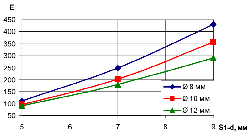
Рис. 3.18. Залежність теплогідралічної ефективності від геометрії пучка трубок
