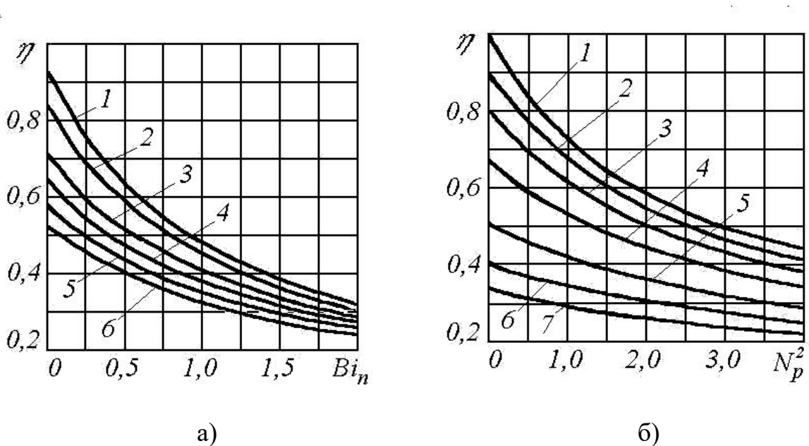
Рис. 4.17. Теплова ефективність кільцевого ребра з рівномірним покриттям малої провідності: а) 1 – N_p^2 = 0,2 ; 2 – 0,5; 3 – 1,0; 4 – 1,5; 5 – 2,0; 6 – 2,5; б) 1 – Bi_n = 0,2 ; 2 – 0,1; 3 – 0,25; 4 – 0,5; 5 – 1,0; 6 – 1,5; 7 – 2
