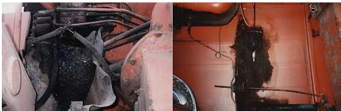
Рис. 3.5. Конструктивний недолік - підтікання оливо і палива із стиків з'єднань трубопроводів.
