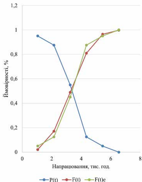
Рис. 3.14. Експериментальна функція розподілу F_e(t) , теоретична функція розподілу F_T(t) , та ймовірність безвідмовної роботи машини P(t)
