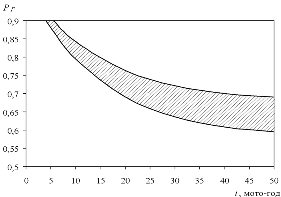
Рис. 2.5. Графік залежності ймовірності готовності комбайна до роботи P_G від наробітку t і часу відновлення працездатності t_\epsilon
