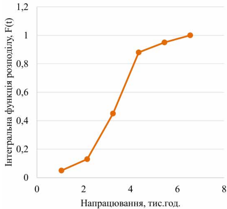
Рис. 3.13. Інтегральна функція наробітку комбайнів
