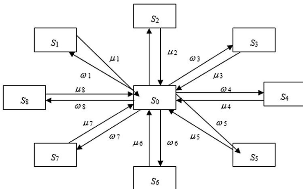
Рис. 2.4. Графік можливих переходів зернозбирального комбайна із працездатного стану S_0 в стан відмови однієї з підсистем S_i
