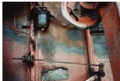
Рис. 3.7. Попадання сторонніх предметів під шнек жатки.
