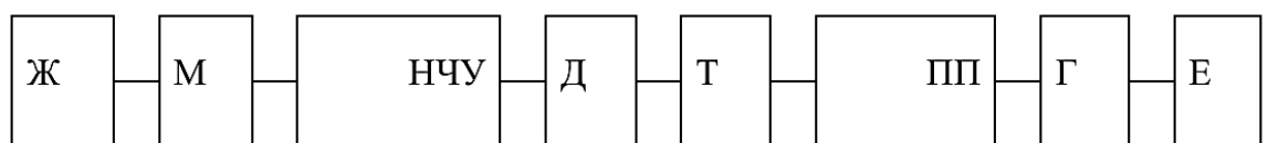
Рис. 2.3. Схема з'єднання складових підсистем зернозбирального комбайна:
