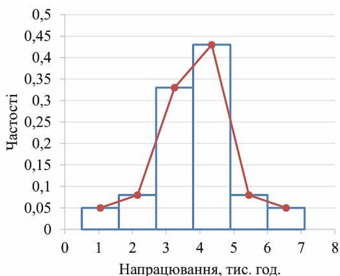
Рис. 3.12. Зображення гістограми та полігона в загальному вигляді
