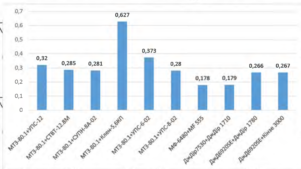
Фиг. 3.3.1. Затрати праці конкуруючих МТА на сівбі кукурудзи в ТОВ «Нива Переяславщини»
