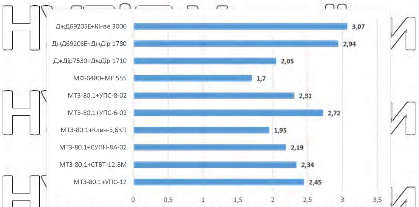
Рис. 3.3.2. Продуктивність конкуруючих МТА на сівбі кукурудзи в умовах ТОВ «Нива Переяславщини»
