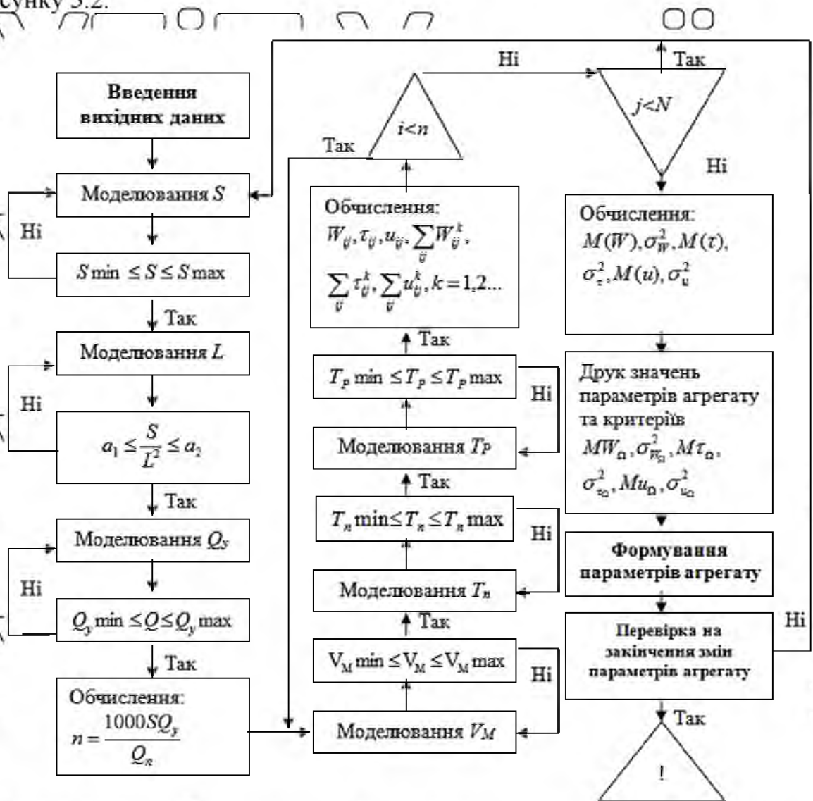
Рис. 3.2 – Алгоритм статистичного моделювання експлуатаційно-економічних показників машинних агрегатів
