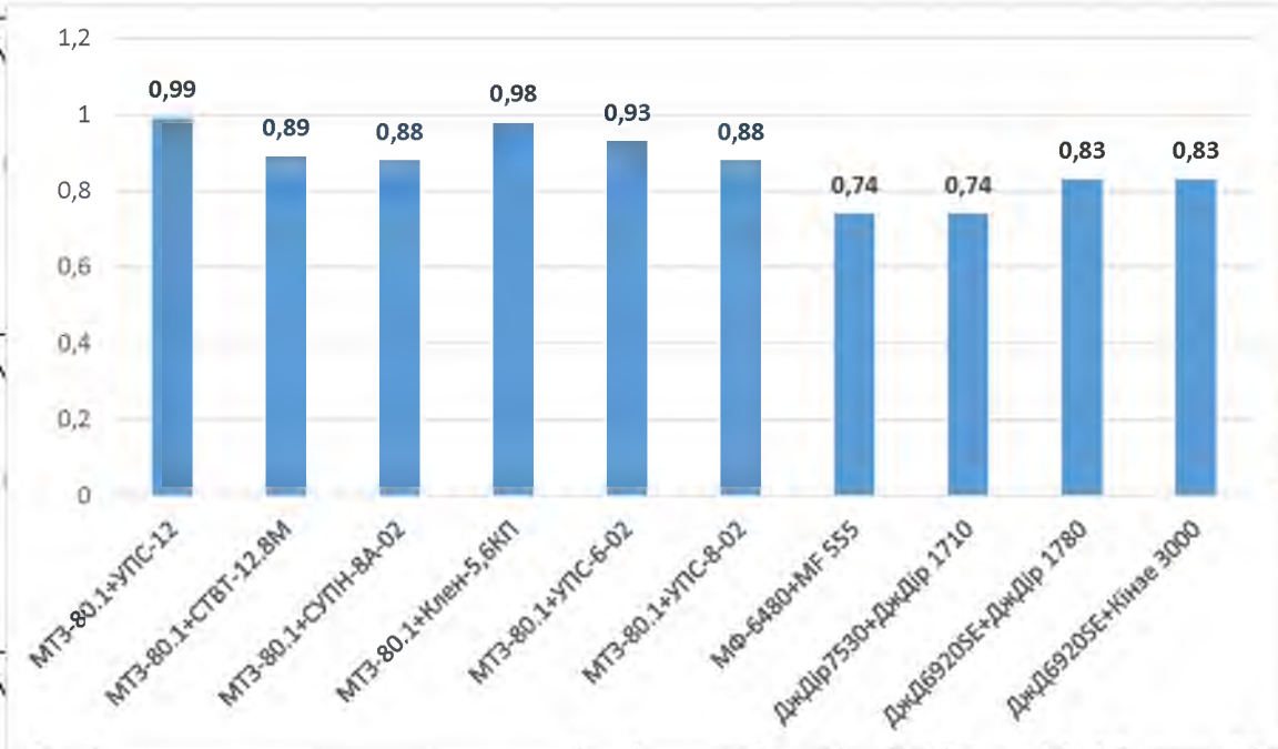
Рис. 3.3.4. Коефіцієнт використання агрегату конкуруючих МТА на сівбі кукурудзи в умовах ТОВ «Нива Переяславщини»
