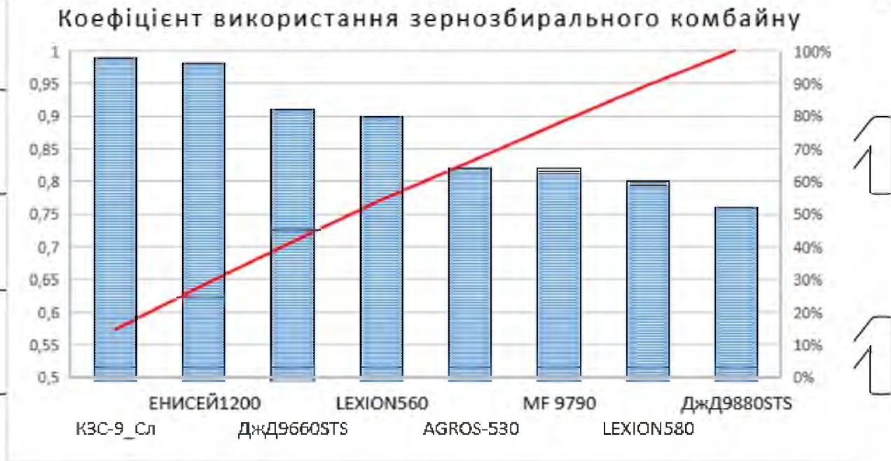
Рис. 3.3.8. Коефіцієнт використання конкуруючих зернозбиральних комбайнів на збиранні кукурудзи в умовах ТОВ «Нива Переяславщини» (пряме комбайнування).
