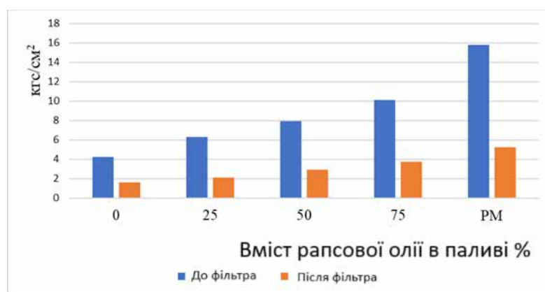
Рис. 1. Результати дослідження залежності тиску до і після фільтра тонкої очистки палива від вмісту ріпакової олії в дизельному паливі.
