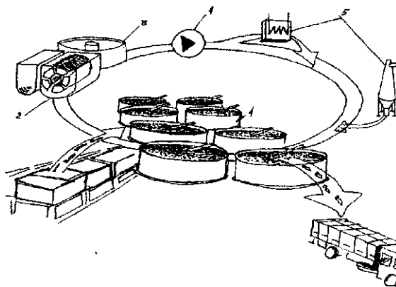
Мал. 62. Схема установки «Штеллерматик» 1 — рибоводні басейни; 2 — окислювальний басейн; 3 — басейн-відстійник; 4 — насосна група; 5 — терморегуляція та оксигенація
