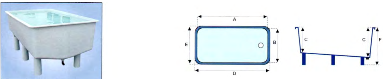
Мал. 44. Спеціальний басейн на ніжках для осетрових риб, з ухилом дна
