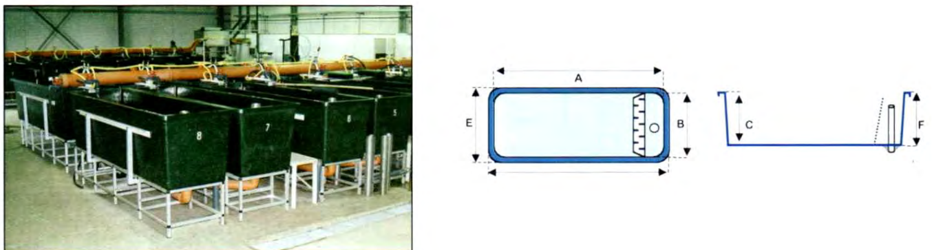
Мал. 45. Лотки з плоским дном, без ніжок
