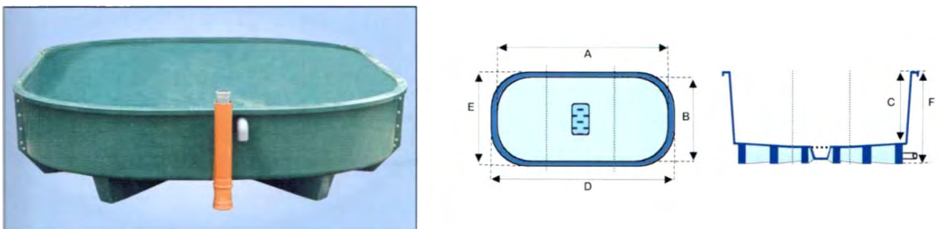
Мал. 52. D-подібний сегментний басейн з ухилом дна, стічною трубою та прямком для фекалій
