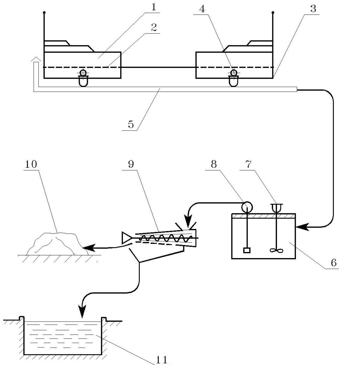
Рис.21. Технологічна схема видалення і переробки гною
