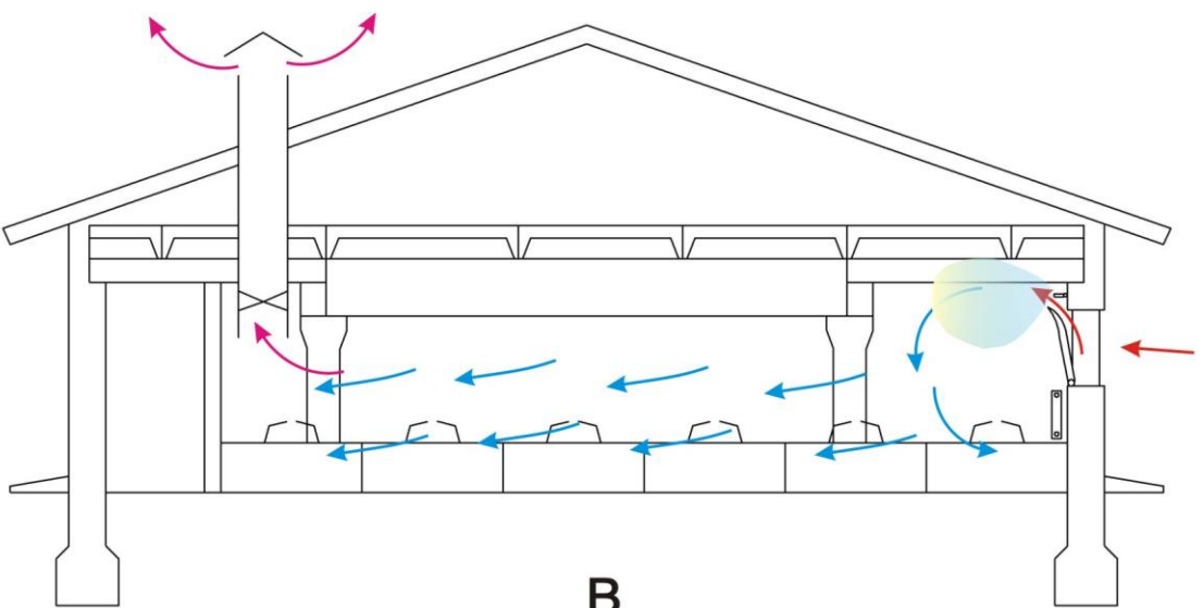
Рис.19. Схема вентиляції (а), водяного опалювання (б) і кондиціонування (в) на прикладі секції для опоросу
