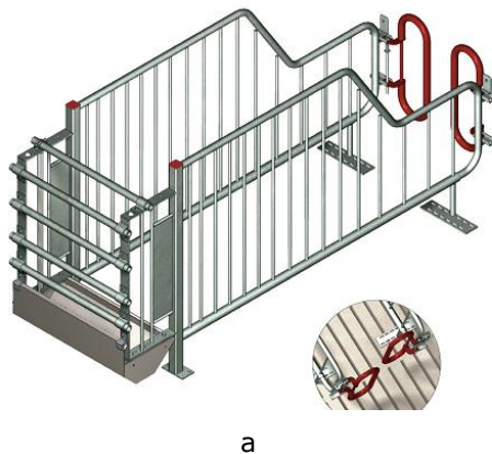
Рис. 7. Загальний вигляд станка (а) і секції (б) для індивідуального утримання свиноматок
