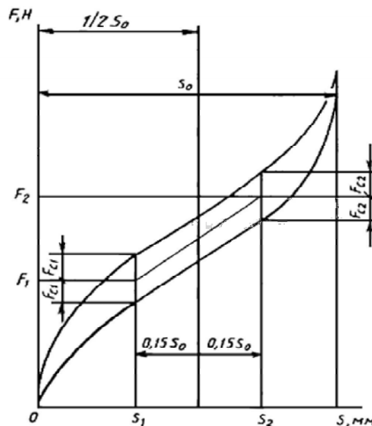
Рис.1.1 – Пружна характеристика підвіски сидіння
