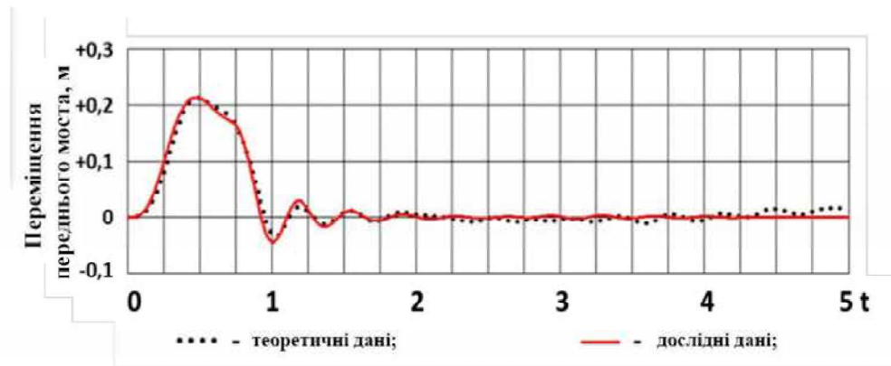
Рис. 4.9 – Вертикальні переміщення переднього моста
