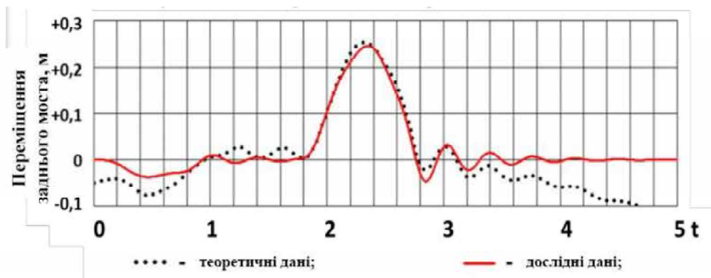
Рис. 4.11 – Вертикальні переміщення заднього моста
