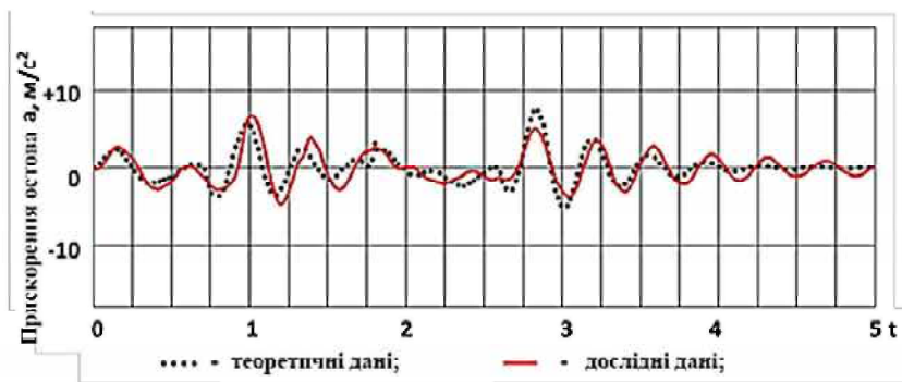
Рис. 4.4 – Прискорення остова під час переїзду одиначної нерівності
