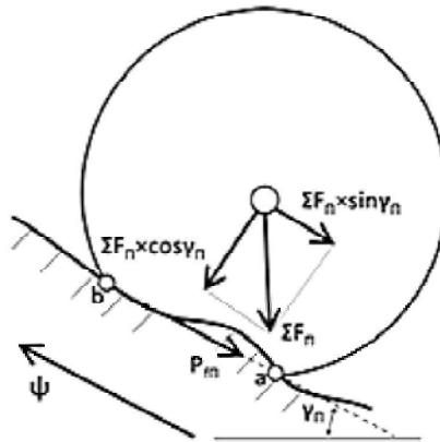
Рис. 2.4 – Схема сил, що діють на передній міст трактора
