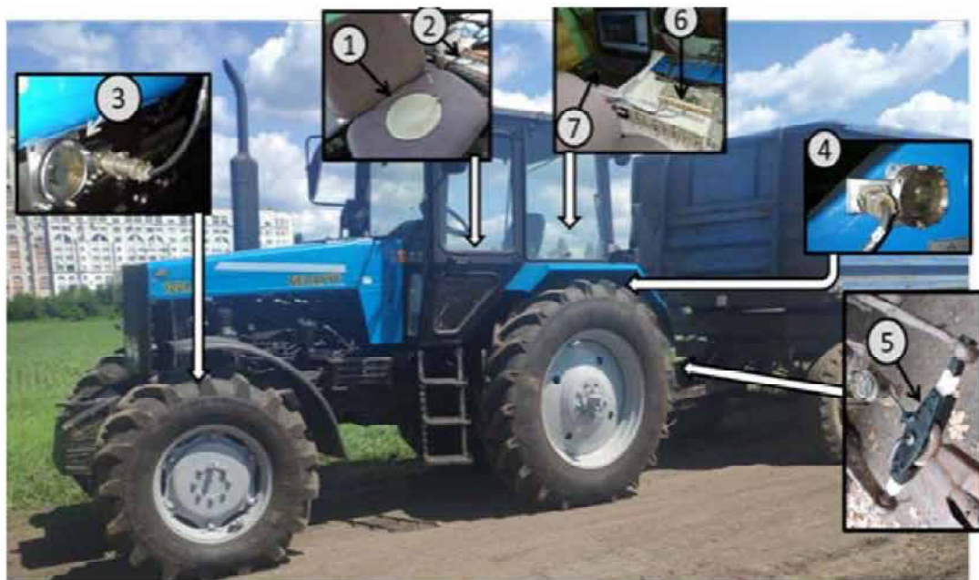
Рис. 3.12 – ТТА з обладнанням на польових випробуваннях: 1 - посадковий диск з ІСР датчиком; 2 - з'єднувальні кабелі; 3 - тензOMETричний віброакселерометр переднього моста трактора; 4 - тензOMETричний віброакселерометр заднього моста трактора; 5 - тягова тензобалка; 6 - тензопідсилувач; 7 - комп'ютер
