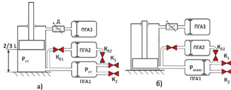
Рис. 2.14 – До розрахунку мінімального робочого об'єму ПГА1: а) у положенні статичної рівноваги; б) у положенні максимального стиснення підвіски
