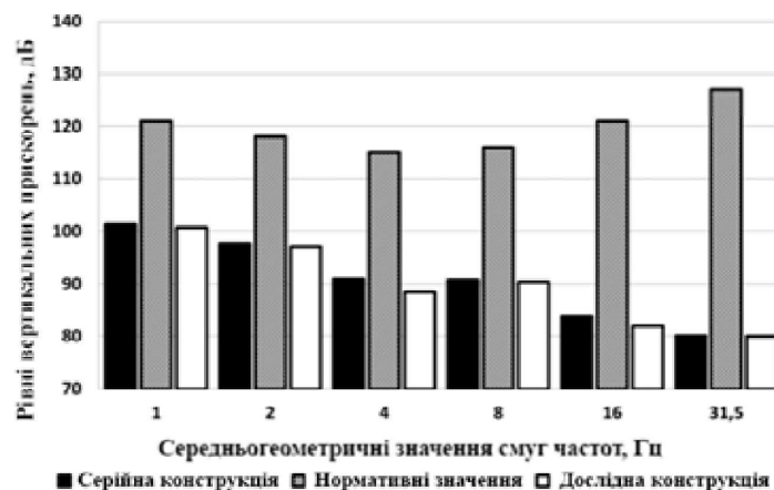
Рис. 4.15 – СКЗ вертикальних прискорень в октавних смугах частот під час руху ТТА у складі ХТЗ-1221.2 + 2ПТС-6 зі швидкістю 5 км/год
