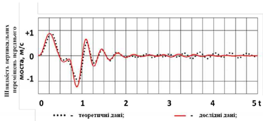
Рис. 4.6 – Швидкість вертикальних переміщень переднього моста під час переїзду одиначної нерівності
