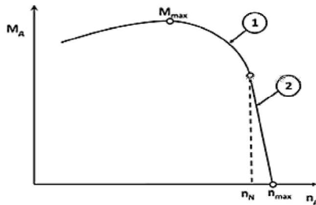
Рис. 2.6 – Характерний вигляд зовнішньої швидкісної характеристики дизельного ДВЗ: 1 - коректорна гілка; 2 - регуляторна гілка
