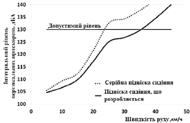
Рис. 2.18 – Залежність інтегрального рівня вертикальних прискорень від швидкості руху за використання серійної та дослідної конструкцій підвісок сидінь
