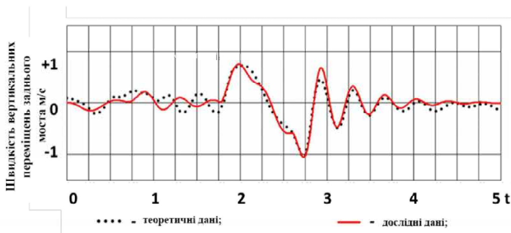
Рис. 4.8 – Швидкість вертикальних переміщень заднього моста під час переїзду одиначної нерівності
