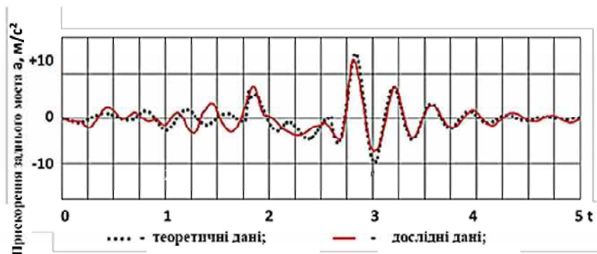
Рис. 4.5 – Прискорення заднього моста під час переїзду одиначної нерівності
