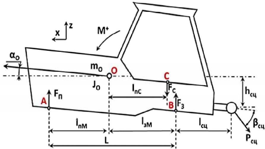
Рис. 2.2 – Схема сил і моментів, що діють на остов трактора у складі ТТА
