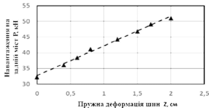
Рис. 4.2 – Залежність сили пружної деформації від прогину задніх шин
