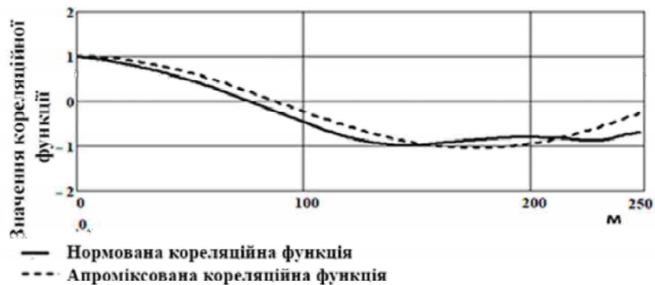
Рис. 3.13 – Значення нормованої та апроксимованої кореляційної функції
