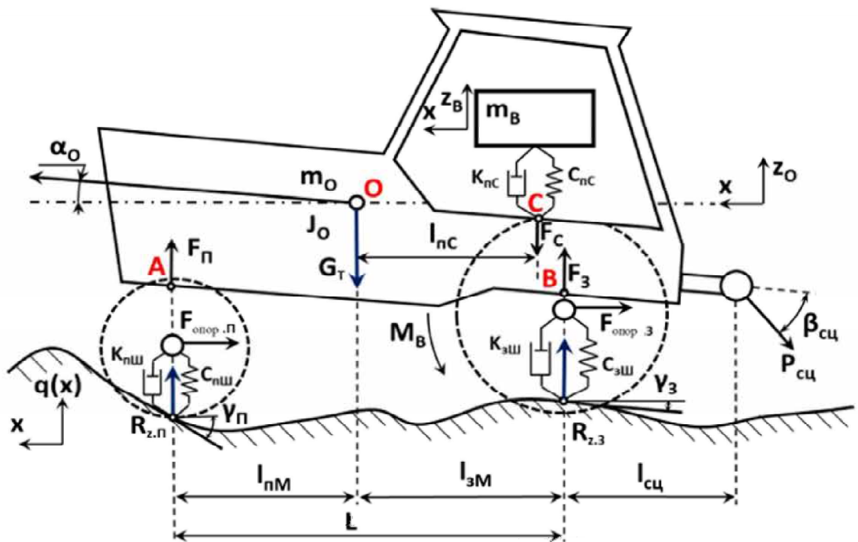
Рис. 2.1 – Загальна схема сил, що діють на трактор у складі ТТА
