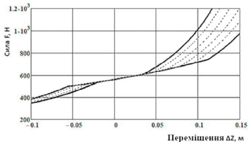
Рис. 2.17 – Варіації пружної характеристики розробленої конструкції підвіски сидіння при зміні моментів перемикання використовуваних ПГА
