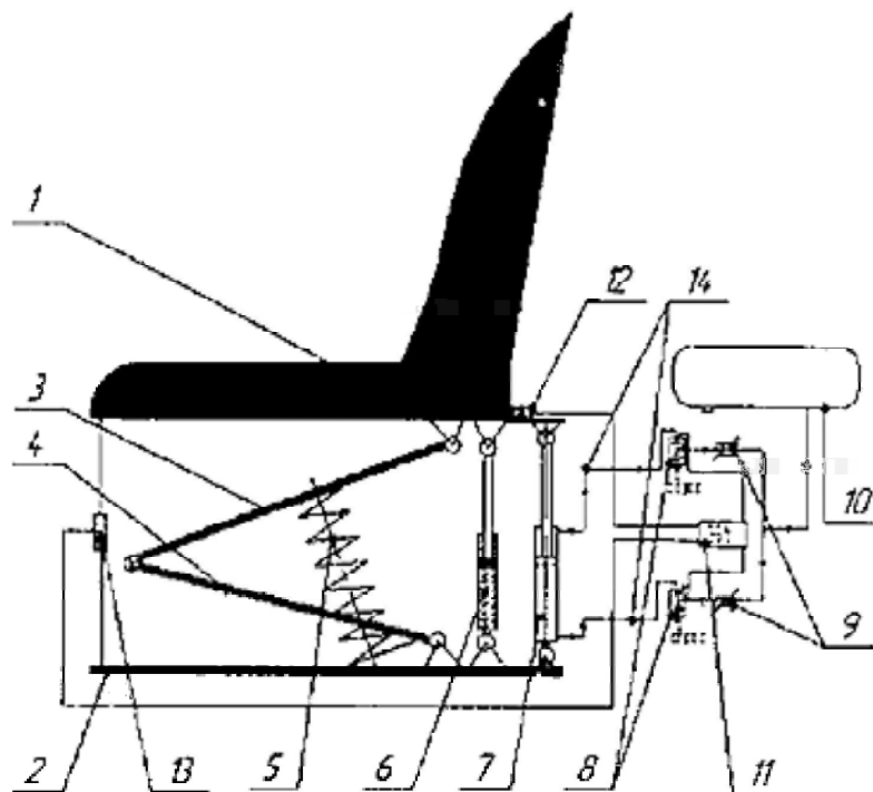
Рис. 1.8 – Адаптивна підвіска з активним пневмопоршневим пружним елементом: 1 – сидіння з подушкою і спинкою; 2 – основа; 3, 4 – верхня і нижня пара планок; 5 – циліндрична пружина; 6 – гідравлічний демпфер; 7 – активний пневмоелемент; 8 – електромагнітні клапани; 9 – дросель; 10 – ресивер; 11 – електронний блок керування; 12 – датчик вібрації; 13 – датчик положення; 14 – пневмомагістралі.
