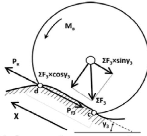
Рис. 2.7 – Схема сил, що діють на задній міст трактора
