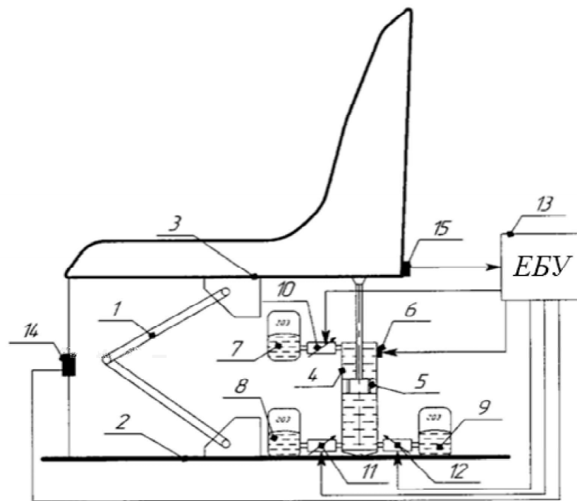
Рис. 1.12 – Адаптивна конструкція підвіски сидіння ТТА: 1 - напрямні планки; 2 - основа; 3 - подушка сидіння зі спинкою; 4 - гідравлічний демпфер; 5 - електромагнітна котушка; 6 - датчик демпфера (електронний перетворювач); 7, 8, 9 - пневмогідравлічні акумулятори; 10, 11, 12 - керовані дроселі; 13 - ЕБУ; 14, 15 - датчики вібрації
