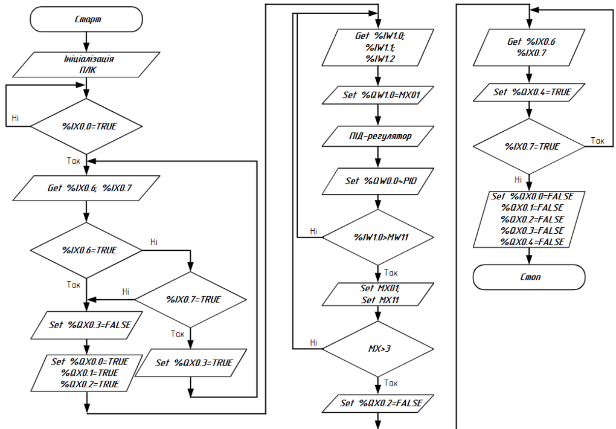
Рис. 6.3. Блок-схема основного алгоритму роботи САК диференційованими режимами активного вентилявання зерна в бункері БВ-40
