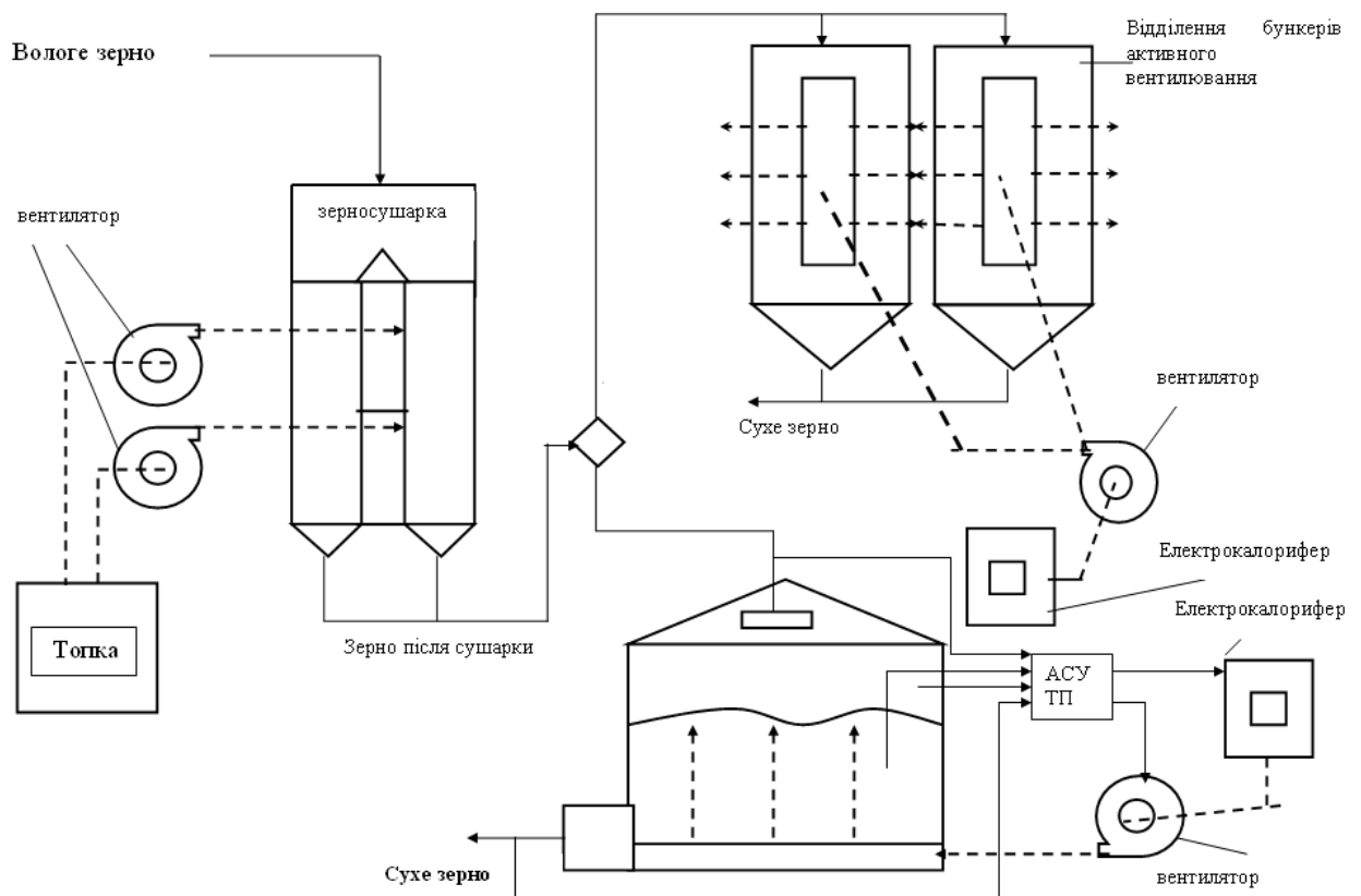
Рис. 2.1. Схема реалізації процесу двостадійного сушіння
