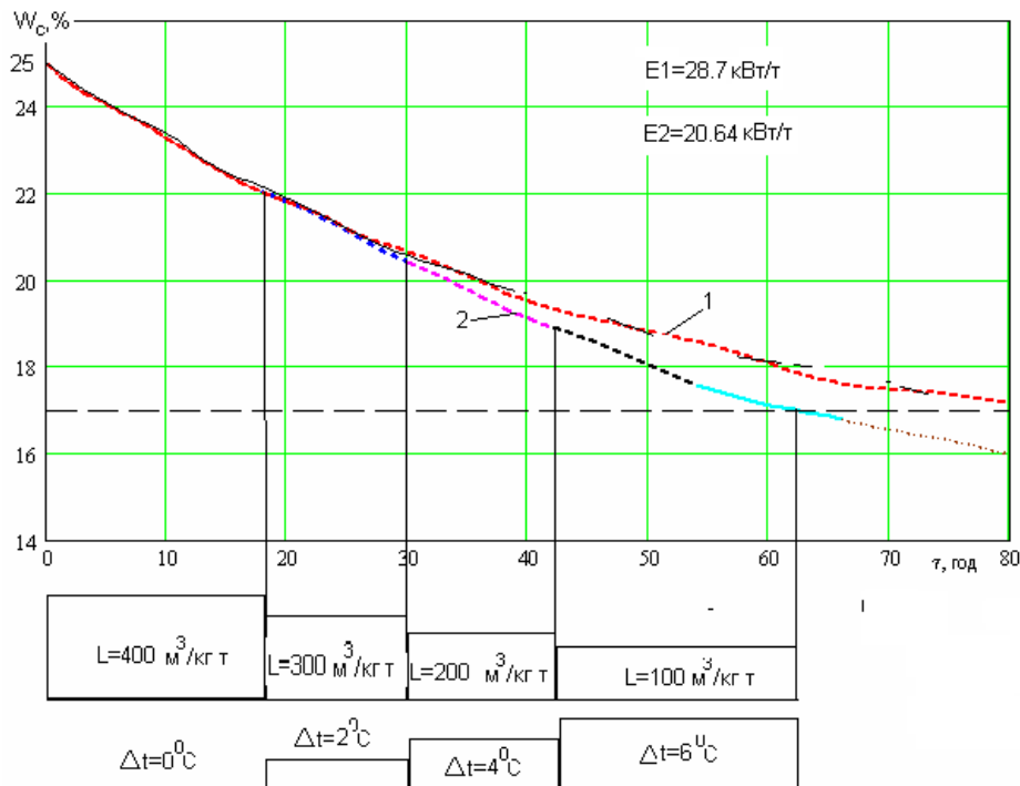
Рис. 3.13. Залежність зміннення вологи зерна в часі і технологічного регламенту (добова зміна температури повітря апроксимована
