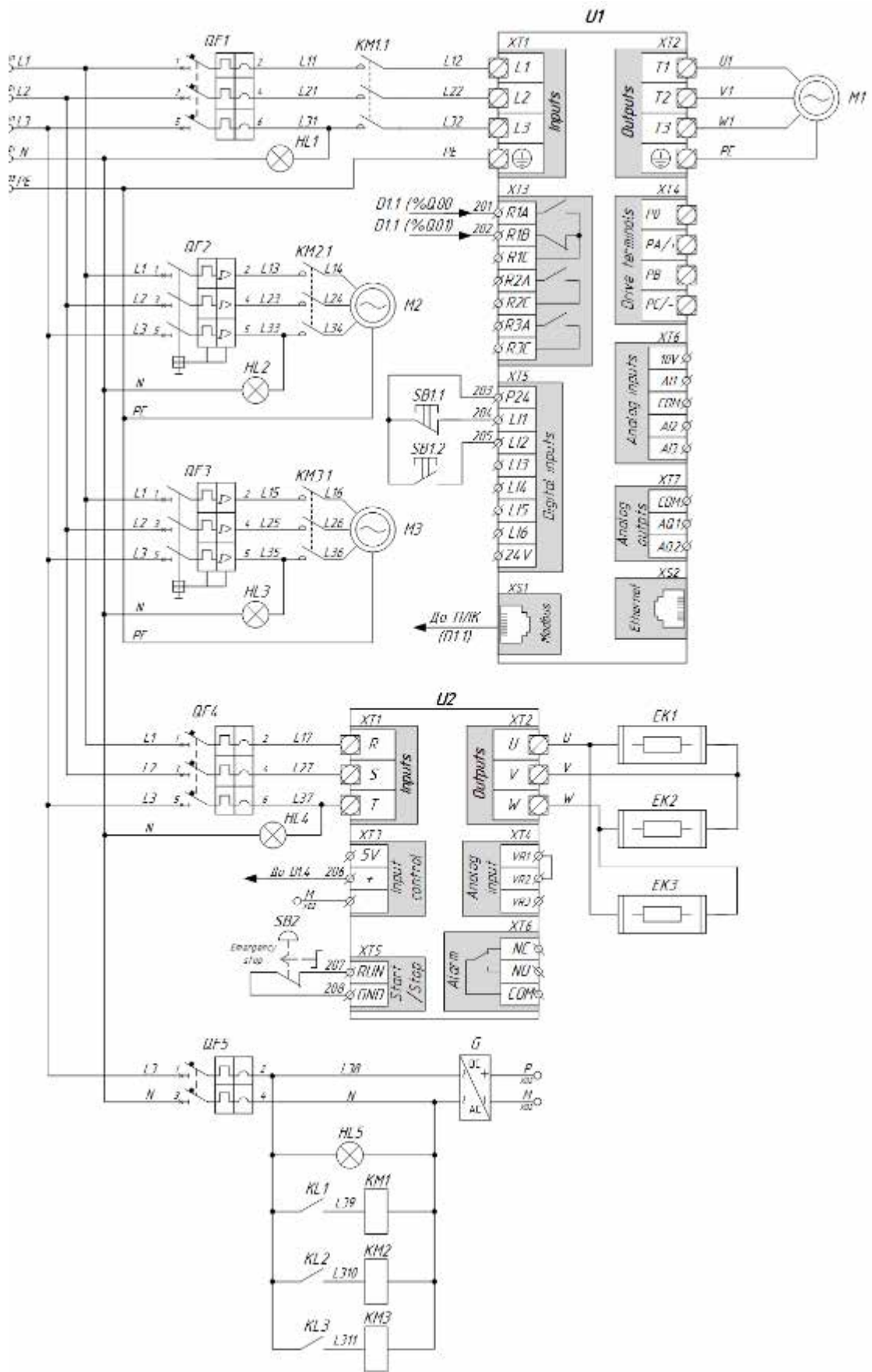
Рис. 6.1. САК диференційованими режимами активного вентилявання зерна в бункері БВ-40. Схема електрична принципова
