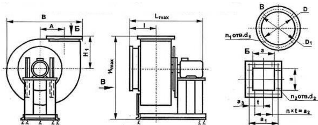
Рис. 4.6. Зовнішній вигляд вентилятора В-Ц4-70-8
