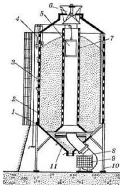
Рис. 1.5. Бункер активного вентилявання БВ-40:
