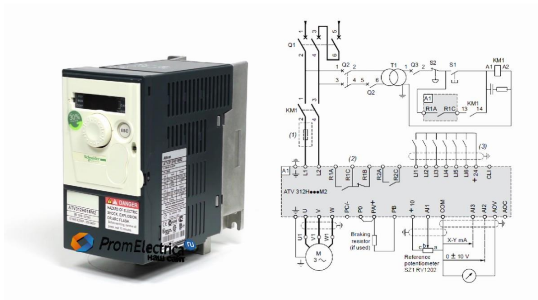
Рис. 4.9. Зовнішній вигляд перетворювача частоти Altivar ATV312 фірми Schneider Electric
