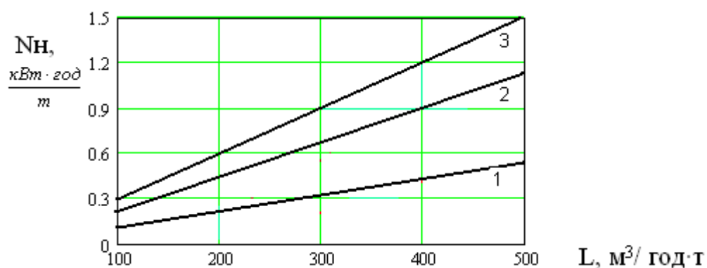
Рис. 3.10. Залежність питомої потужності калорифера від питомих витрат повітря і ступеню підігріву повітря (1 - \Delta t=3^\circ\text{C} , 2 - \Delta t=6^\circ\text{C} , 3 - \Delta t=9^\circ\text{C} )
