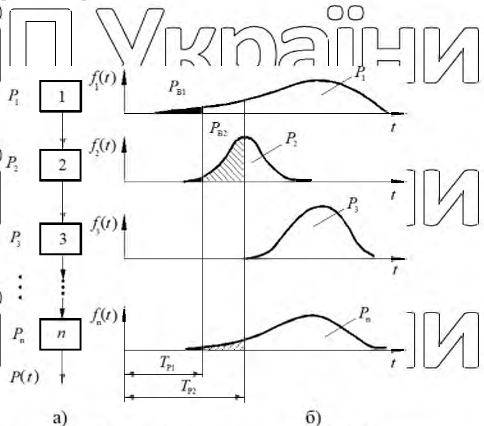
Рисунок 3.1 – Розрахункова схема послідовного з'єднання елементів складної технічної системи: а) – схема з'єднання, б) – закономірності розподілу термінів служби елементів
