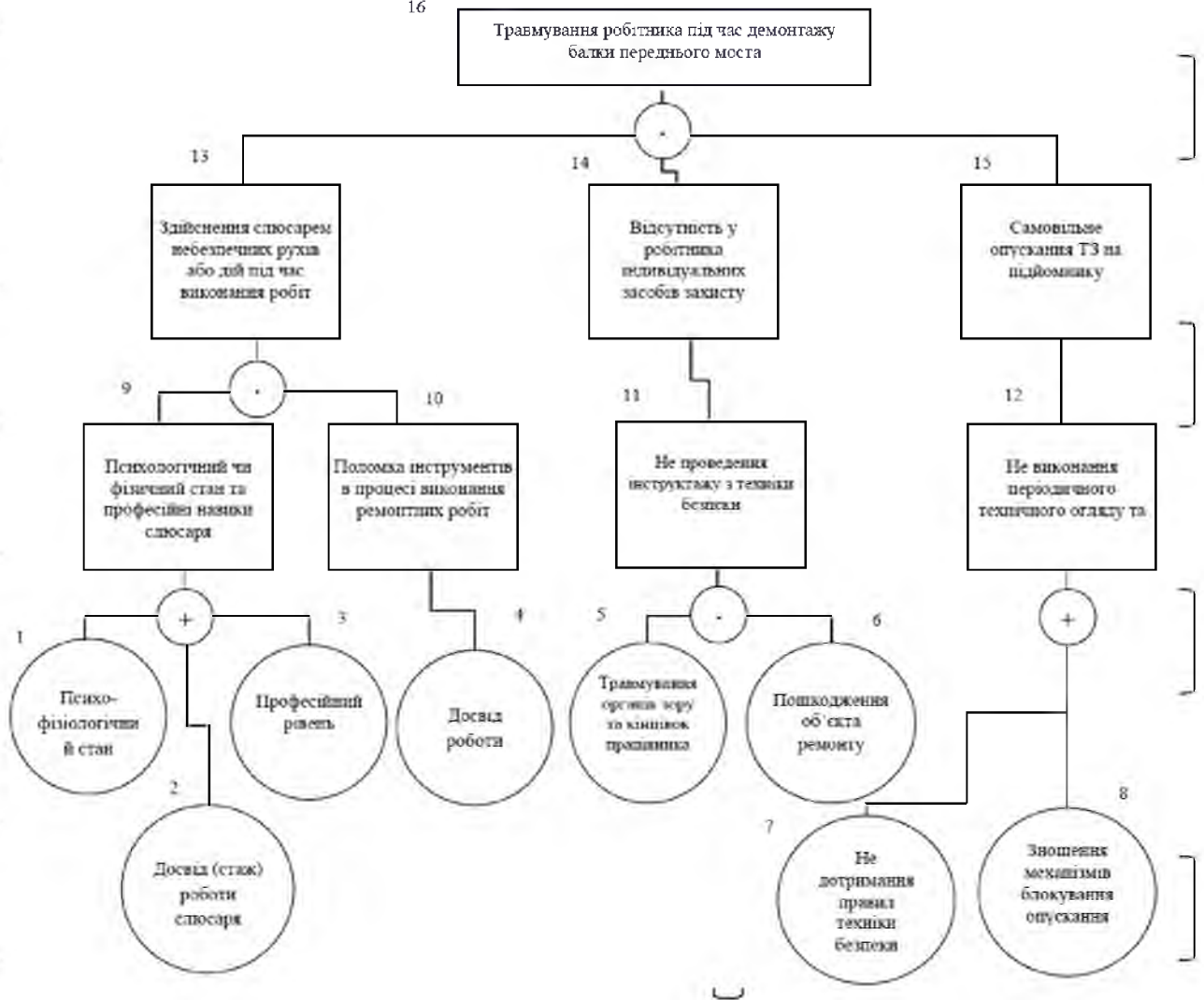
Рисунок 5.2 – Матриця логічних взаємозв’язків між окремими подіями травмо небезпечної ситуації в процесі сервісу шкільних автобусів
