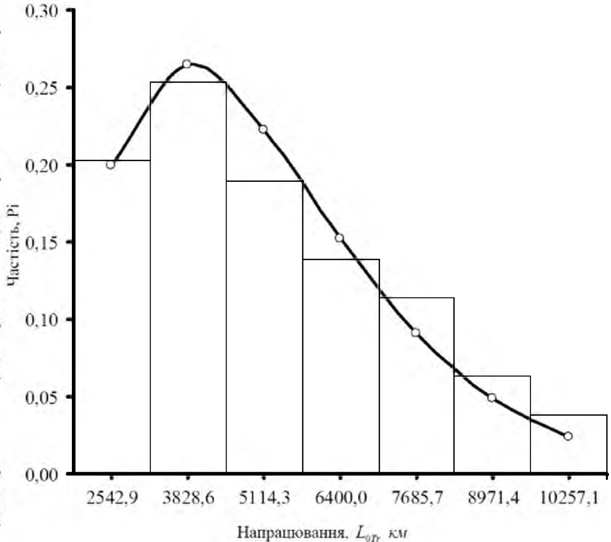
Рисунок 4.2 – Гістограма та теоретична крива розподілу середнього напрацювання на відмову автомобілів сервісної служби Volkswagen Transporter у ТОВ «Аграрний комплекс Тернопільчанка»
