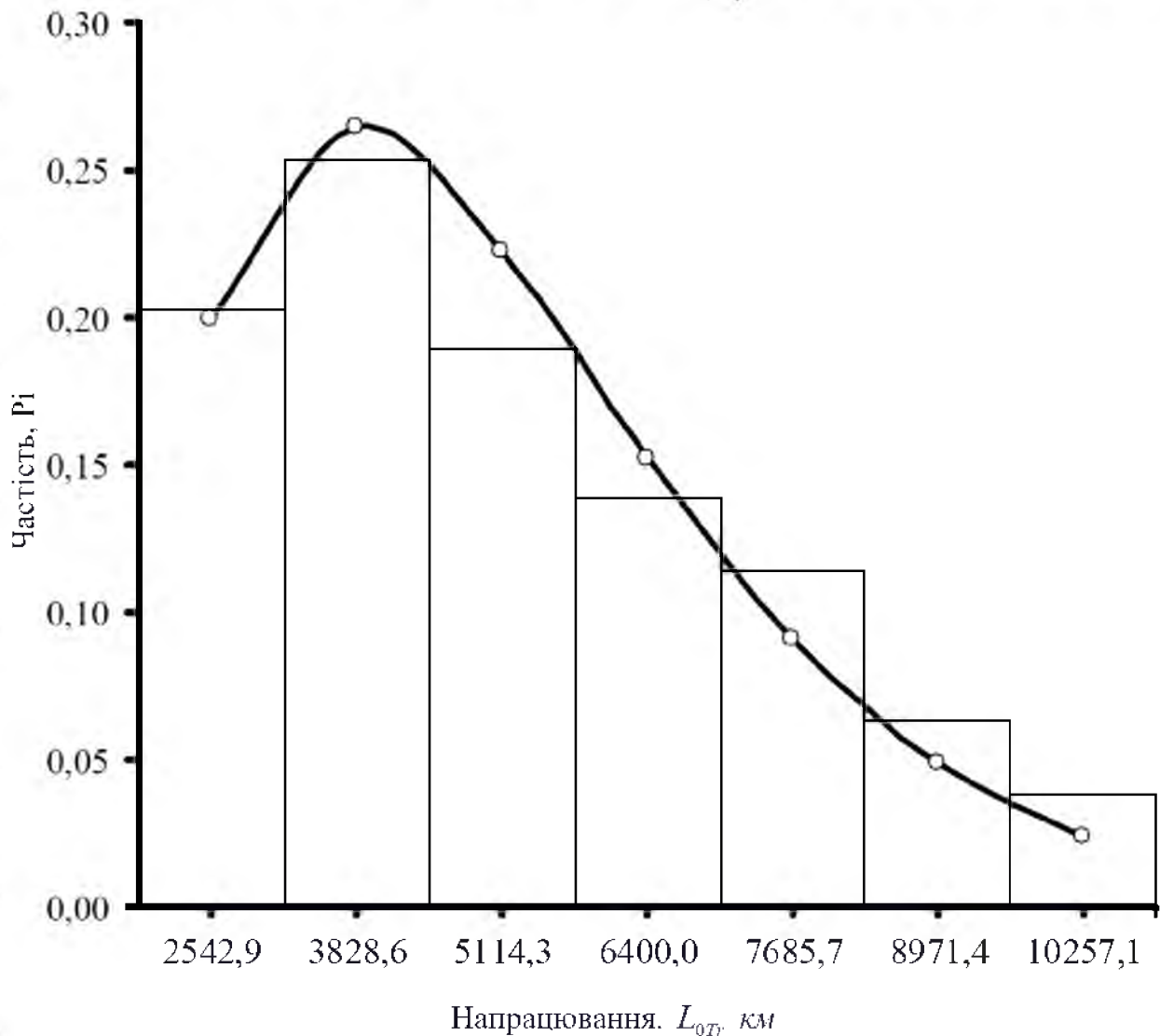
Рисунок 4.1 – Гістограма та теоретична крива розподілу середнього
