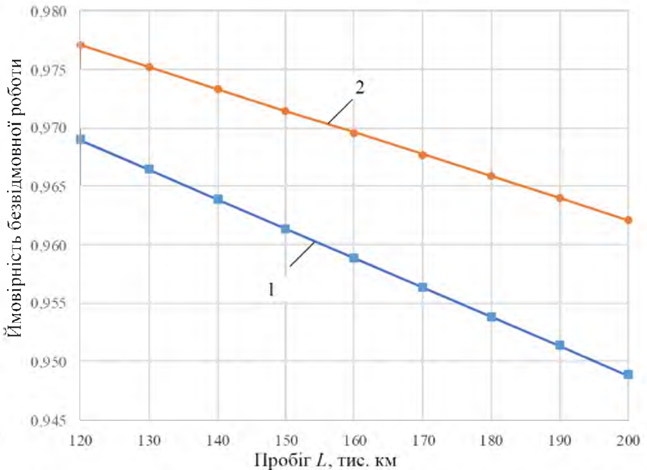
Рисунок 4.3 – Графічна інтерпретація теоретичної ймовірності
