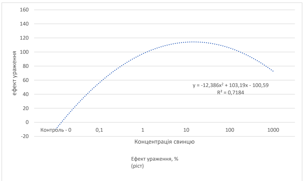
Рисунок 3.5 - Ефект пригнічення проростання насіння Lactuca sativa L внаслідок впливу свинцю
