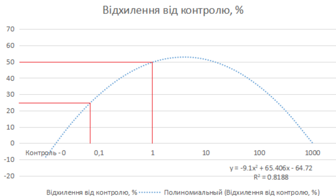
Рисунок 3.2 - Відхилення значень показників нітрифікаційної здатності від контролю
