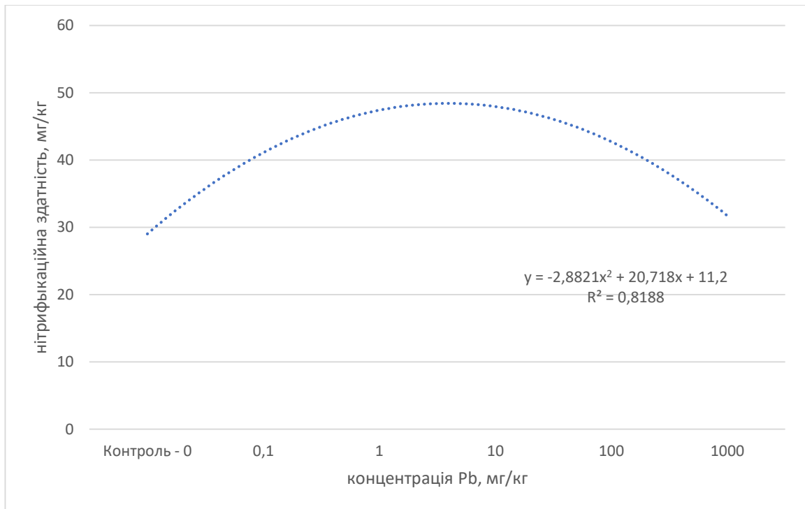
Рисунок 3.1 - Вплив свинцю на процеси мінералізації азоту у ґрунті
