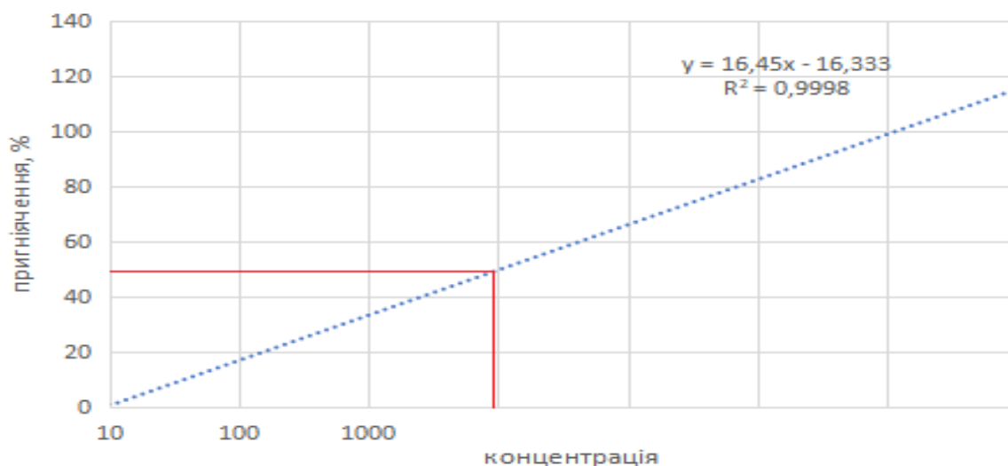
Рисунок 3.3 - Встановлення EC 50 для свинцю за активністю N-мінералізації
