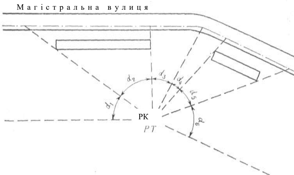
Рис. 2.21. Приклади розбивання примагістральної території забудови на ділянках з різними умовами поширення шуму.
