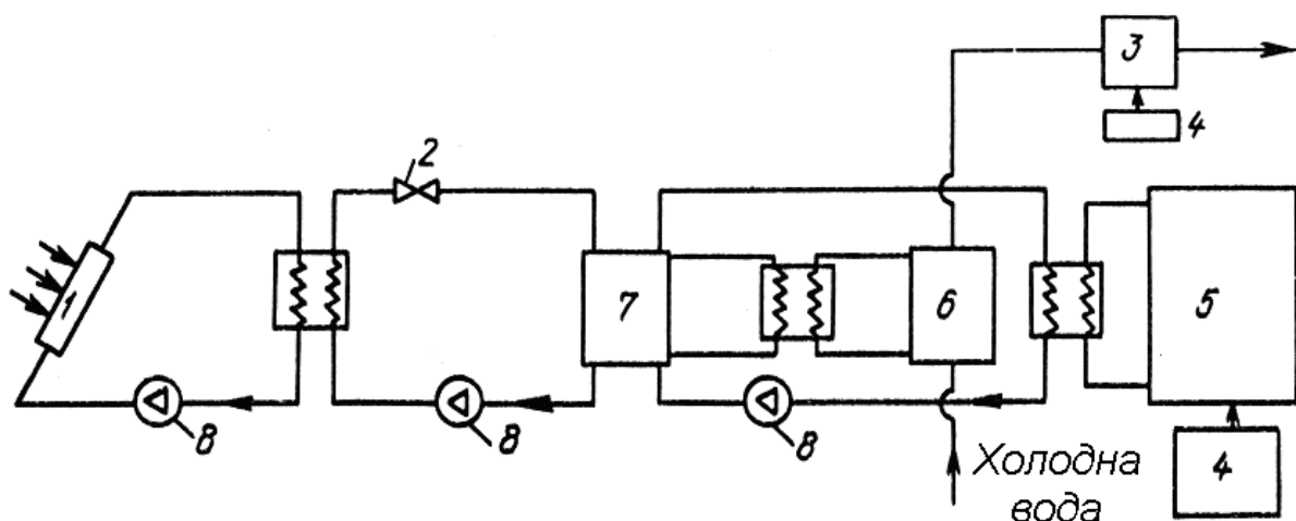
Рис. 3.33. Схема рідинної сонячно-насосної системи теплопостачання:
