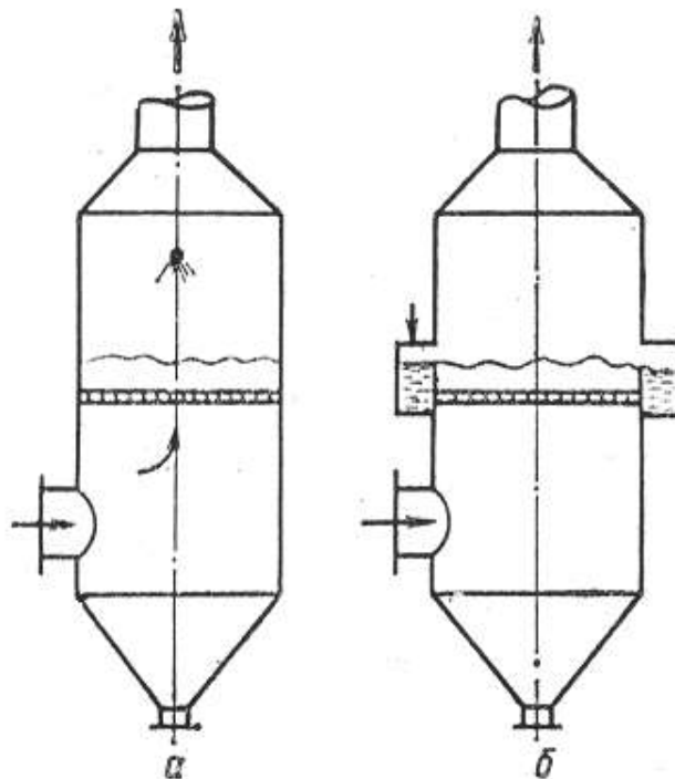
Рис. 2.10. Пінні пиловловлювачі:
