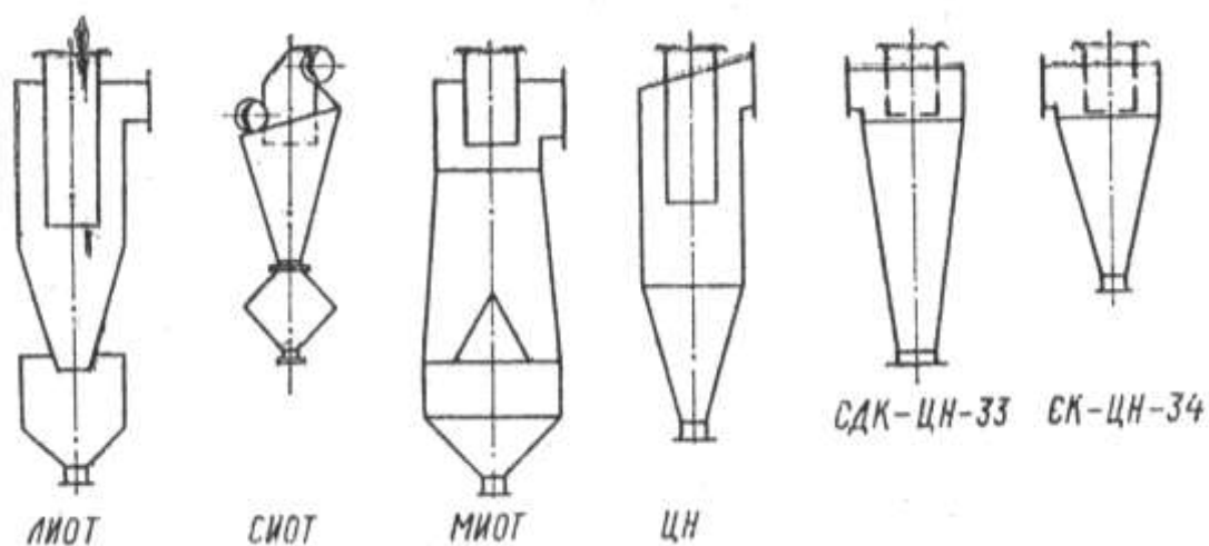
Рис. 2.4. Основні види конструкцій циклонних пиловловлювачів
