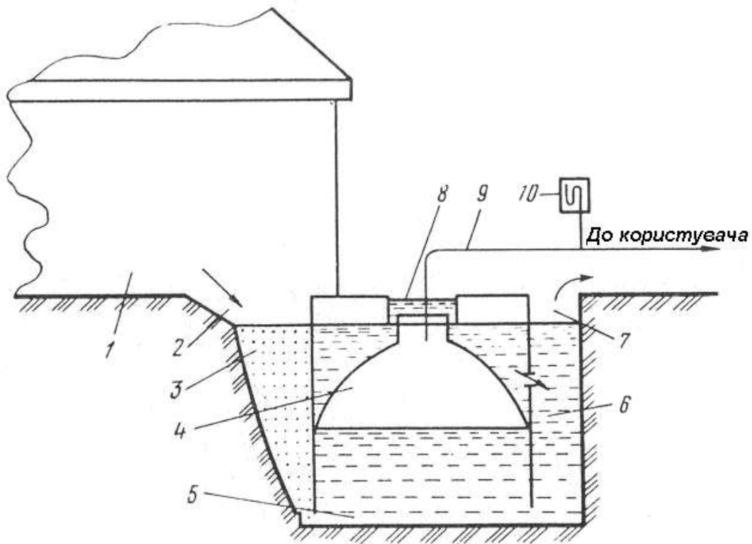
Рис. 3.10. Схема біогазової установки "Габор":
