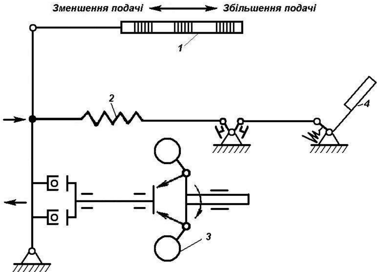
Рис. 2.37. Схема всережимного регулятора частоти обертання:
