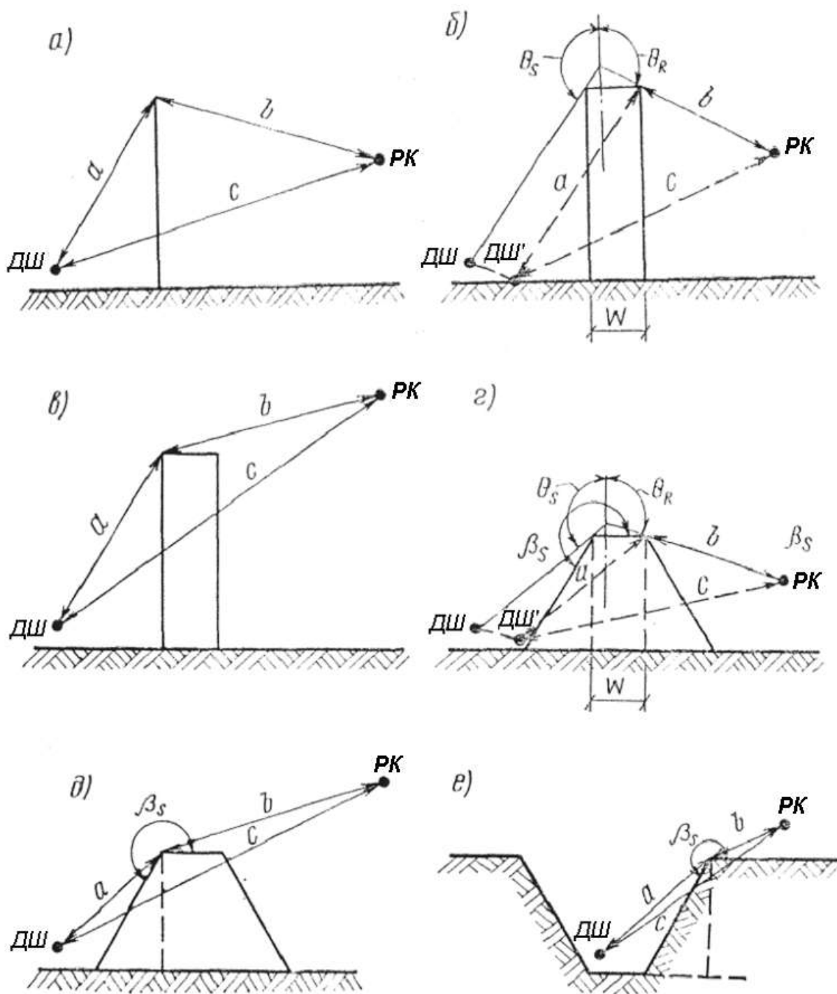
Рис. 2.27. Розрахункові схеми для визначення зниження рівнів шуму екранами.
