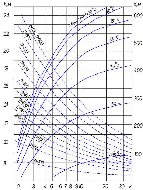
Рис. 3.44. Номограма для визначення величини K і h – втрат тиску в діафрагмі за заданими d , D і T_n
