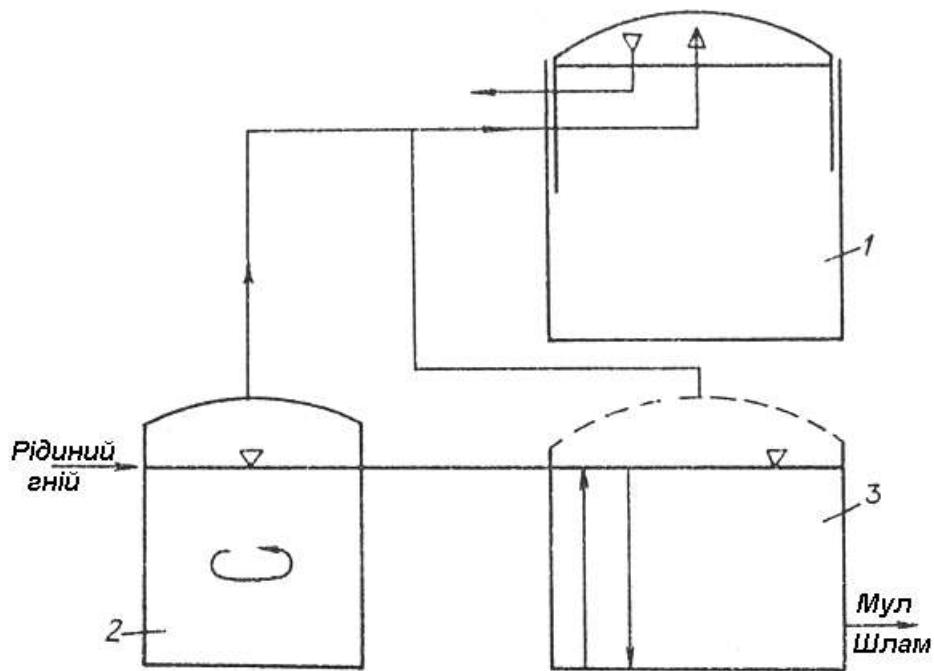
Рис. 3.3. Схема безперервного зброджування: 1 – газгольдер; 2 – реактор; 3 – сховище мулу (шламу)
