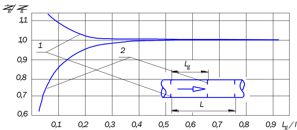
Рис.3.46. Графік залежності коефіцієнтів опору діафрагми \zeta_g і \zeta'_g від відстані між ними L_g за умови, що 0 < L_g < L
