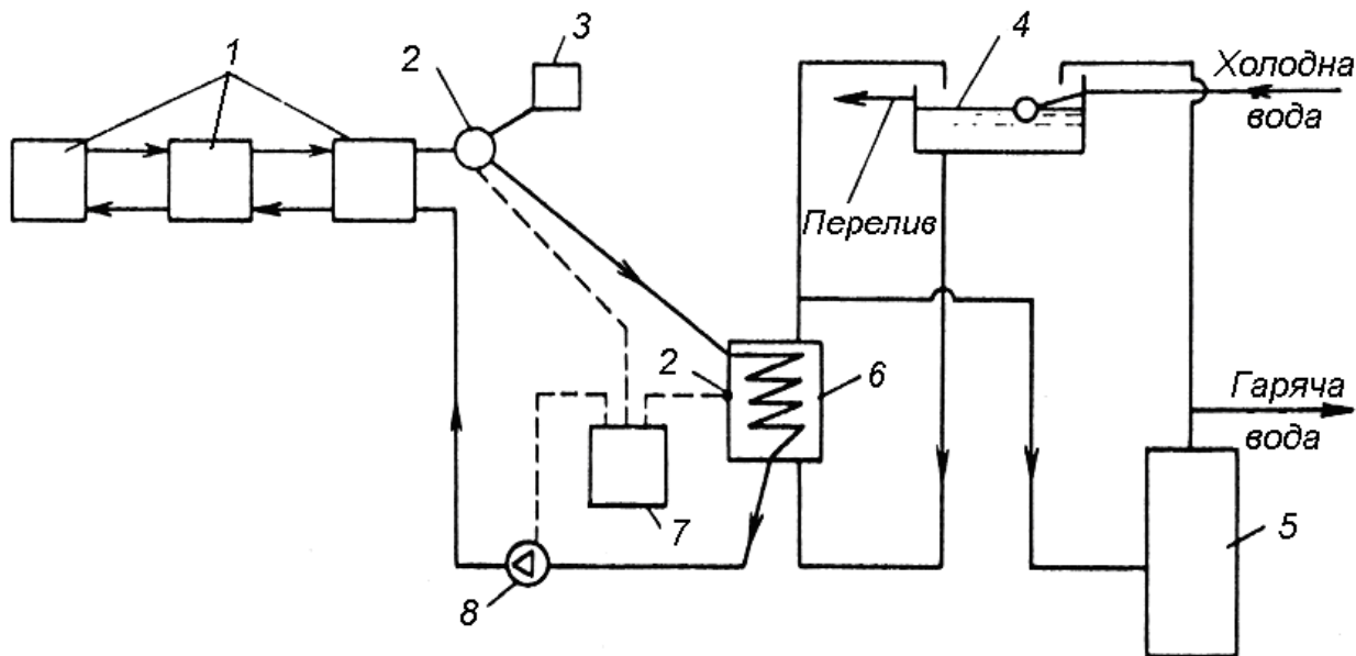
Рис. 3.37. Система гарячого водопостачання з примусовою циркуляцією:
