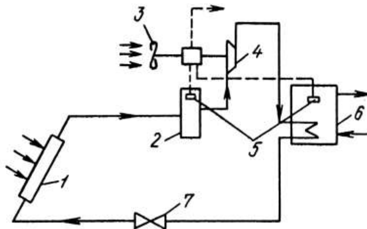
Рис. 3.28. Схема геліовітротеплонасосної установки
