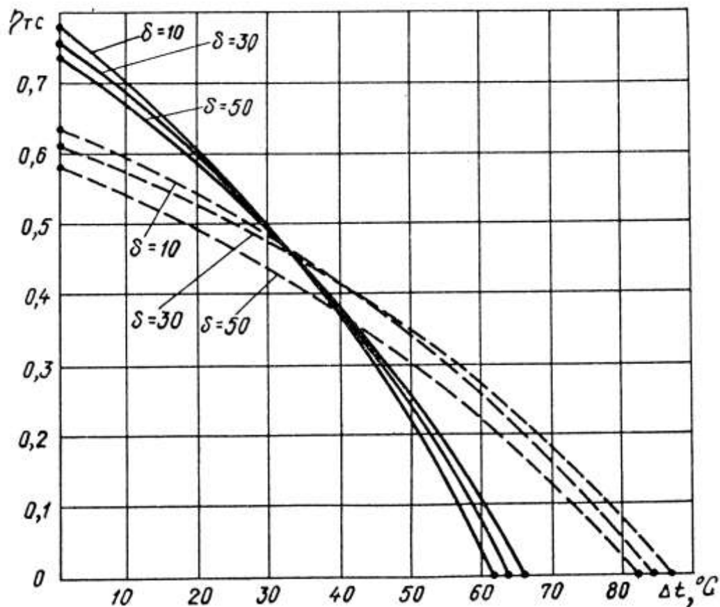
Рис. 3.21. Залежність теплового ККД заскління від різниці температур між поверхнею нагрівання і довколишнім повітрям при: — — одному листі скла; — — — — двох листах скла
