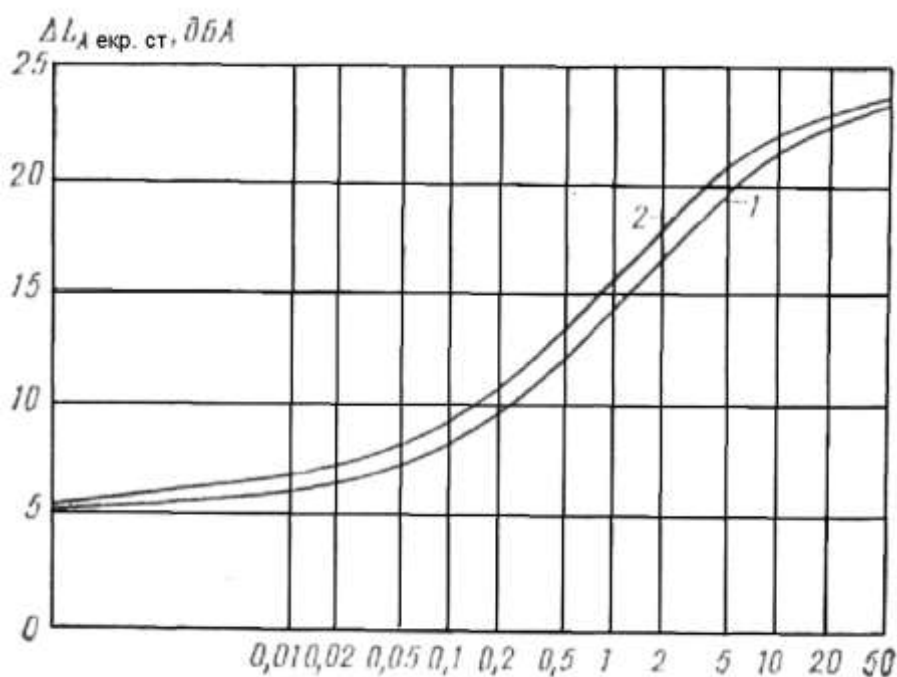
Рис. 2.26. Графіки для визначення зниження рівня шуму екраном-стіною
