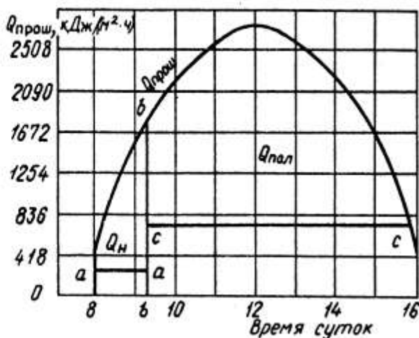
Рис. 3.24. Схема для визначення корисної поверхні нагрівання для M = 50 л/год
