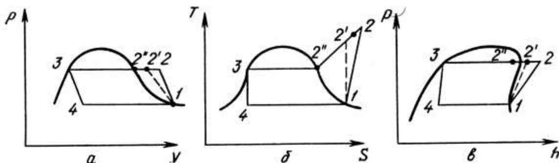
Рис. 3.30. Реальний коловий цикл теплового насоса у діаграмах: а – p-v ; б – T-S ; в – p-h
