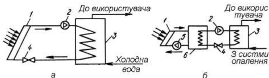
Рис. 3.34. Схеми теплових насосів, що використовують сонячне нагрівання: а – прямий; б – непрямий; 1 – колектор; 2 – компресор; 3 – конденсатор; 4 – редукційний клапан; 5 – насос; 6 – випарник
