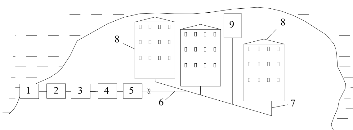
Рис.2.7. Схема традиційної системи водопостачання
