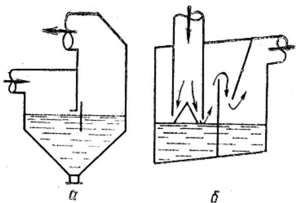
Рис. 2.13. Абсорбційні уловлювачі ударно-інерційного типу; а – типу ПВМ; б – скрубер Дойля
