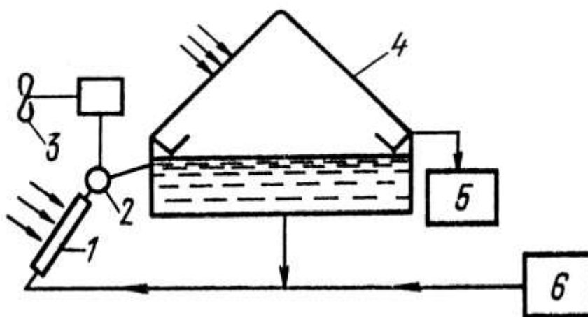
Рис. 3.25. Схема геліовітротеплової опріснювальної установки
