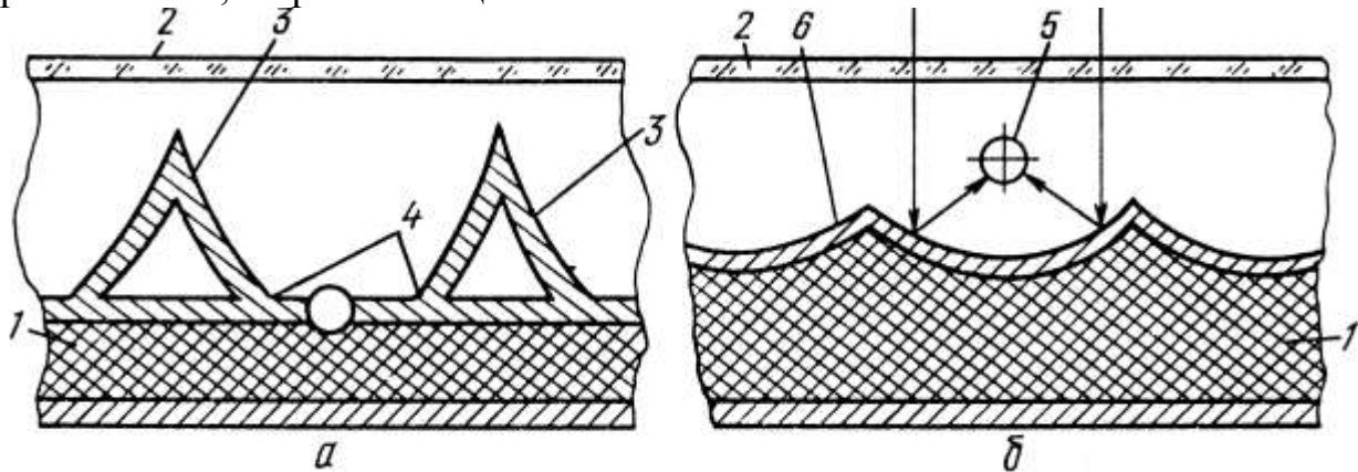
Рис. 3.16. Концентрувальний колектор:
