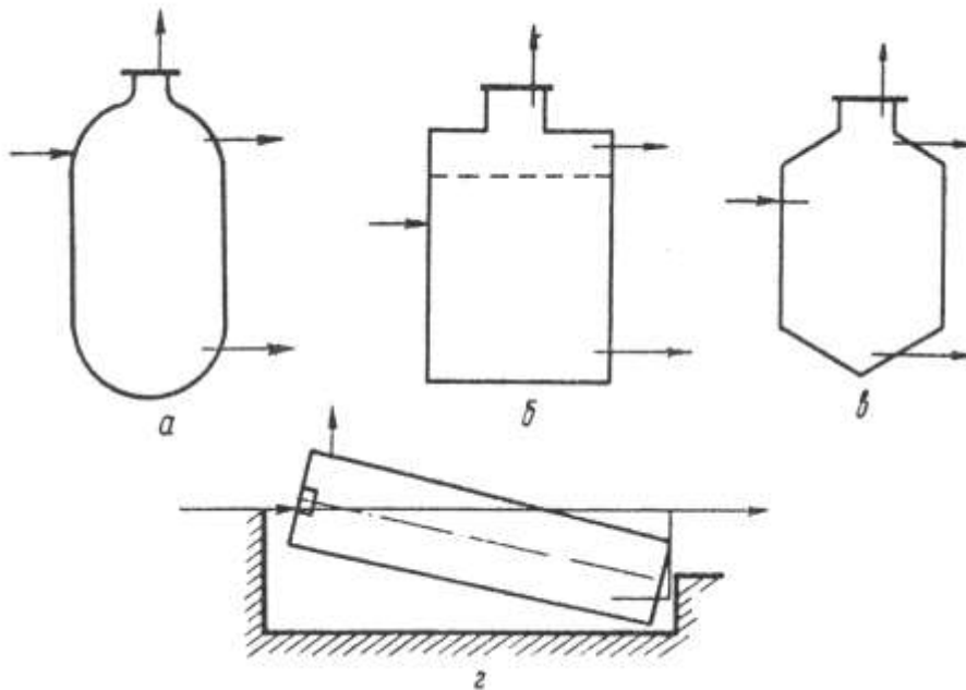
Рис. 3.6. Форми камер зброджування: а – овальна; б – циліндрова; в – циліндрово-конічна; г – похило-горизонтальна
