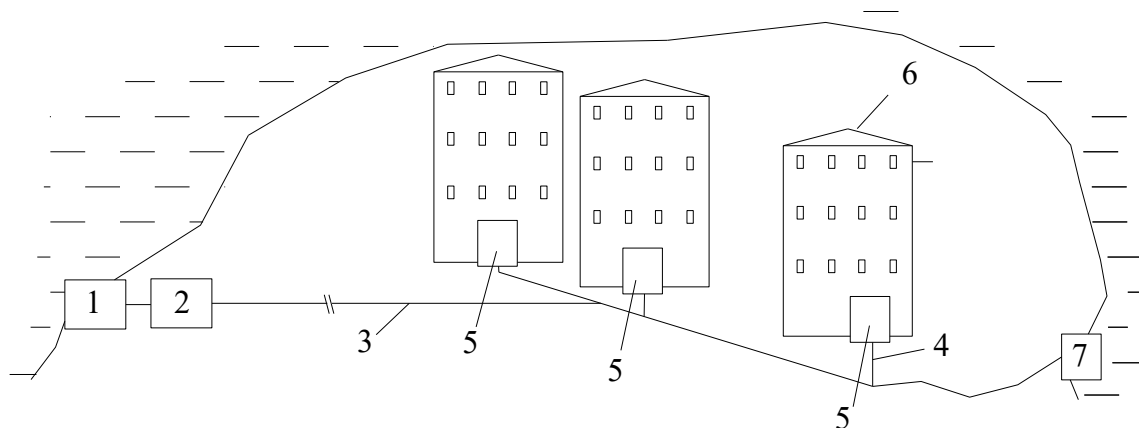
Рис.2.8. Схема удосконаленої системи водопостачання
