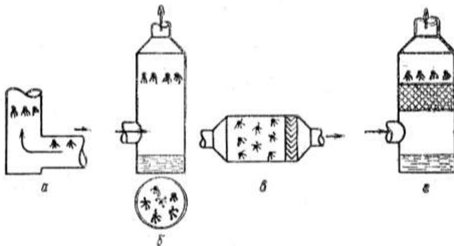
Рис. 2.8. Абсорбційні пристрої для очищення газів:
