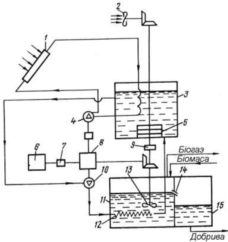
Рис. 3.27. Схема геліовітроенергетичної метаногенерувальної установки
