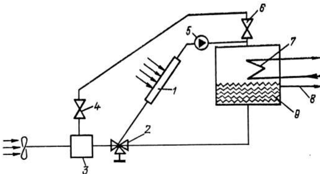
Рис. 3.26. Схема геліовітропелової установки:
