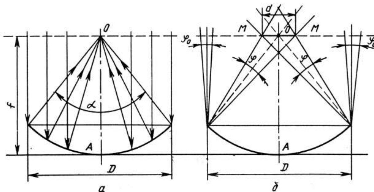
Рис. 3.15. Концентрація променів після відбиття від дзеркала параболоїда: а – паралельних; б – непаралельних
