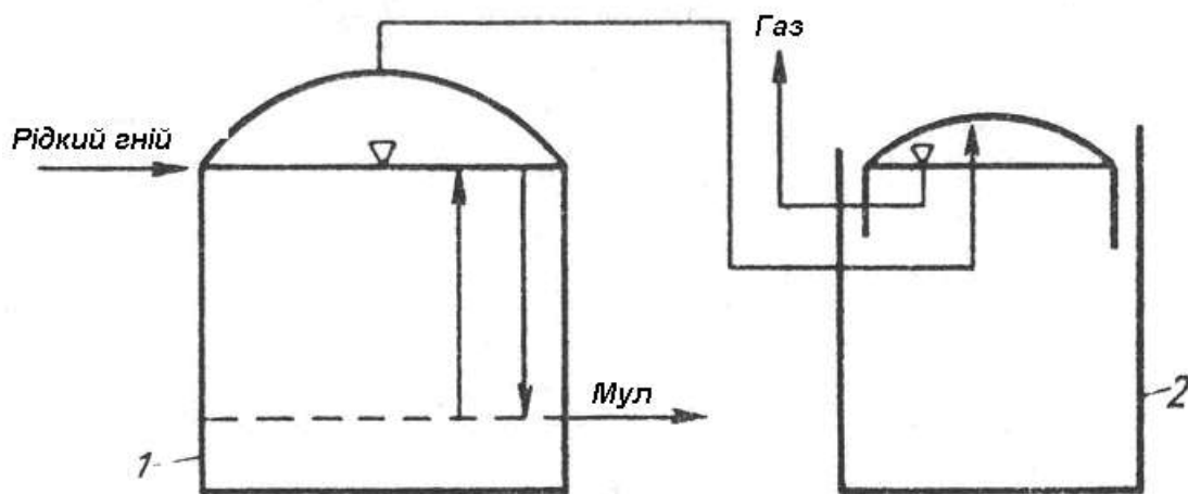
Рис. 3.5. Схема аккумулятивного зброджування:
