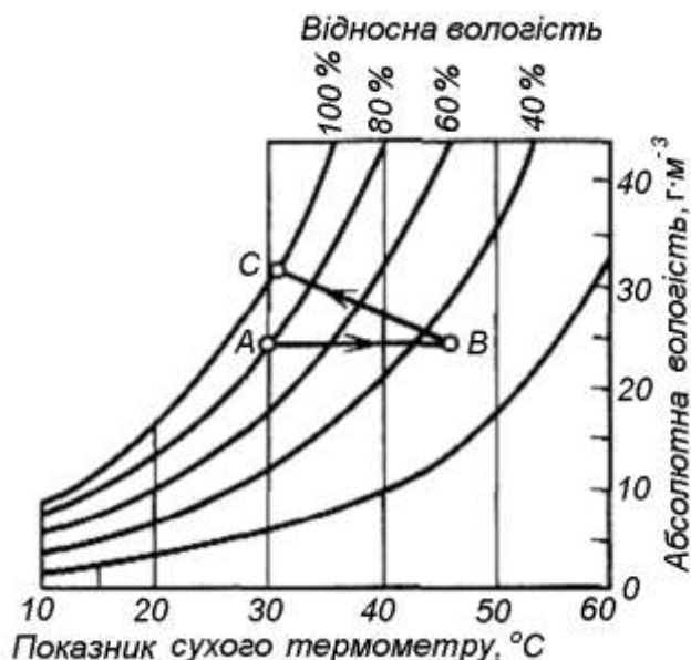
Рис. 3.38. Психрометрична діаграма (для стандартного тиску 101,3 кПа)
