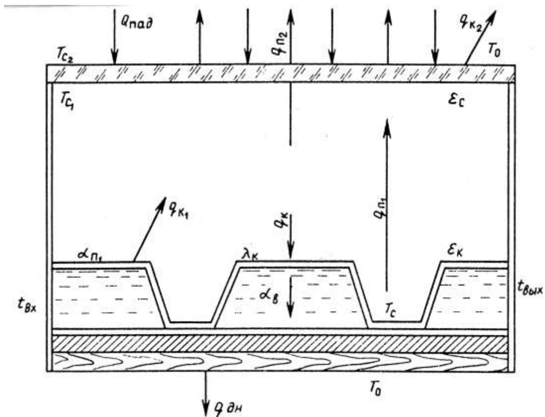
Рис. 3.18. Схема теплових потоків колектора
