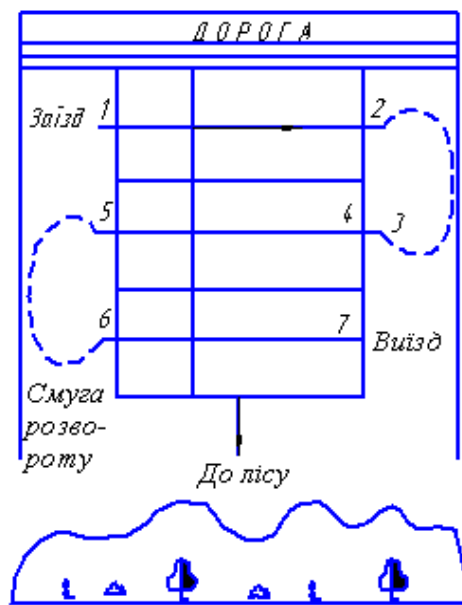
Рис. 5.3 Човниковий спосіб руху агрегату
