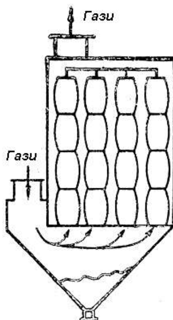
Рис. 2.7. Рукавний фільтр
