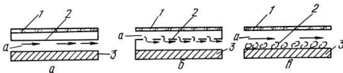
Рис.3.14. Повітронагрівач: а – з плоским листовим теплоприймачем; б – з перфорованим теплоприймачем; в – із стружковим теплоприймачем
