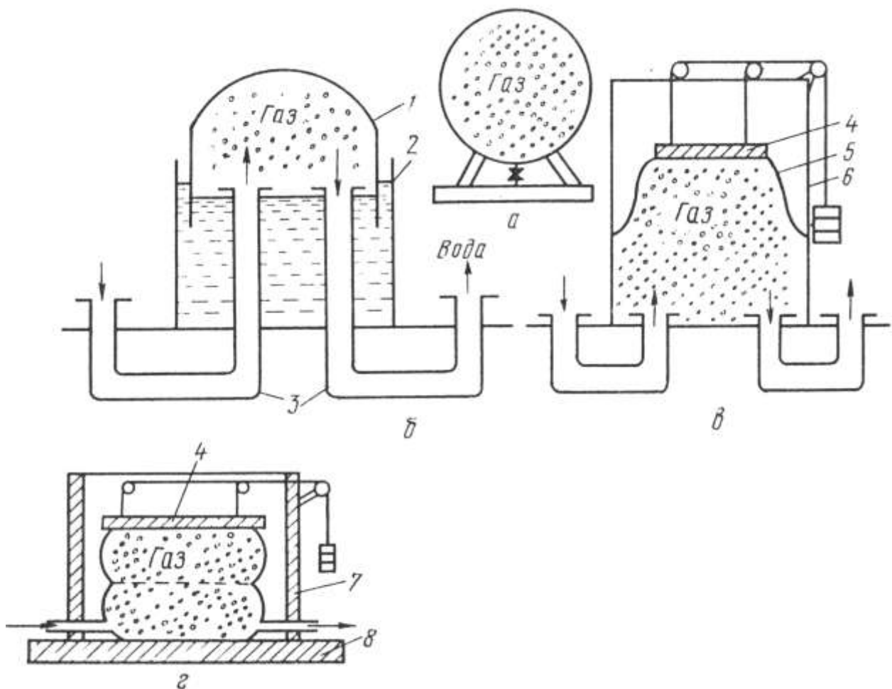
Рис. 3.9. Схеми газгольдерів: а – сферичні високого тиску; б – мокрі однопіднімні низького тиску; в – сухі низького тиску манжетного типу; г – оболонкові низького тиску; 1 – дзвін; 2 – вмістище; 3 – газопровід; 4 – вантаж; 5 – манжета; 6 – резервуар; 7 – кожух; 8 – плита
