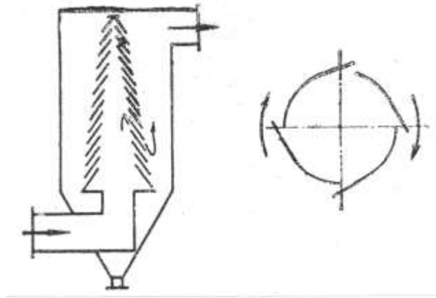
Рис. 2.2. Жалюзійний пиловловлювач
