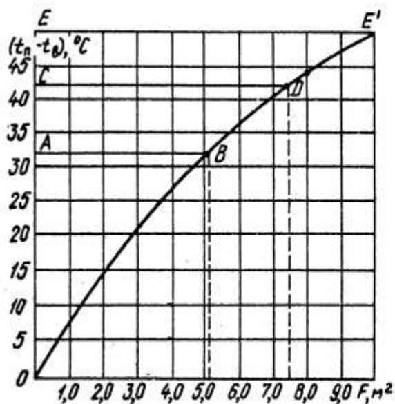
Рис. 3.23. Вплив різниці температур на площу скла стандартної секції колектора
