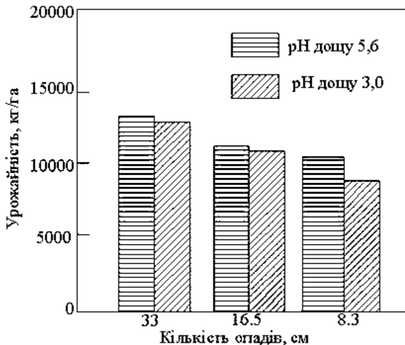
Рис. 2.17. Вплив кислих дощів на урожайність кукурудзи залежно від кількості опадів (за Заїковим та ін., 1991 р.)
