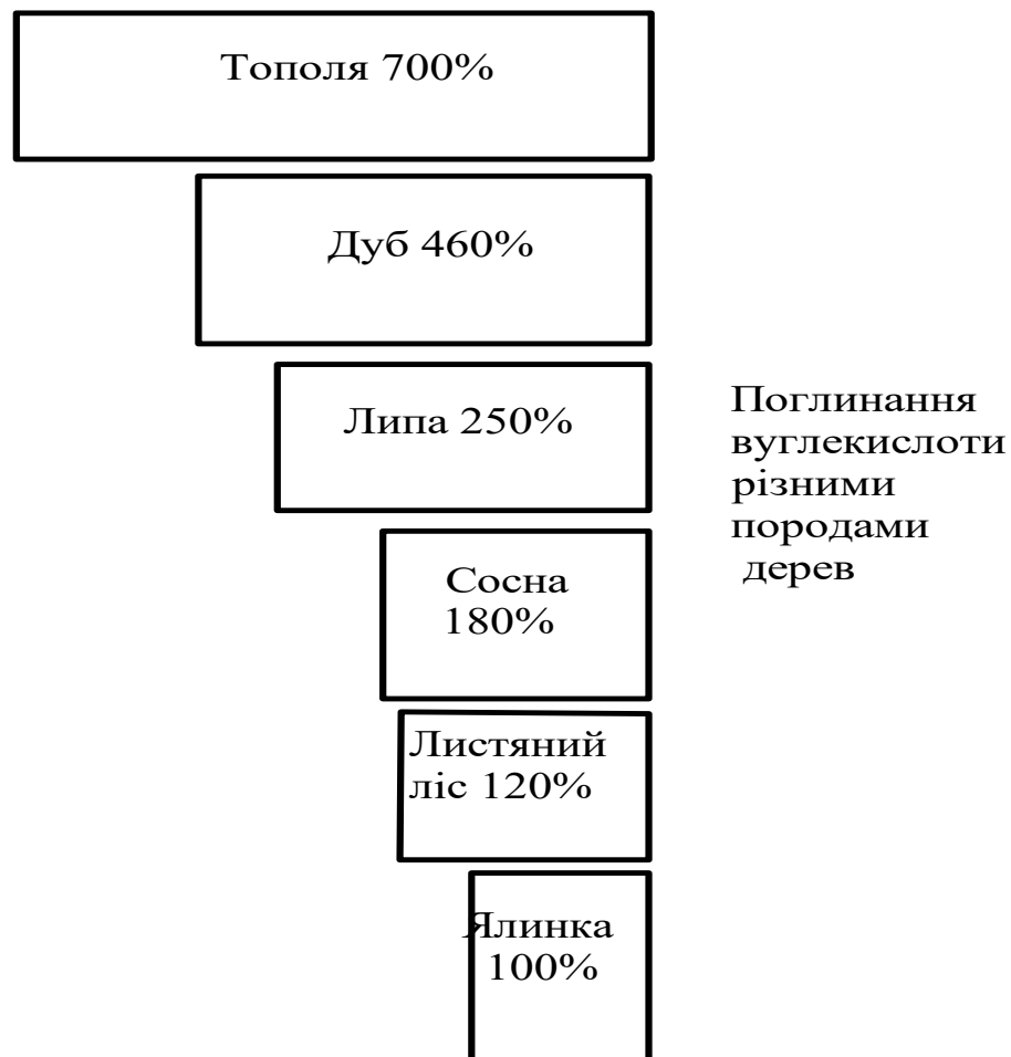
Рис. 2.18. Поглинання вуглекислоти різними породами дерев
