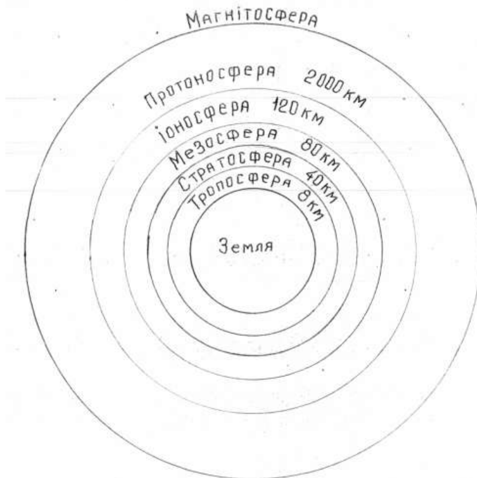
Рис. 2.15. Будова атмосфери
