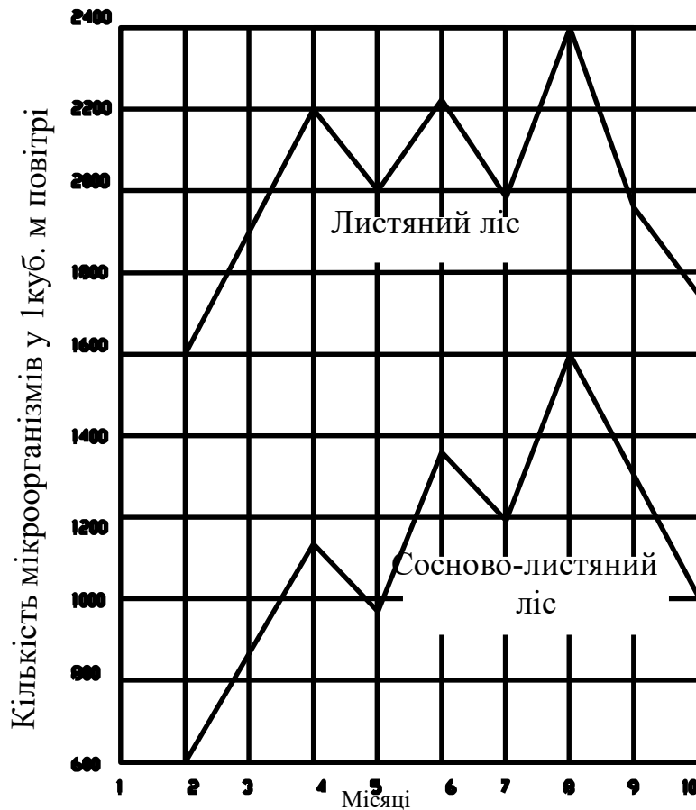
Рис. 1.3. Загальна бактерійна забрудненість повітря в міських лісах м. Києва
