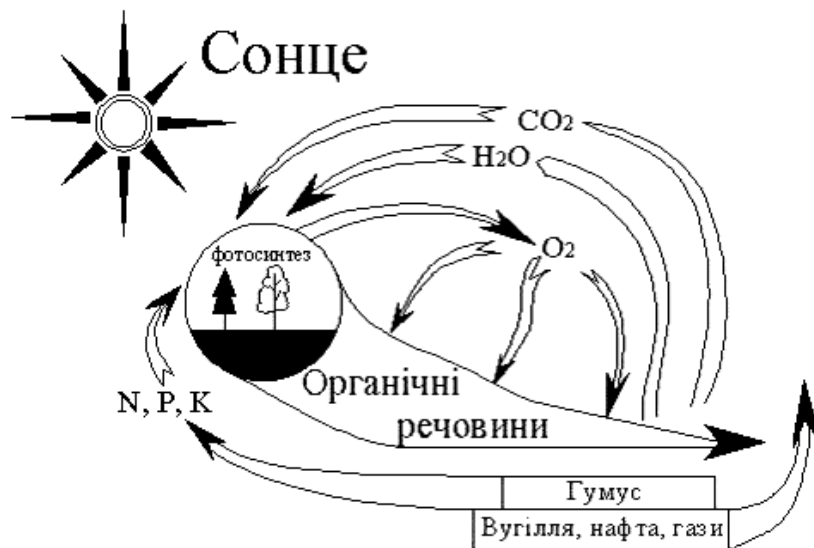
Рис. 1.11. Біологічний кругообіг речовин в екосистемах
