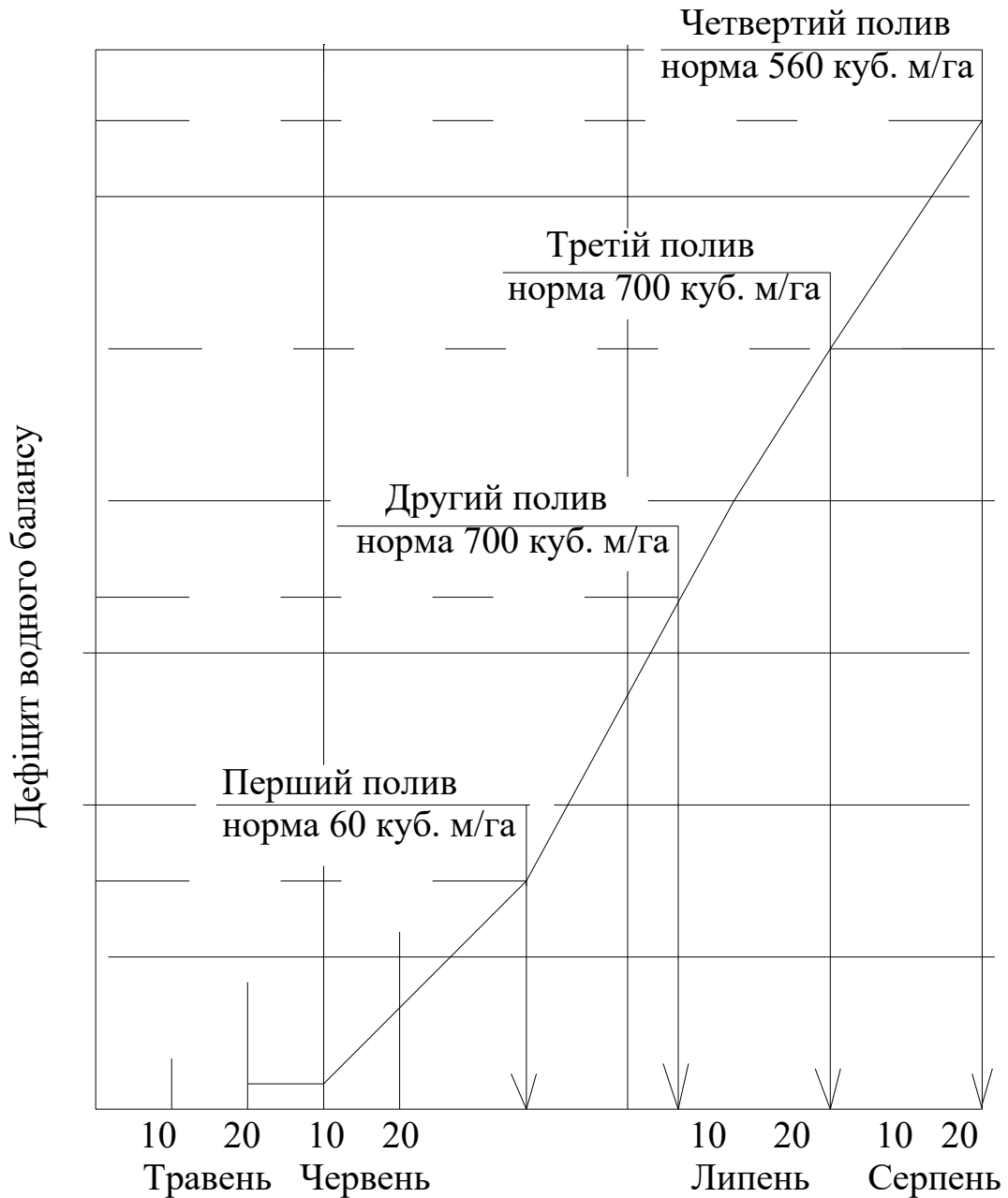
Рис. 1.4. Інтегральна крива дефіциту водного балансу поля, зайнятого під кукурудзу, в період оптимального водозабезпечення
