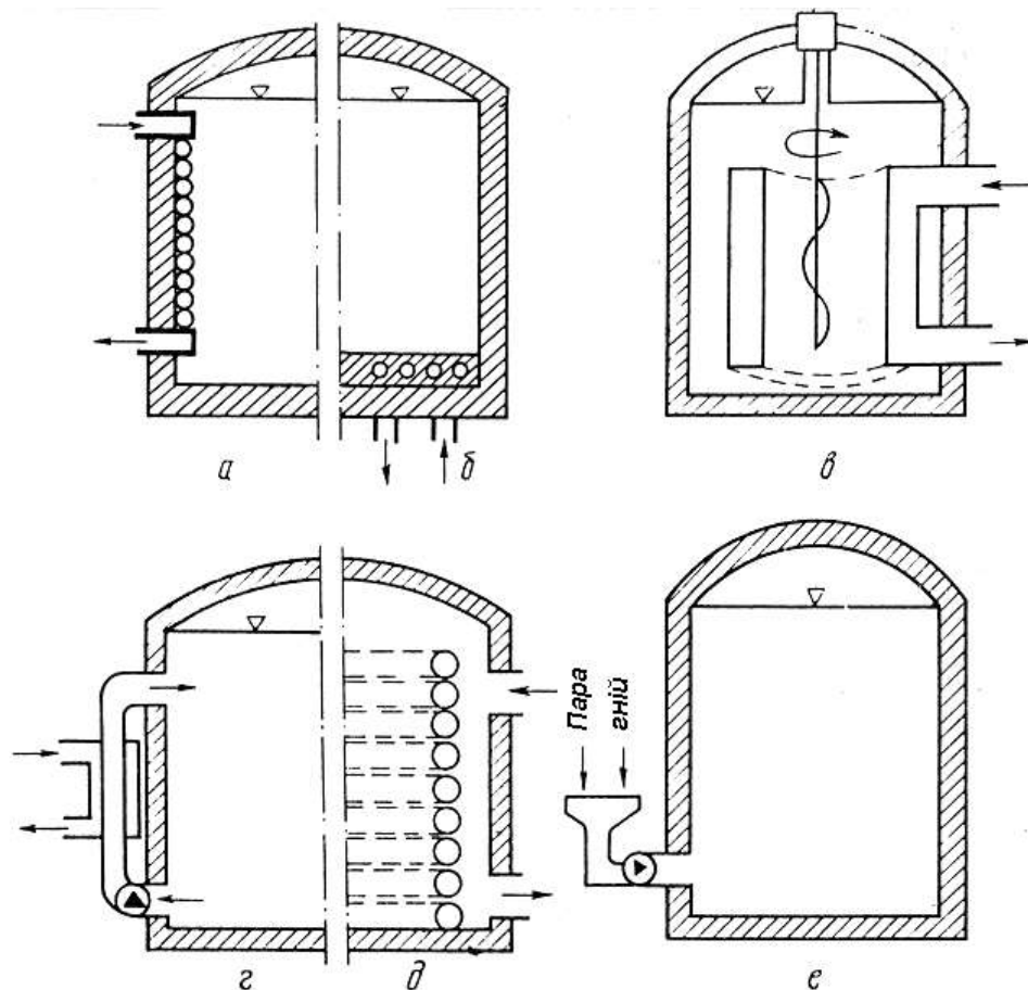
Рис. 3.7. Схеми нагрівальних пристроїв:
