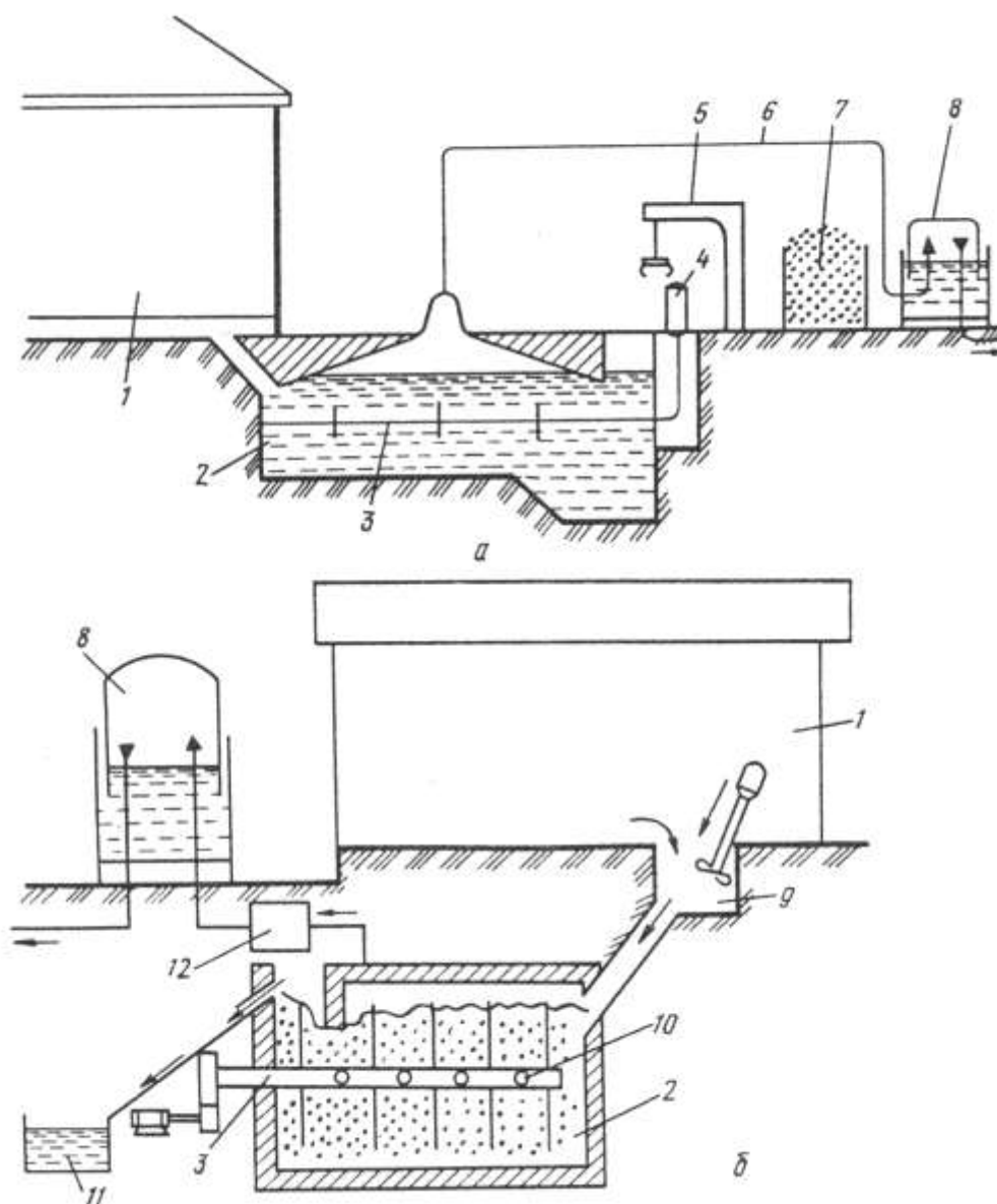
Рис. 3.11. Схема біогазової установки "Дормштадт":
