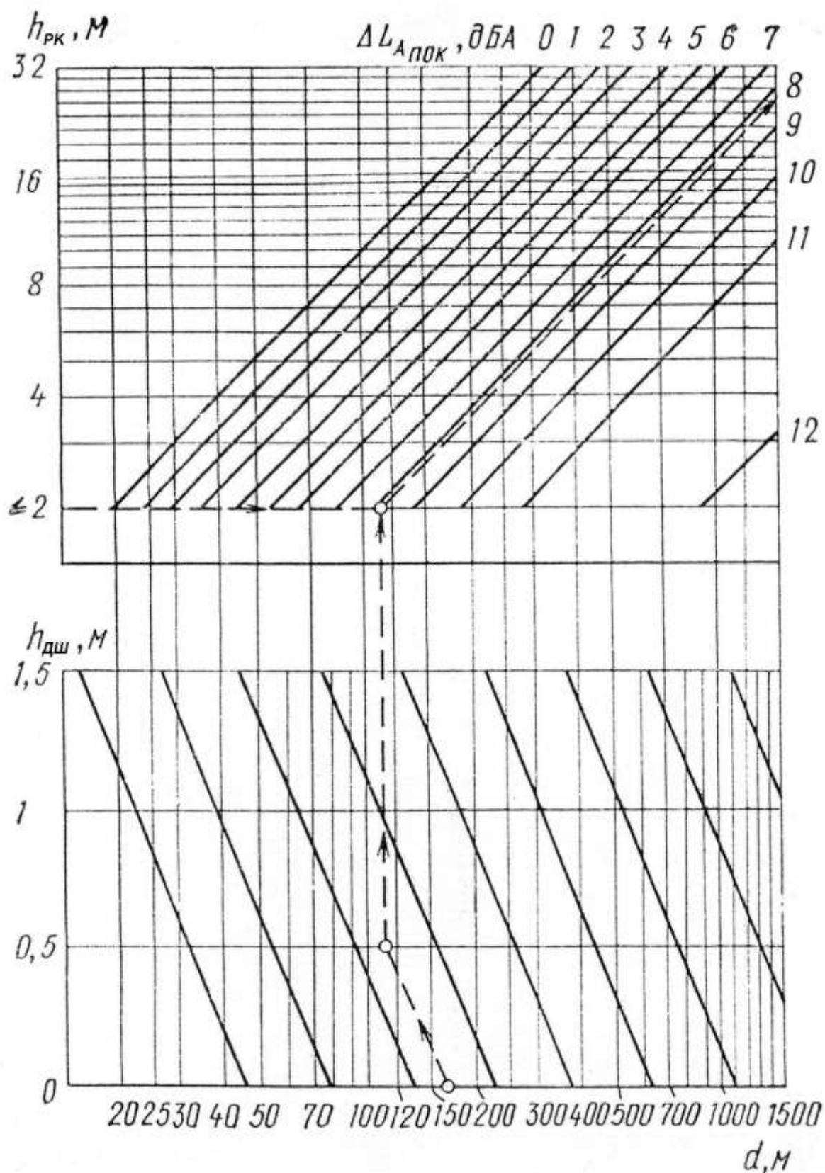
Рис. 2.24. Номограма для визначення зниження рівня шуму внаслідок його поглинання акустично-м'яким покривом території за умови вільного поширення шуму
