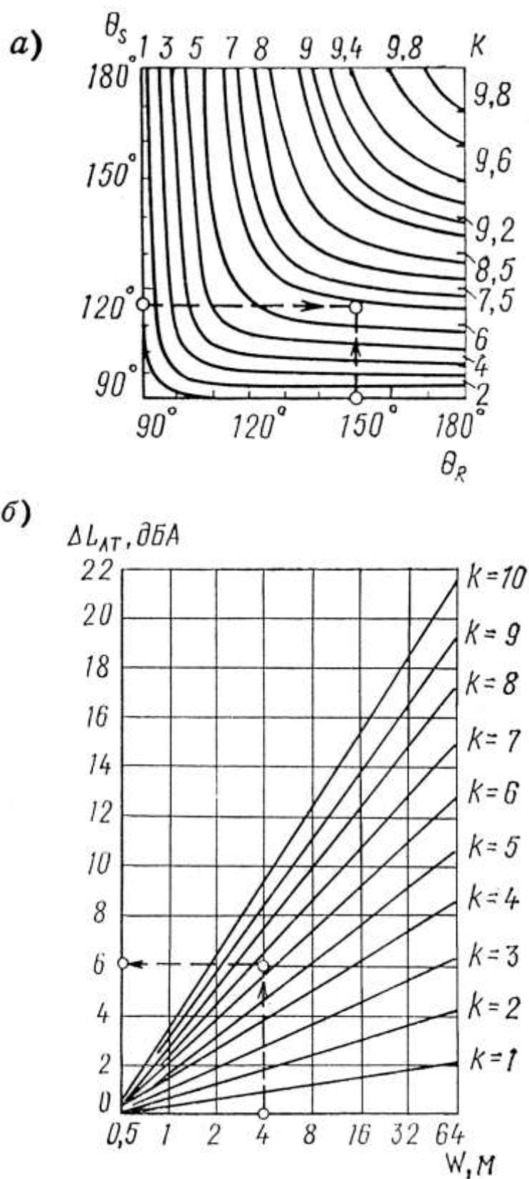
Рис. 2.28. Номограма для визначення додаткового зниження рівня шуму екраном більшої товщини.
