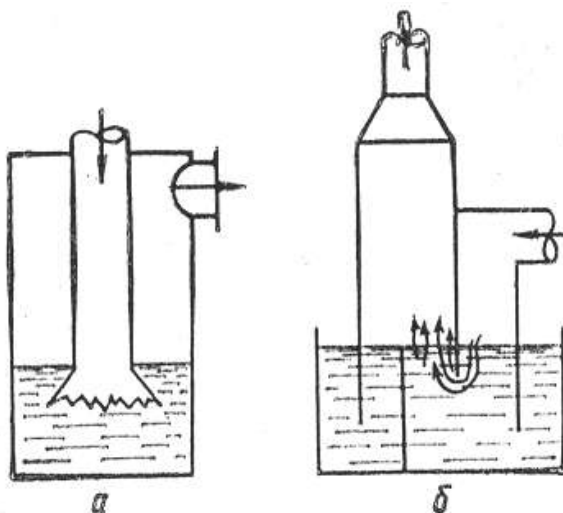
Рис. 2.9. Барботажні апарати для очищення газів: а – прямої дії; б – з відокремлюваною перегородкою
