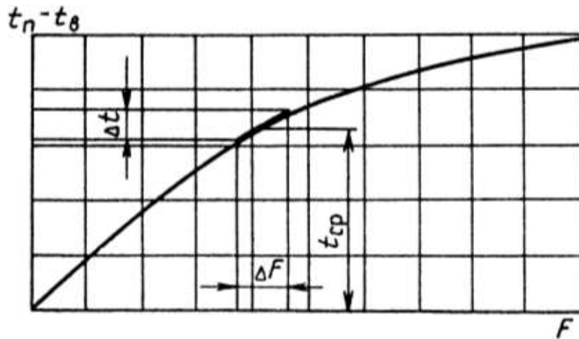
Рис. 3.22. Схема для визначення пропорцій між одинарним і подвійним засклінням колектора
