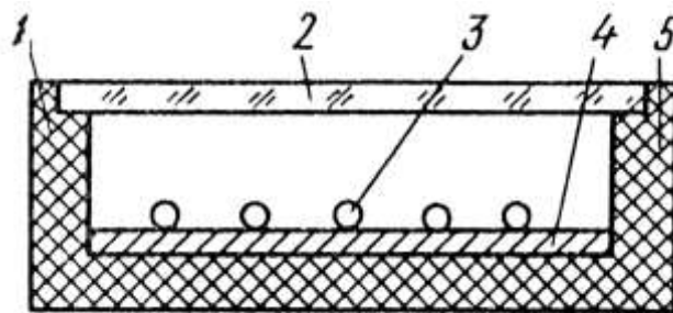
Рис. 3.12. Плоский сонячний колектор з рідинним теплоносієм
