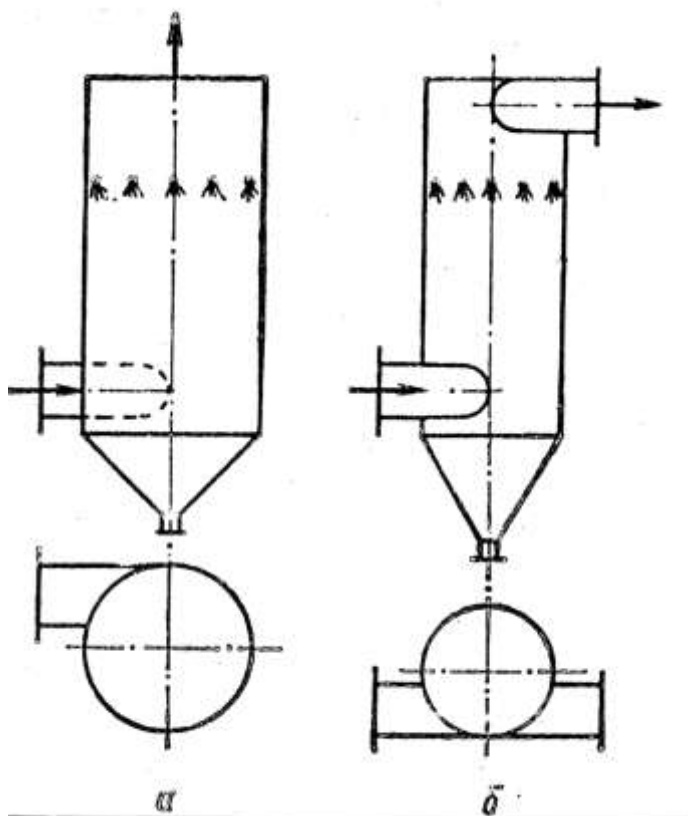
Рис. 2.14. Відцентрові скрубєри: а – типу ВТІ; б – типу ЛПОТ
