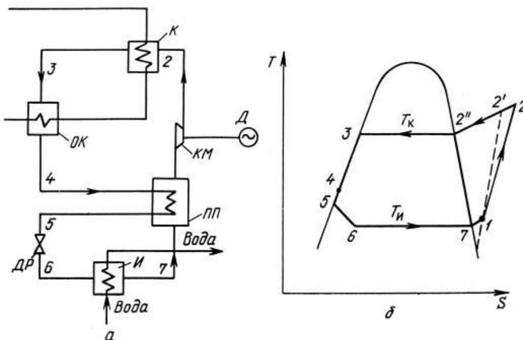
Рис. 3.32. Теплонасосна установка:
