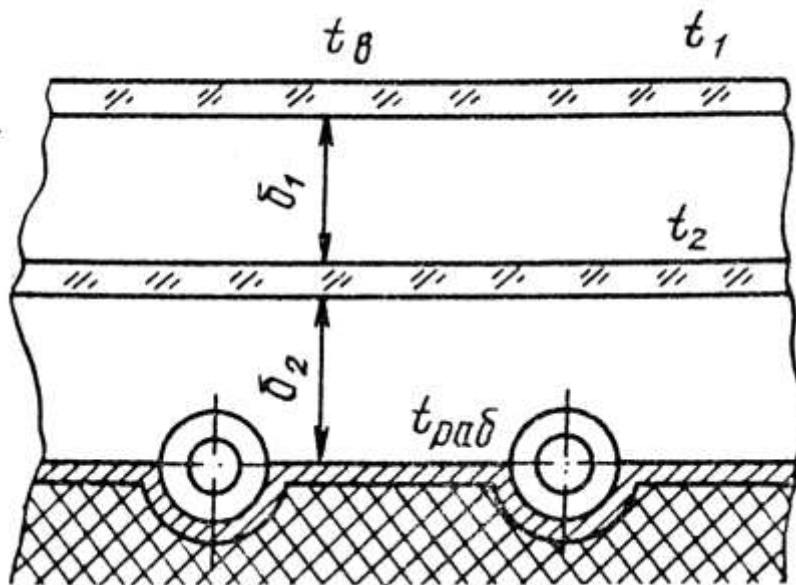
Рис. 3.19. Схема подвійного застління колектора
