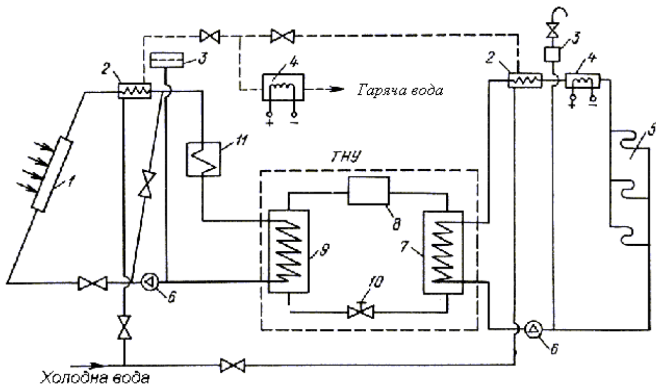
Рис. 3.35. Принципова схема триконтурної сонячно-насосної системи теплопостачання житлового будинку:
