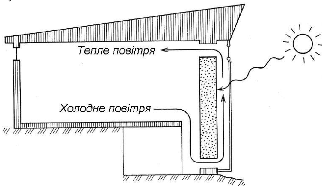
Рис. 3.40. Принцип дії накопичувальної стіни будинку взимку
