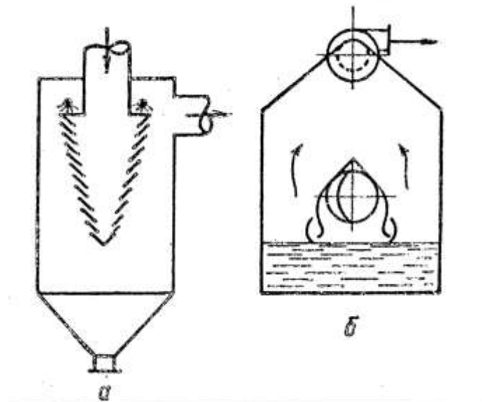
Рис. 2.11. Пиловловлювачі ударно-інерційного типу: а – типу УСД-ЛІОТ; б – ротоклон
