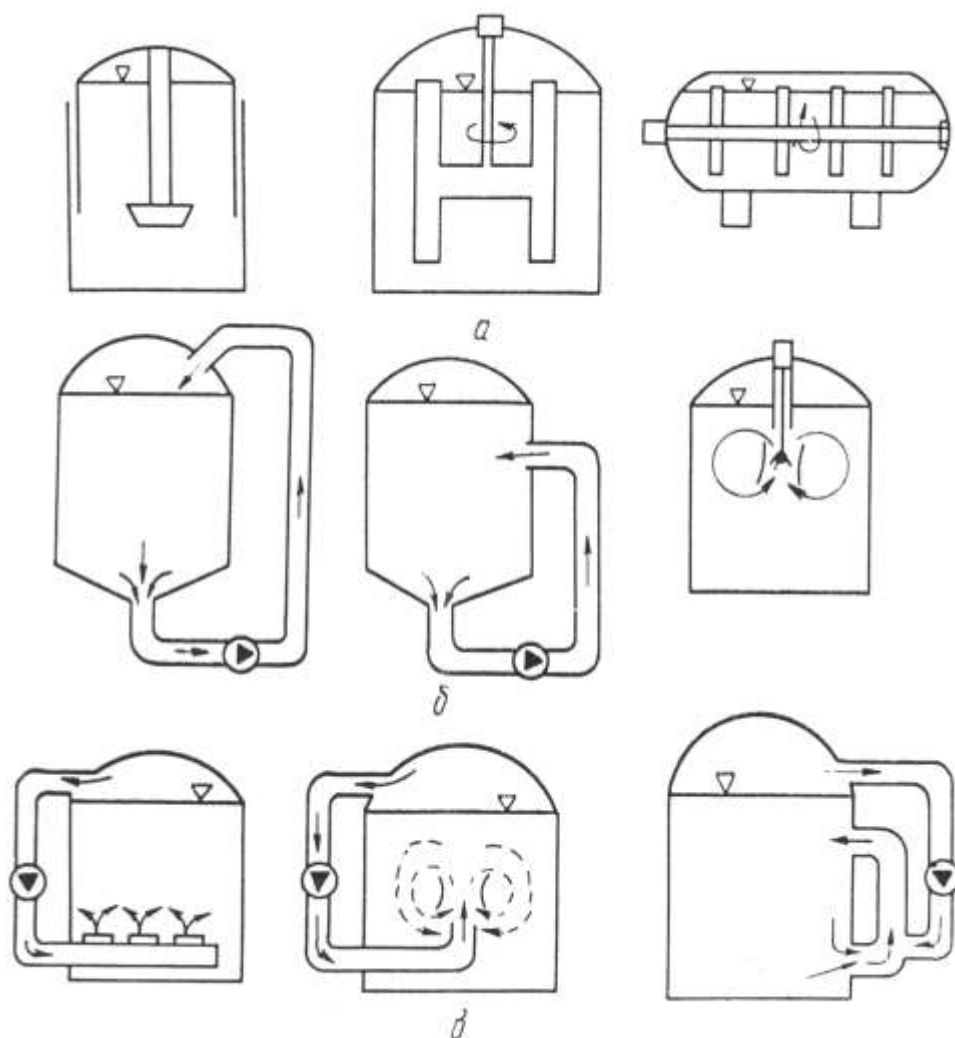
Рис. 3.8. Схеми пристроїв для перемішування: а – механічні; б – гідравлічні; в – газові
