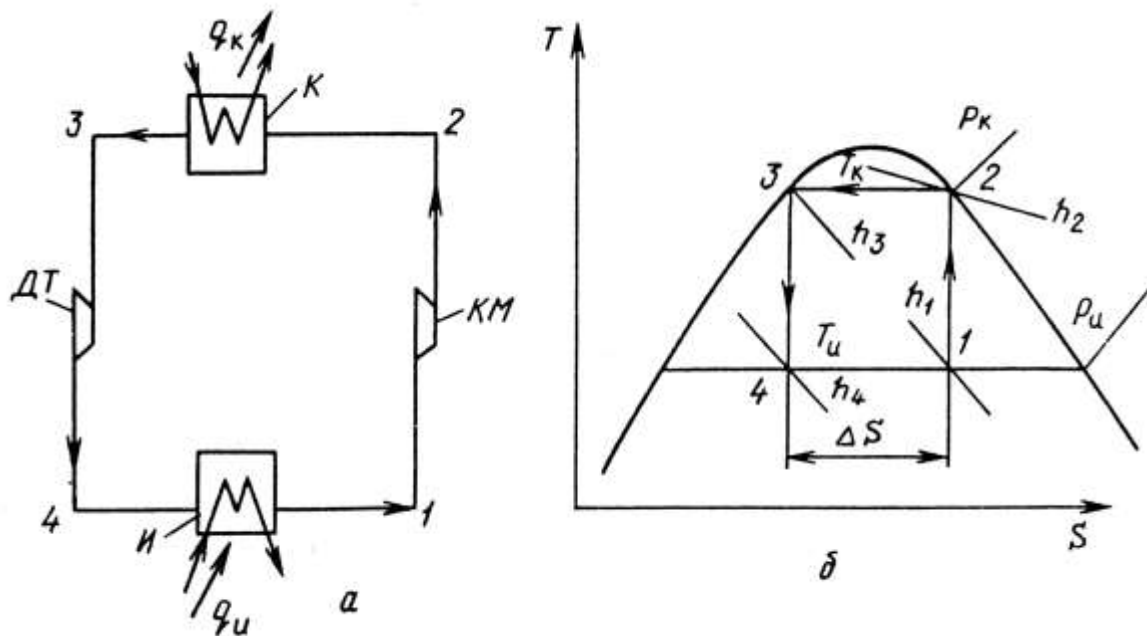
Рис. 3.29. Ідеальний тепловий насос: а – принципова схема; б – круговий цикл у діаграмі T-S ; КМ – компресор; К – конденсатор; ДТ – детандер; И – випарник
