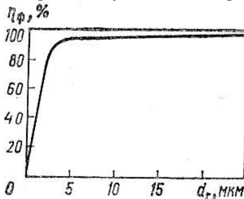
Рис. 2.12. Залежність ефективності ротоклону від фракційності уловлюваного пилу
