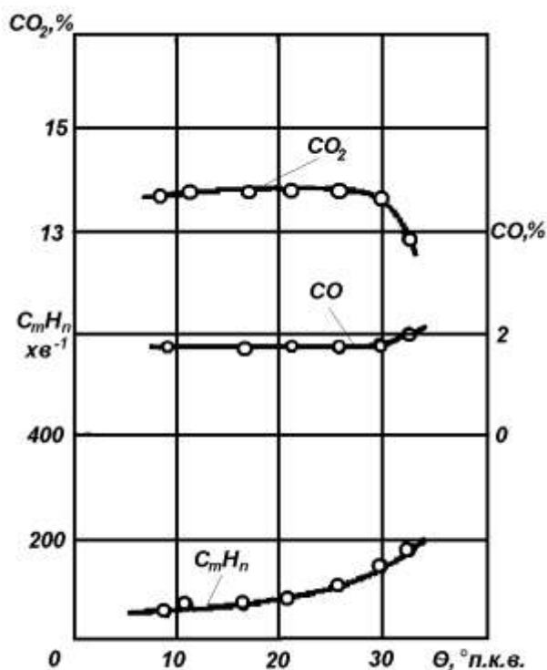
Рис. 2.33. Вплив кута випередження запалювання у бензиновому двигуні на вміст окремих компонентів у відпрацьованих газах
