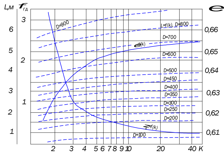
Рис. 3.45. Номограма для визначення довжини L впливу діафрагми для коефіцієнтів опору \zeta_g і стиснення струменя \varepsilon за заданими K і D
