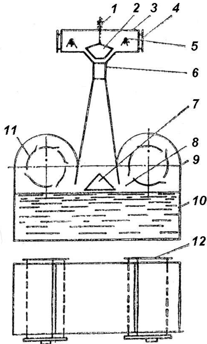
Рис. 2.16. Абсорбційний пристрій типу ТММ для очищення газів
