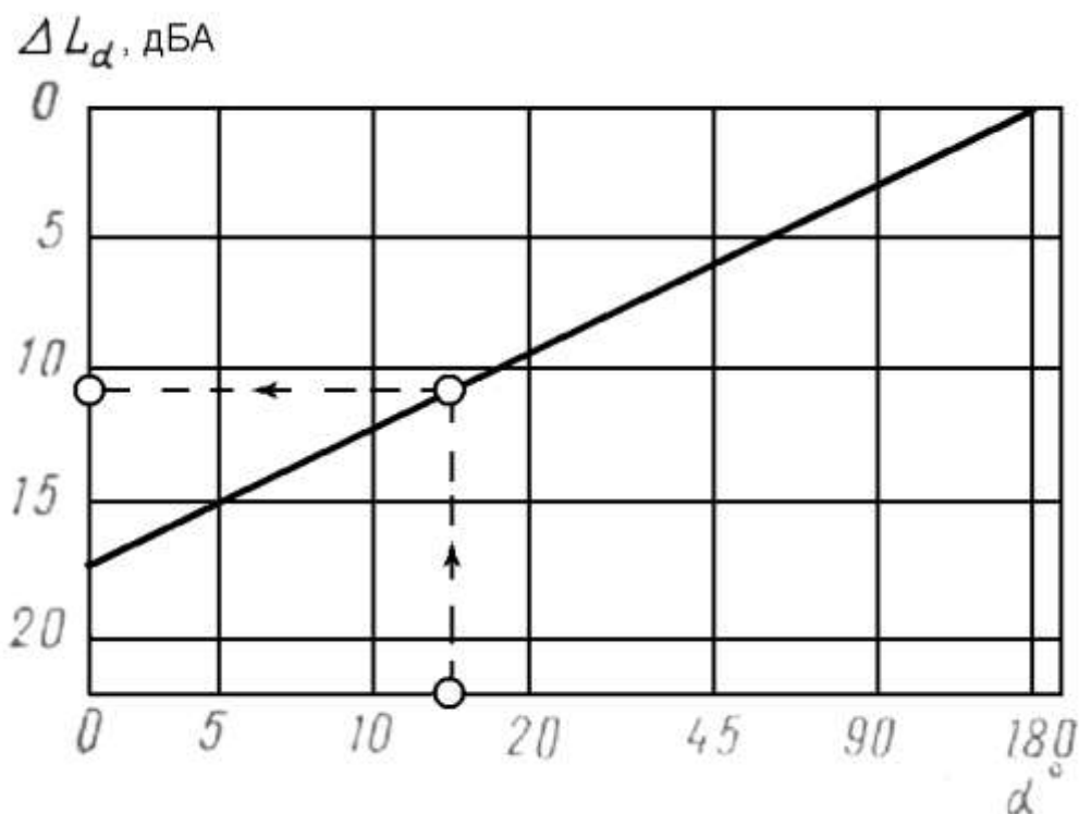
Рис. 2.31. Графік для визначення зниження рівня шуму внаслідок обмеження кута огляду вулиці (дороги) з розрахункової точки
