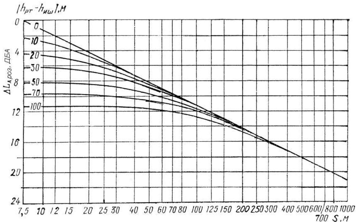
Рис. 2.22. Графік для визначення зниження рівня шуму залежності від відстані між джерелом шуму і розрахунковою точкою та від різниці їх висот
