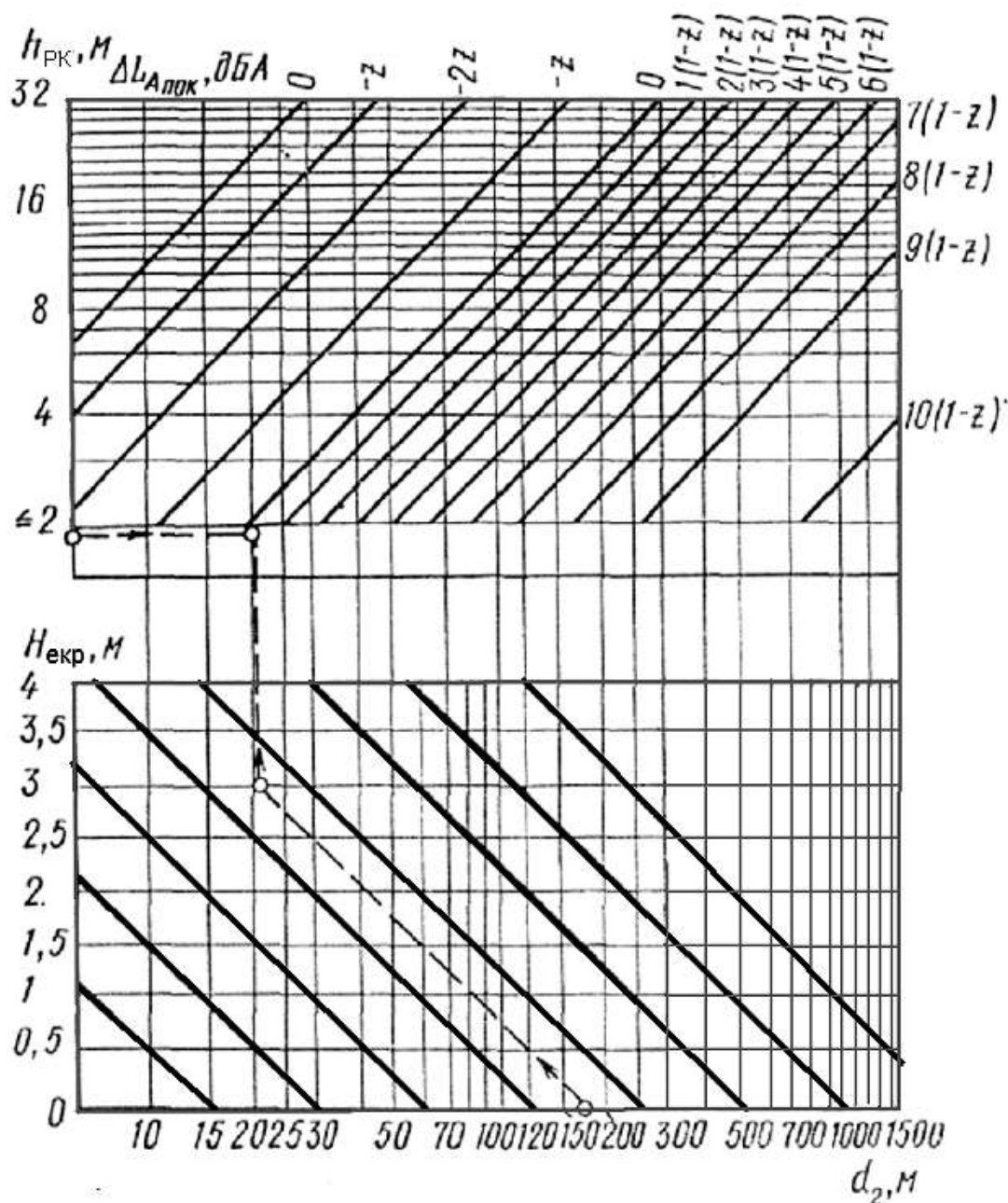
Рис. 2.29. Номограма для визначення зниження рівнів шуму за екраном внаслідок його поглинання акустично-м'яким покривом території
