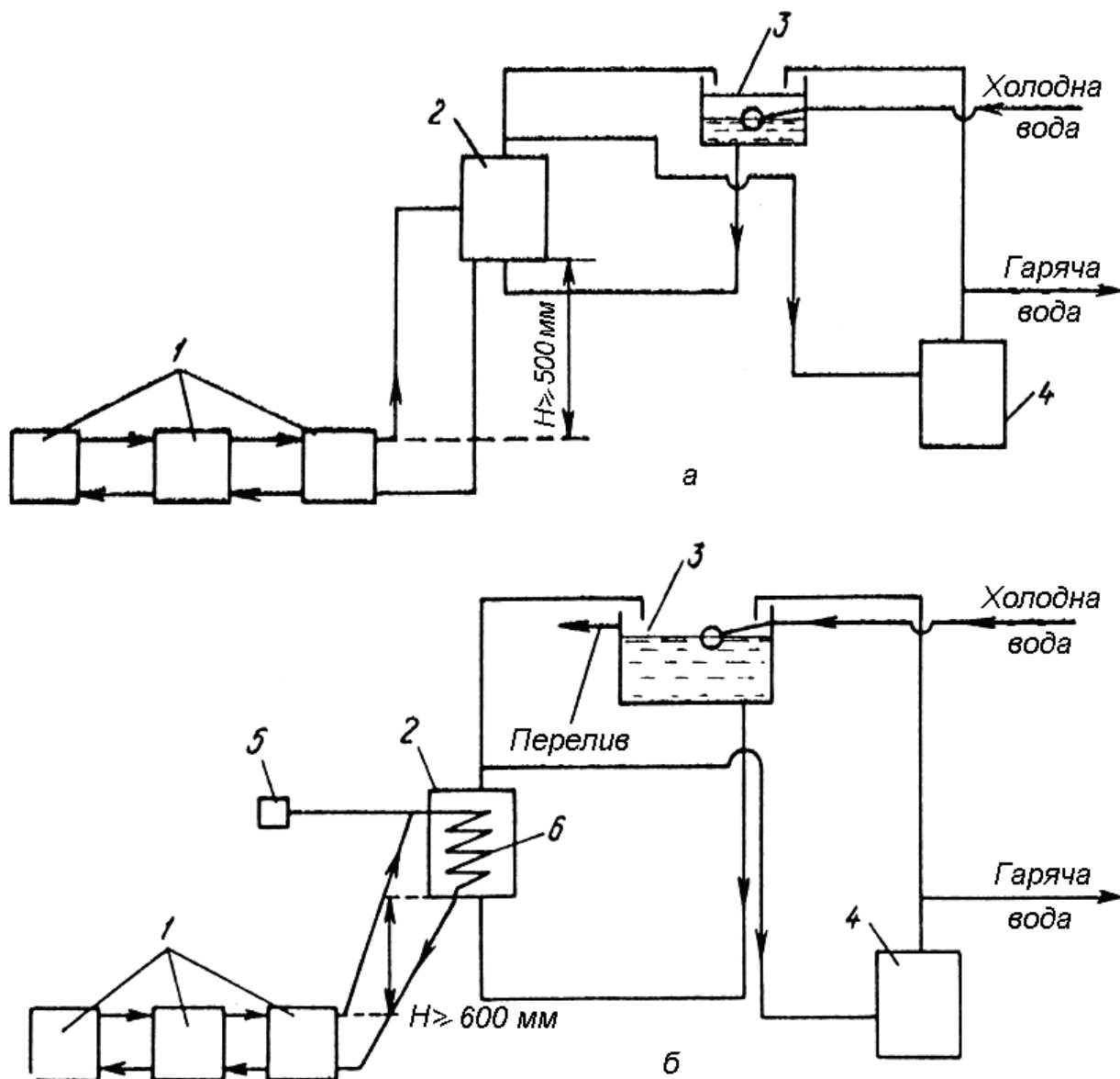
Рис. 3.36. Термосифонна система гарячого водопостачання: а – одноконтурна; б – двоконтурна; 1 – плоскі сонячні колектори; 2 – бак-акумулятор; 3 – бак холодної води; 4 – додаткове джерело тепла (колонка); 5 – герметичний розширювальний бак; 6 – теплообмінник
