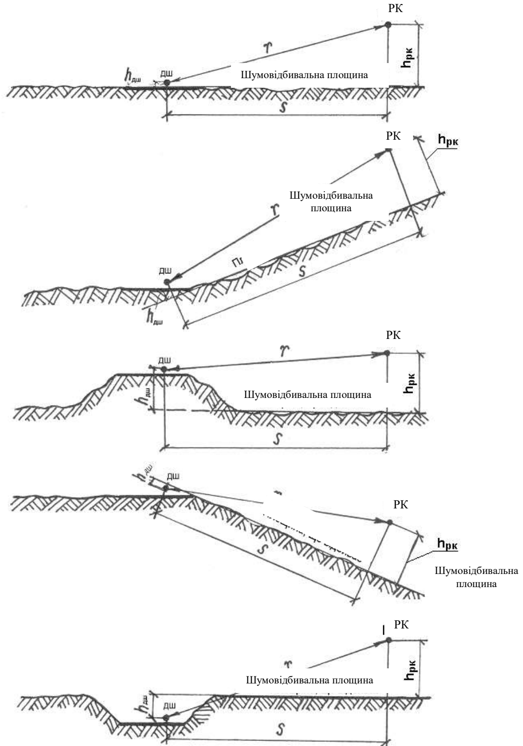
Рис. 2.23. Поперечні профілі транспортних шляхів і прилеглих ділянок для різних видів розташування проїзної частини відносно рівня поверхні території
