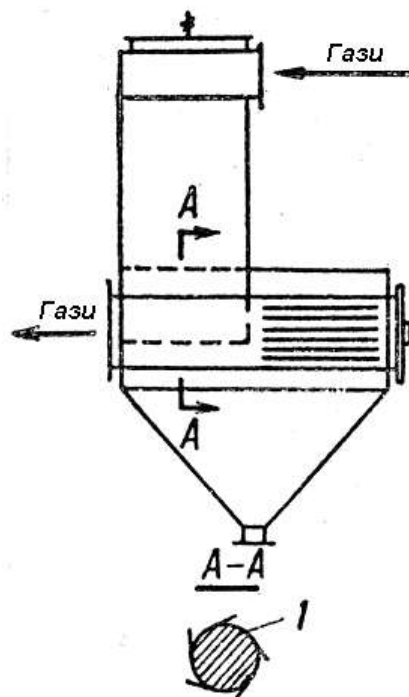
Рис. 2.6. Пориста фільтраційна набивка 1 у очищальному пристрої типу ТМС
