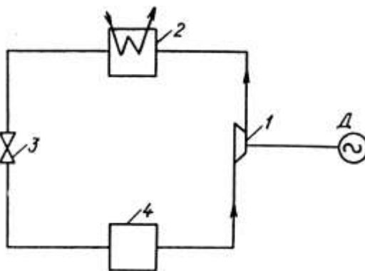
Рис. 3.31. Схема теплового насоса
