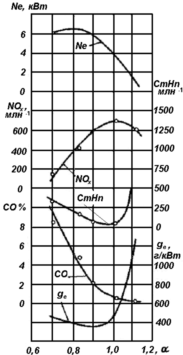
Рис. 2.31. Вплив складу паливної суміші на показники роботи бензинового двигуна
