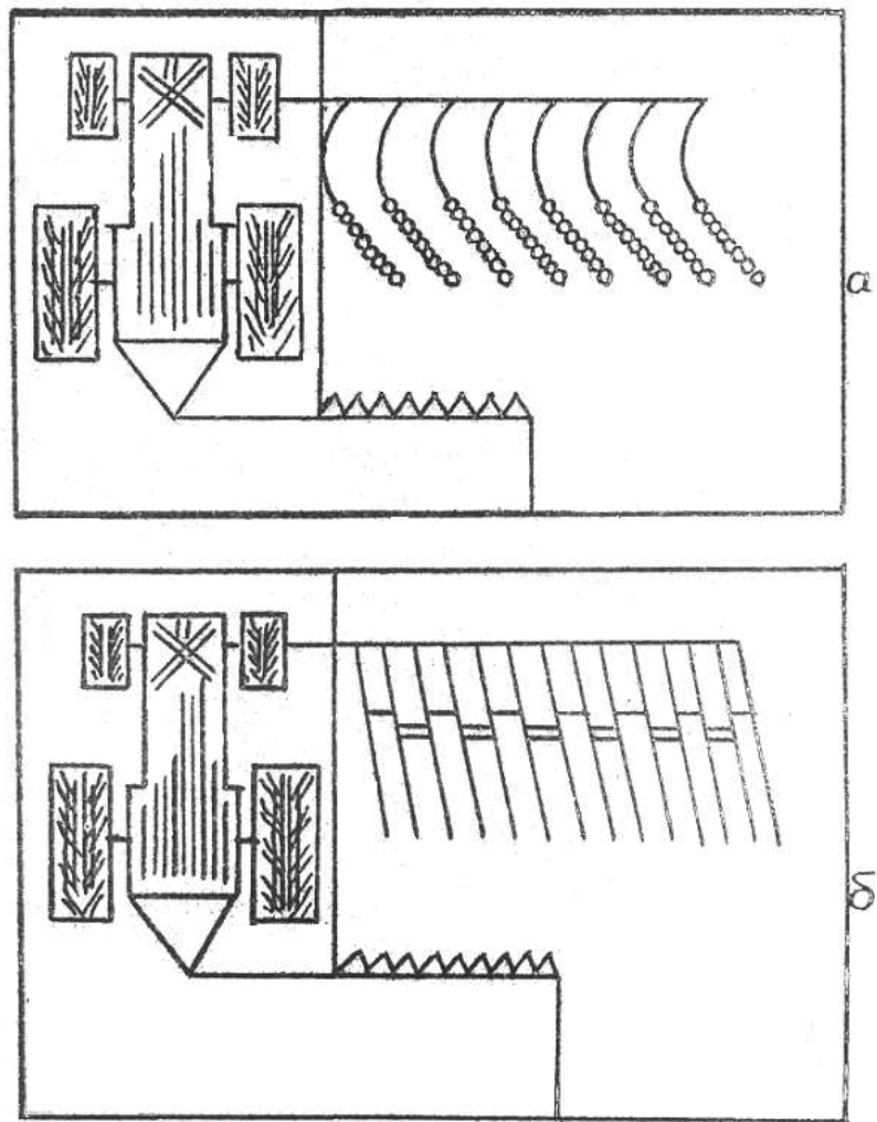
Рис. 5.4. Виполохуючий пристрій: а) – з ланцюгів; б) – з пружинними прутами
