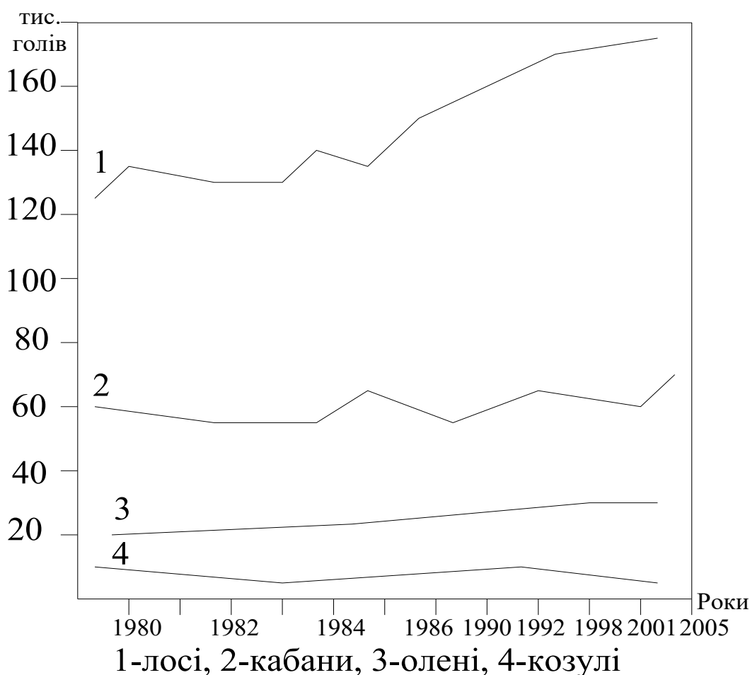
Рис. 2.12. Динаміка чисельності основних видів мисливських тварин в Україні
