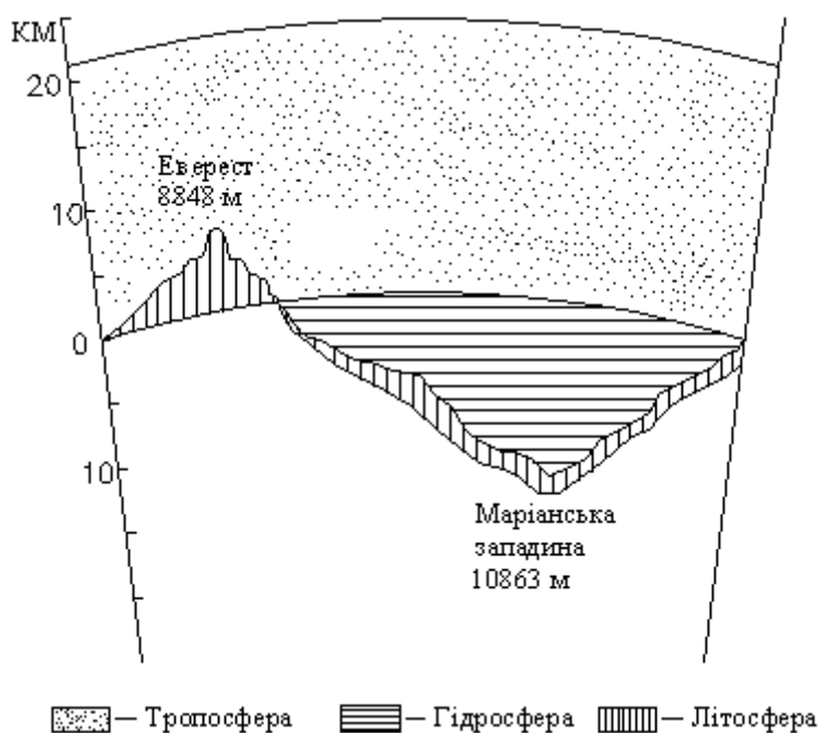
Рис. 1.9. Межі проникнення життя в біосфері
