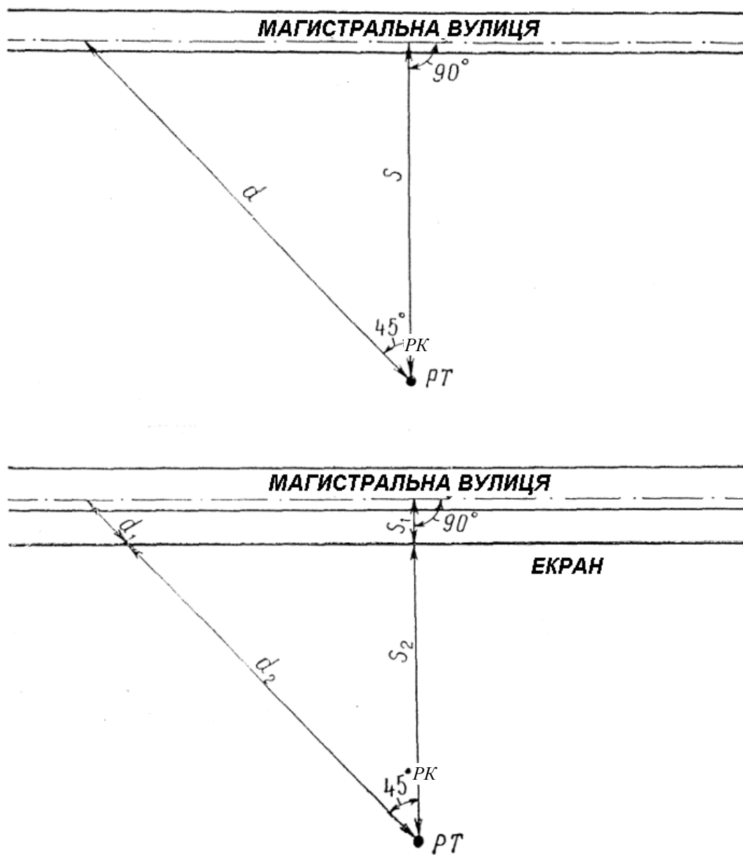
Рис. 2.25. Схеми для визначення розрахункової відстані
