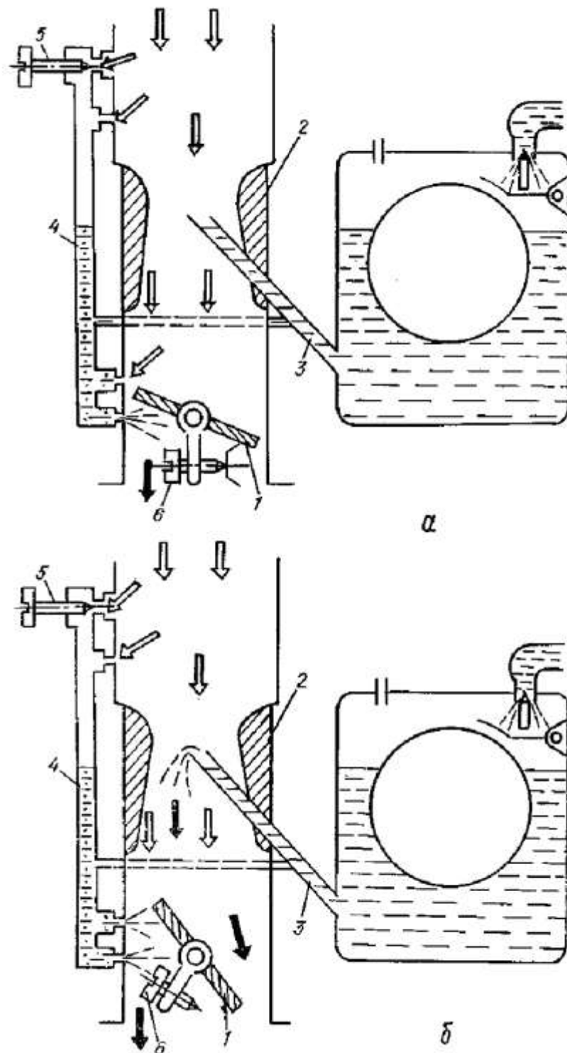
Рис. 2.34. Робота карбюратора в режимі n_{\min} (а) і n_{\text{підв}} (б) під час контролювання бензинового двигуна на допустимий вміст шкідливих речовин у відпрацьованих газах:
