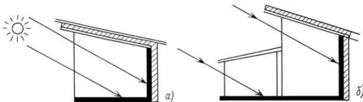
Рис. 3.39. Пасивний сонячний нагрівач: основна система (а) і вікно у ліхтарі (б) для прямого нагрівання задньої стіни будівлі (стрілками показано, де використано масивні, забарвлені у чорний колір поверхні з посиленою теплоізоляцією для поглинання і накопичення сонячного тепла)
