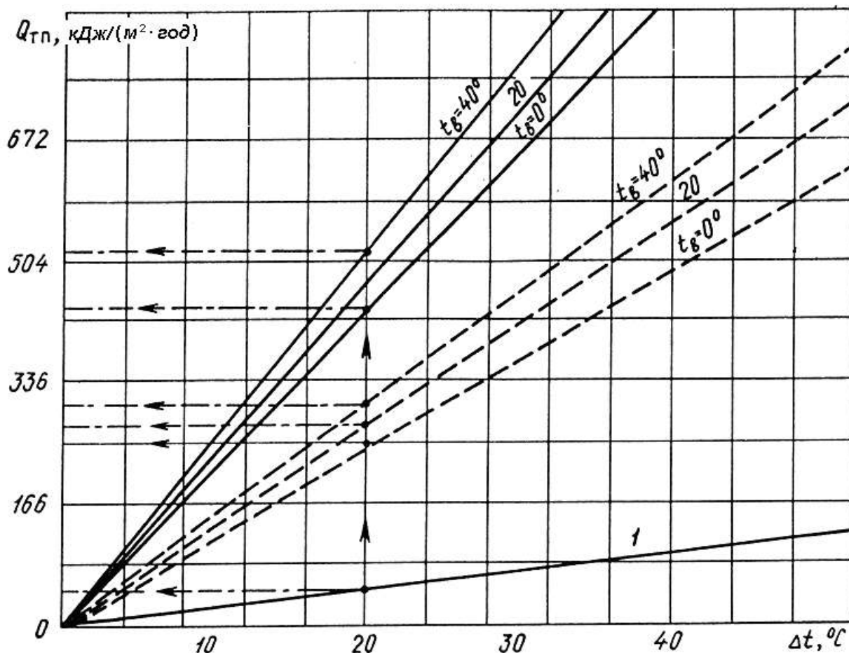
Рис. 3.20. Залежність теплових втрат Q_{т.п} колектора трубчастого типу від різниці температур \Delta t між поверхнею нагрівання і довколишнім повітрям:
