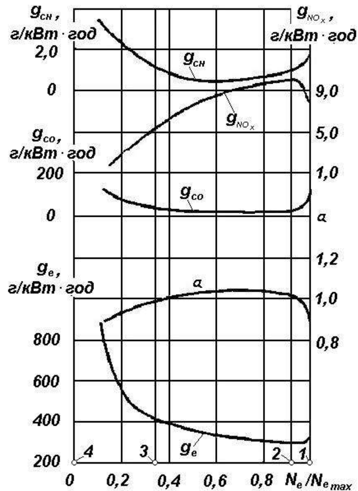
Рис. 2.35. Навантажувальна характеристика роботи бензинового двигуна
