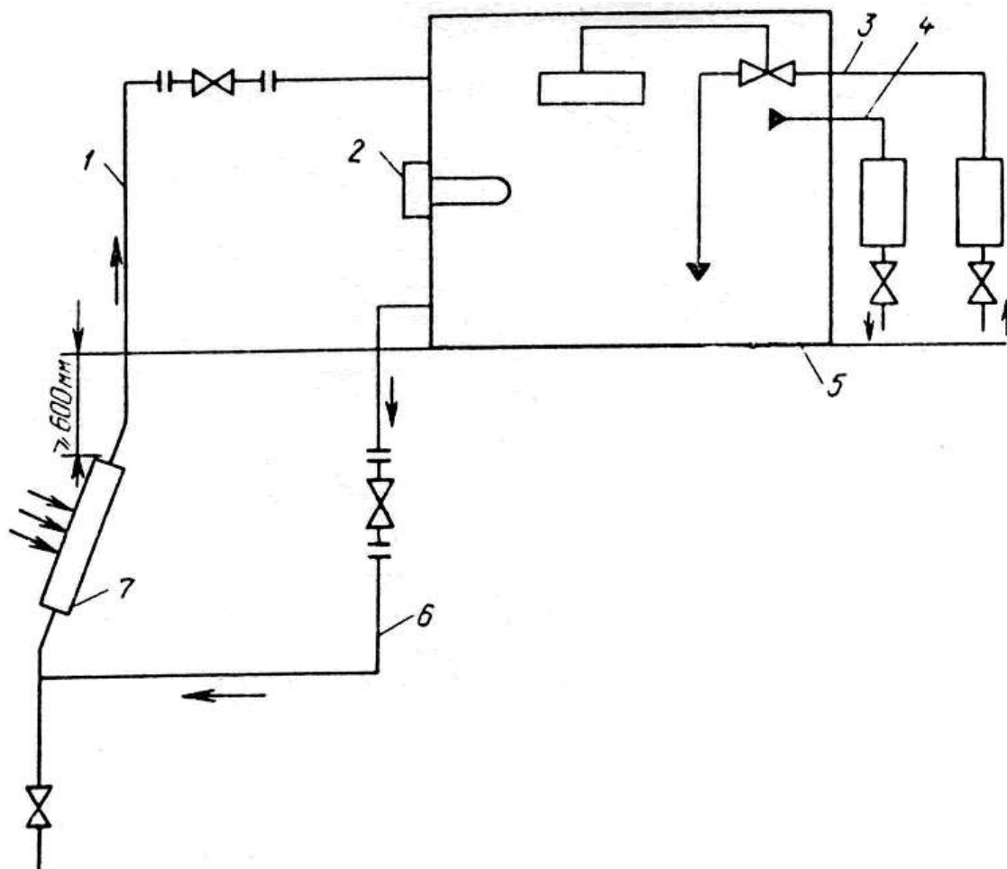
Рис. 3.33, а. Схема підігрівання води на доїльному майданчику
