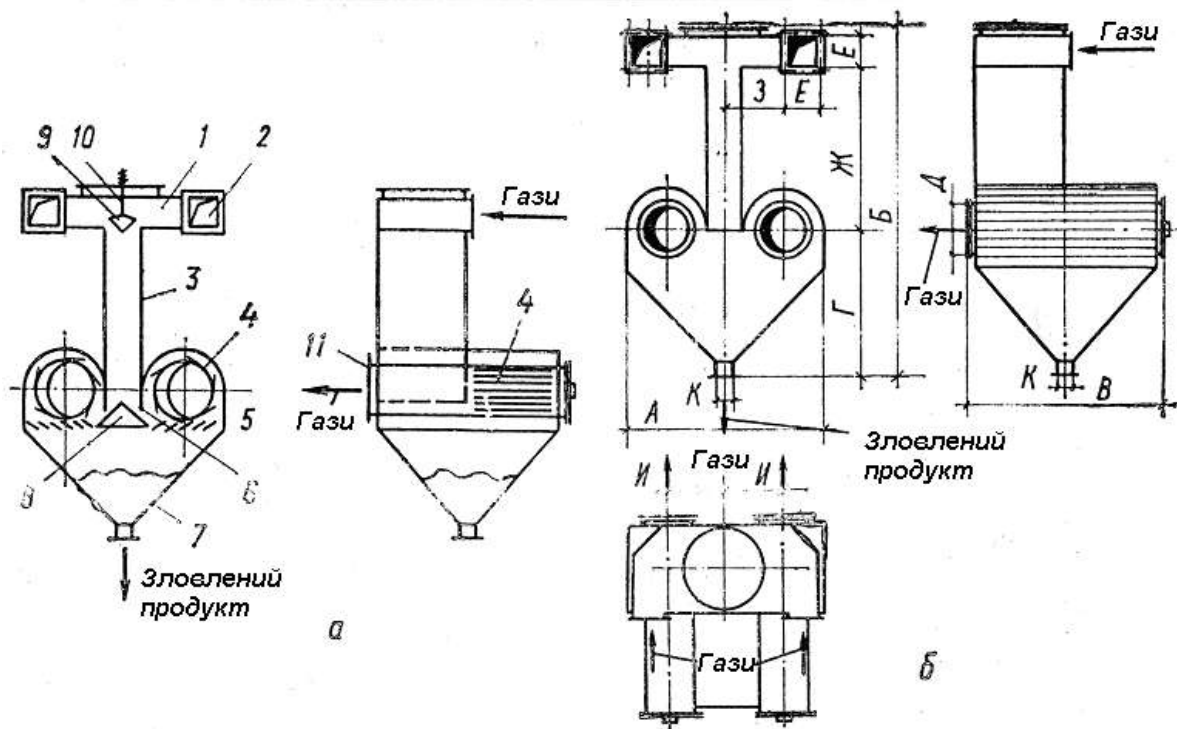
Рис. 2.5. Принципова схема очищального пристрою типу ТМС (а) і приєднувальні розміри (б)
