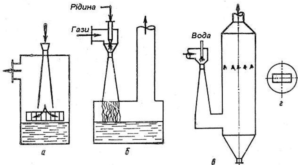
Рис. 2.15. Скрубери Вентурі:
