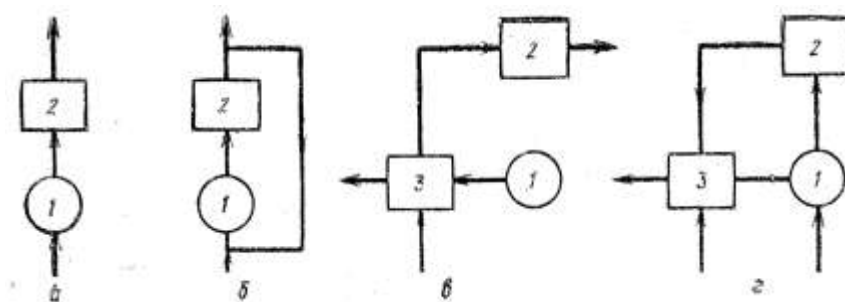
Рис. 2.17. Схеми каталітичного знешкодження газових викидів а – без рециркуляції газів; б – з частковою рециркуляцією газів; в – з теплообмінником на димових газах; г – з теплообмінником змішувача; 1 – підігрівач; 2 – реактор; 3 – теплообмінник
