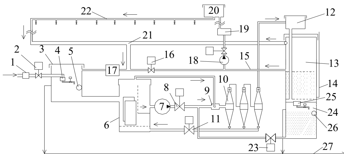
Рис.2.9. Технологічна схема автоматичної системи безпечного водопостачання
