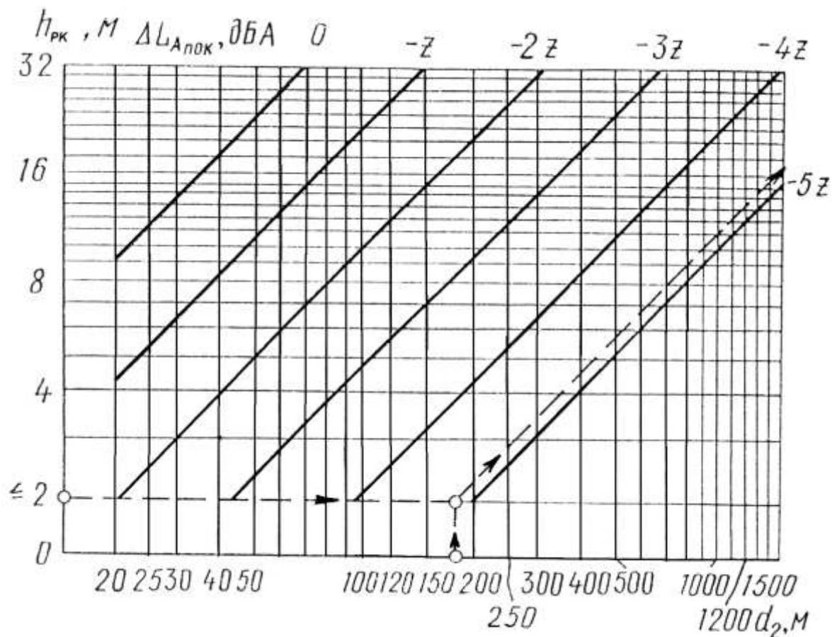
Рис. 2.30. Номограма для визначення підвищення рівня шуму внаслідок його відбиття від акустично-жорсткого покриття території за екраном
