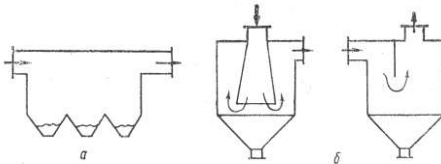
Рис. 2.1. Пиловловлювачі:
