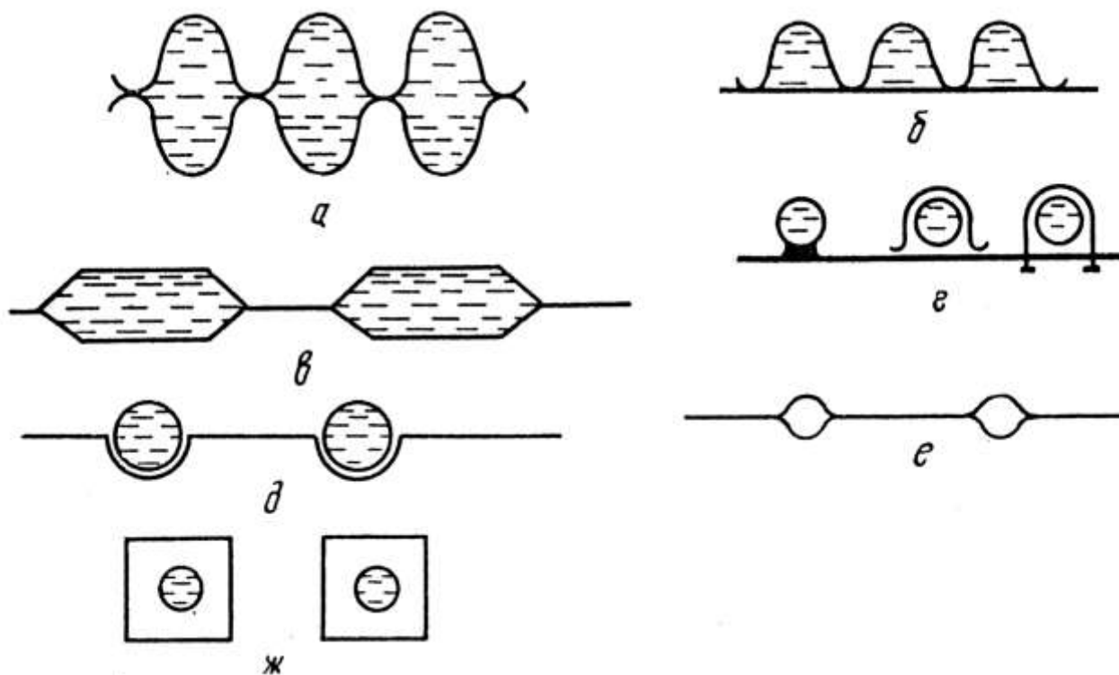
Рис. 3.13. Поперечний переріз поглинальних пластин:
