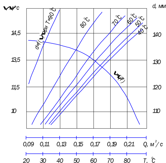
Рис. 3.43. Номограма для визначення швидкості w і діаметра отвору діафрагми d за заданими T_i і Q_i
