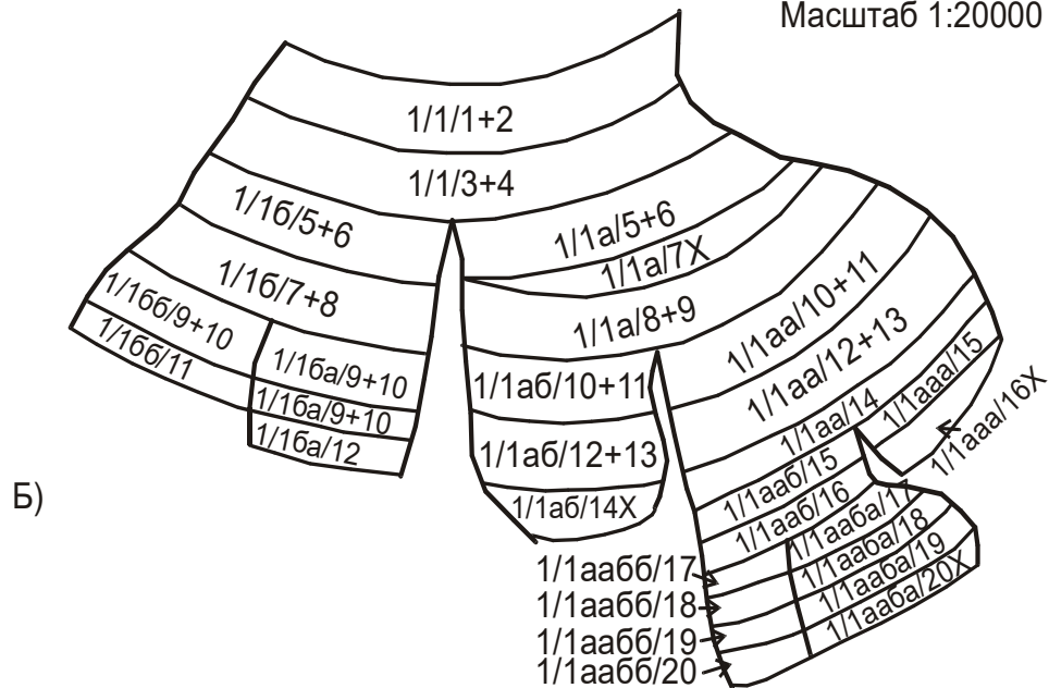
Рис. 14.14 Конкретні приклади застосування логічної формули присвоєння номерів підрозділам агроландшафтно реорганізованих угідь. Аркуш 1
