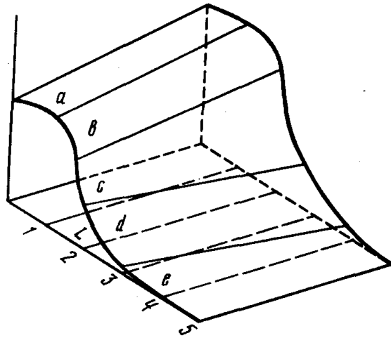
Рис.15.2. Співвідношення метричних мір (1,2,3,4,5) і позиційних мір (a,b,c,d,e) нахилі (складено за В.А. Боковим)
