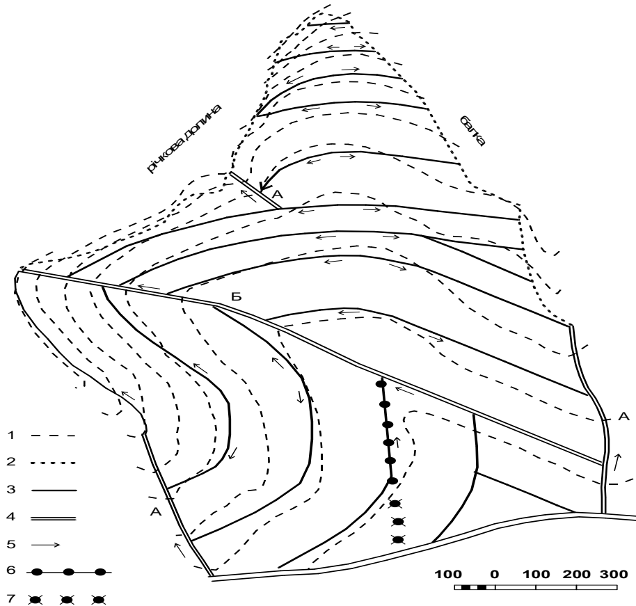
Рис. 14.1. Стоковідвідний характер рубезів контурно-смугової просторової структури агроландшафтів на ріллі земельного масиву, обумовленого геоморфологічно, а з півдня вздовж вододільної лінії обмеженого істотним антропогенним рубезем.
