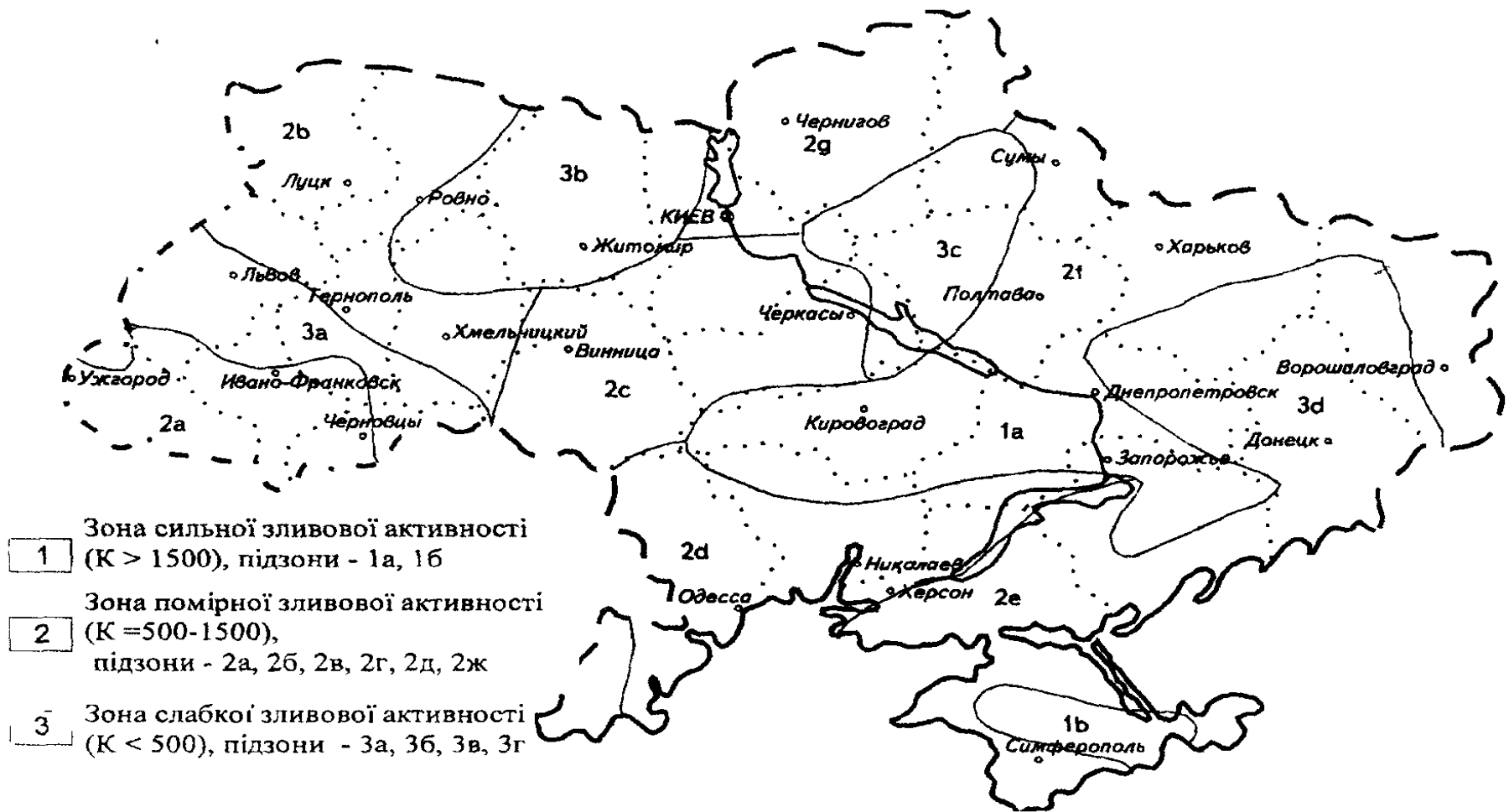
Рис.12.1. Злизова небезпека на території України
