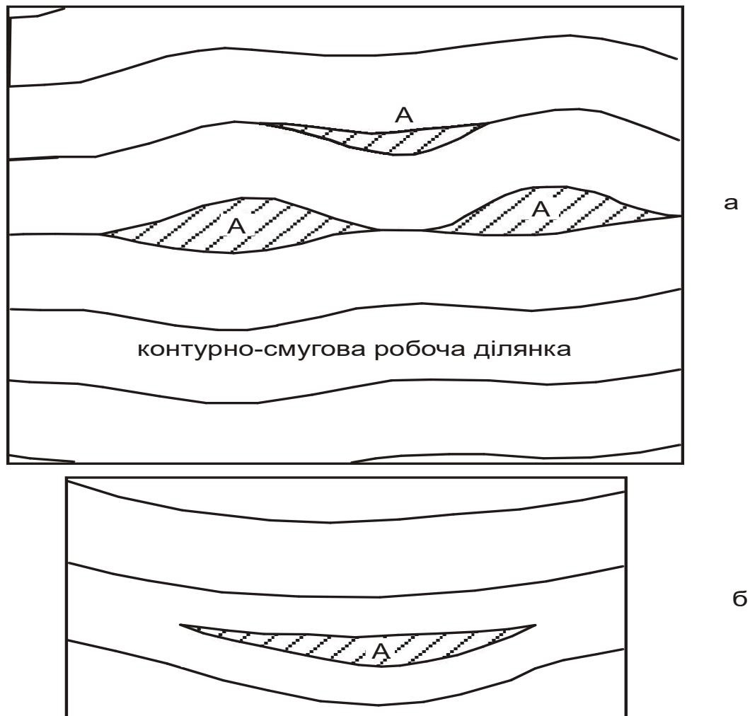
Рис. 14.7. Якщо привододільний простір являє собою вузьку смугу горбів і сідловин, що чергуються (“стрічковий плакор”), можливо вивести до вододільної лінії коректуючі клини (А), розмістивши їх: а) між контурно-смуговими робочими ділянками або між схилівими блоками протилежних експозицій; б) посередині робочої ділянки
