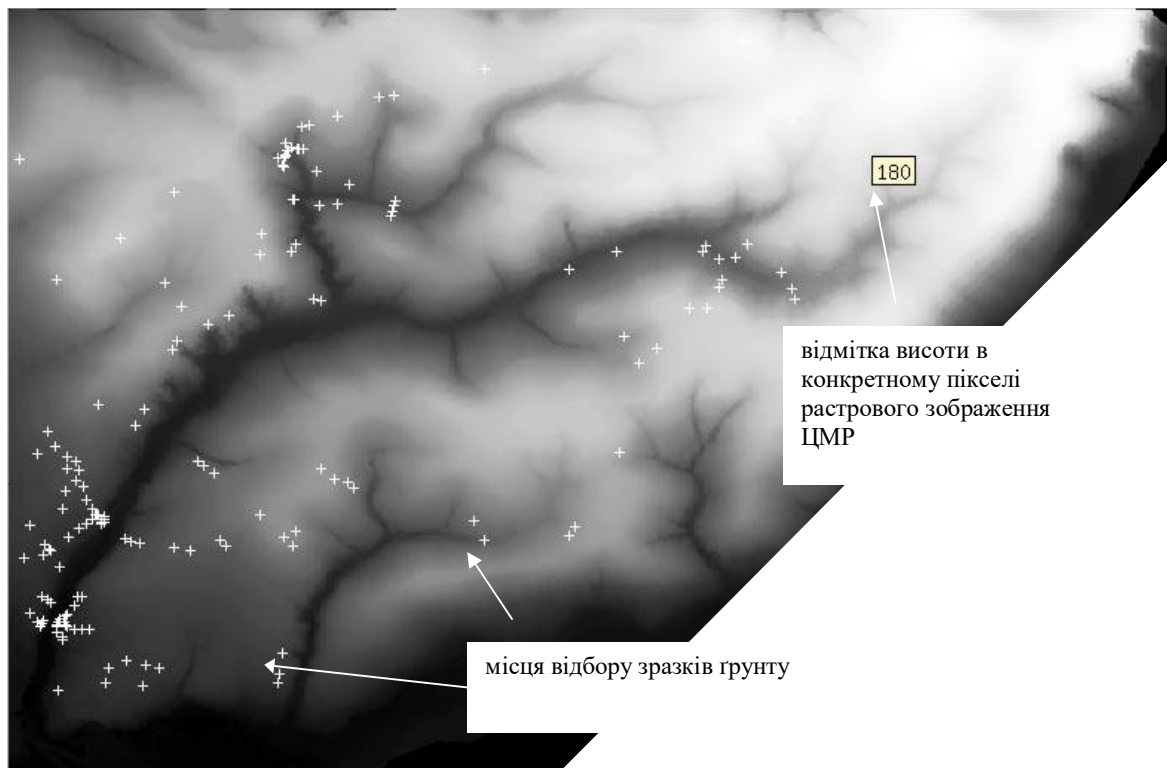
Рис. 15.15.– Цифрова модель рельєфу ландшафтного парку “Печенізьке поле”
