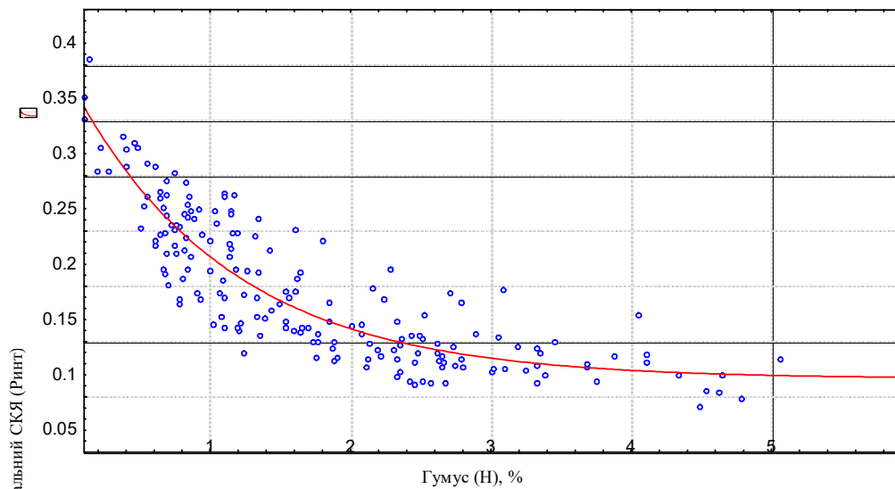
Рис.8.1. Зв'язок між Рінт та Н для ґрунтів Лісостепу та Сухого Степу
