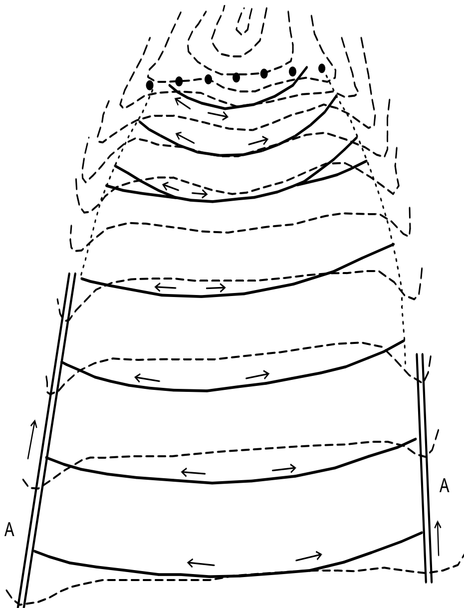
Рис. 14.3. Якщо на міжuloговинно-міжбалковій частині земельного масиву переважають прямолінійні горизонталі, стоківідвідний характер рубежам надається через деяку їхню увігнутість.
