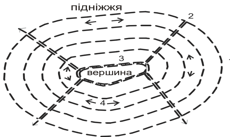
Рис. 14.10. Організація території поверхні куполоподібного підвищення (без істотного вздовжсхилового розчленування): вгорі — контурно-спіральна; внизу — у вигляді схилових блоків контурно-смугових робочих ділянок:
