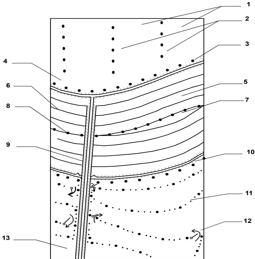
Рис. 14.5. Ілюстративний приклад деталізованого плану розміщення заходів постійної дії на місці стику мікрозони А з двома схиловими блоками контурно-смугових робочих ділянок, орних і пасовищних
