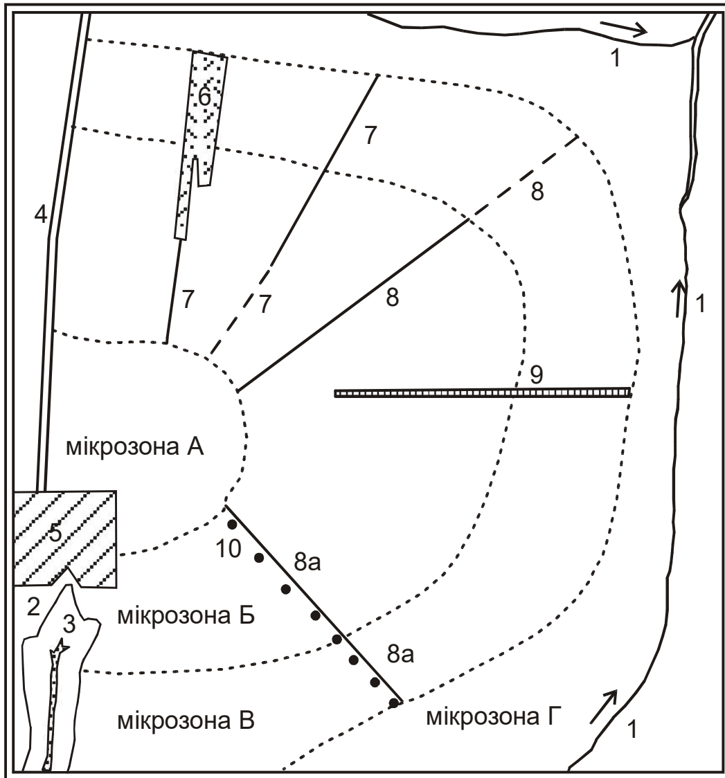
Рис. 14.8. Ілюстративна схема прикладу поділу мікрозон Б+В
