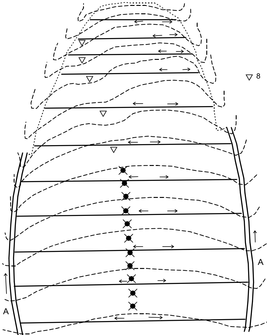
Рис. 14.2. При слабовипуклих горизонталях на міжулоговинно-міжбалковій частині орного земельного масиву безпечно відведення стоку забезпечується прямолінійними (або близькими до прямолінійних) рубежами.
