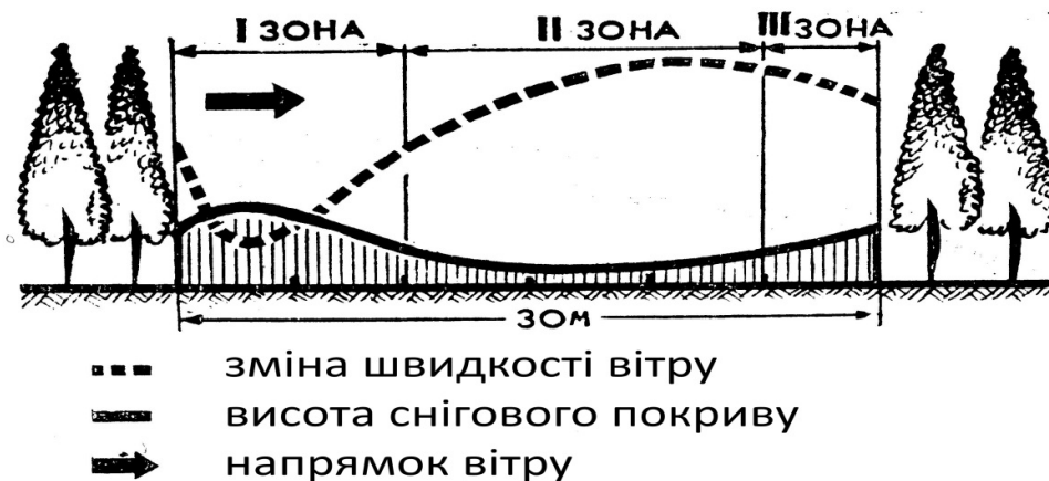
Рис. 15.4. Відкладення снігу за лісосмугою.
