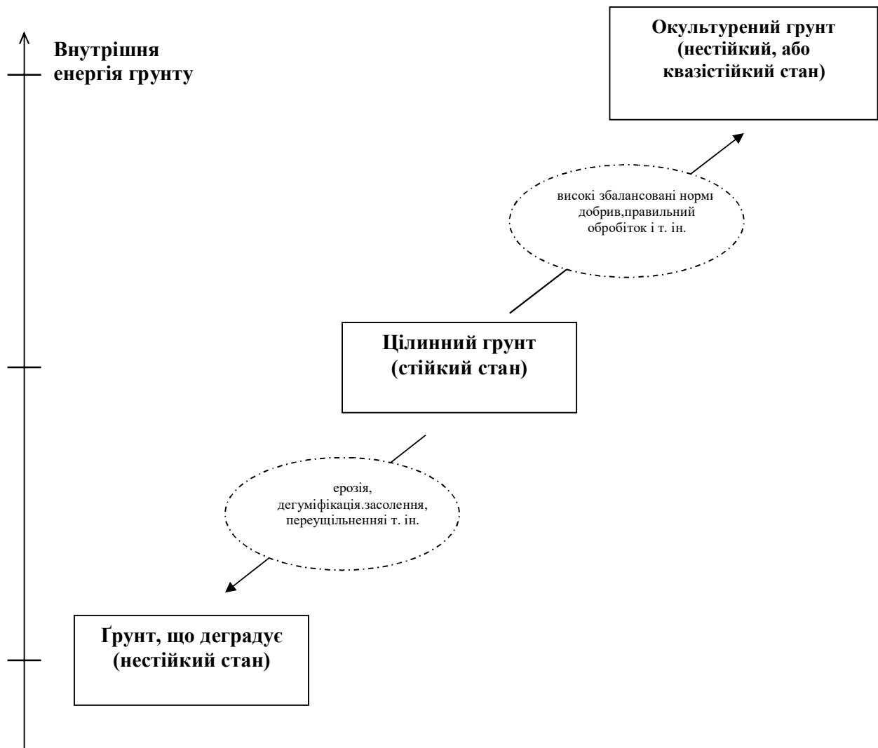
Рис. 3.2. – Схема зміни станів ґрунту
