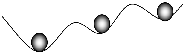
Рис. 3.3. – Стійкість ґрунту на різних енергетичних рівнях
