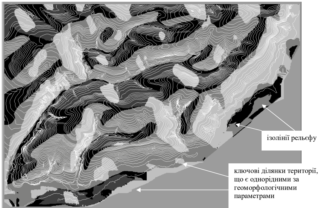
Рис. 15.9.Електронна карта ключових ділянок території однорідних за геоморфологічними параметрами.
