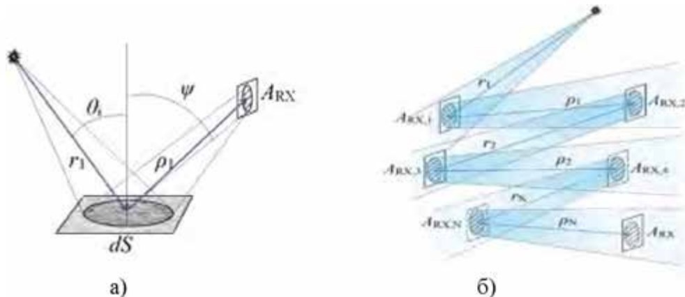
Рисунок. 1 Розсіювання хвиль ММД при відбитті на шорстких поверхнях: а) одне відбиття, б) багаторазове відбиття
