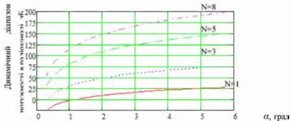
Рисунок.2 Розрахована залежність динамічного діапазону потужності в радіоканалі в залежності від кута розкриття антени \alpha
