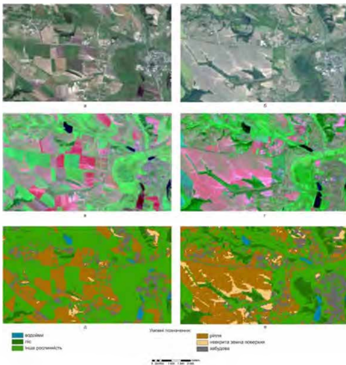
Рис.1. Супутниковий знімок: а – Landsat-5 TM за 1985 р.; б – Landsat-8 OLI за 2019 р. Композит каналів супутникового знімка: в – Landsat-5 TM за 1985 р.; г – Landsat-8 OLI за 2019 р. Землекористування частини Шумської ОТГ; д – за 1985 р.; е – за 2019 р.
