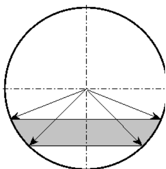
Рис. 2. Сферичне відображення нормалей поверхні
