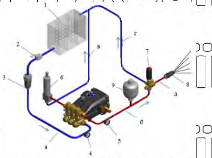
Рис. 3.9. Схематичне зображення підключення насосу високого тиску
