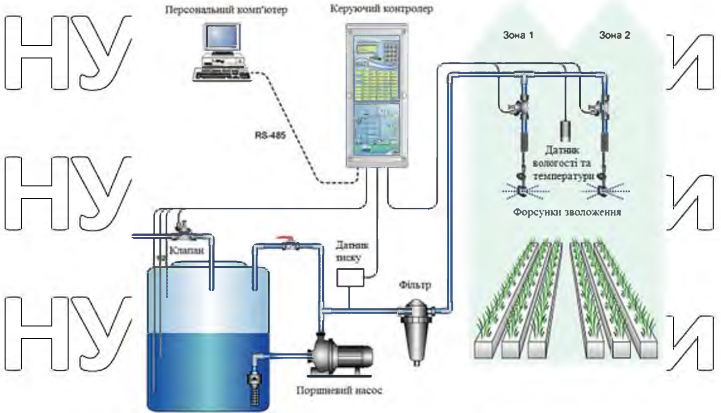
Рис. 3.6. Загальний вигляд системи туманоутворення
