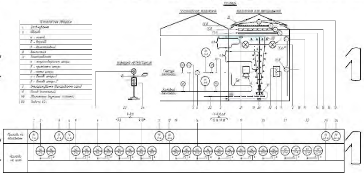
Рис. 2.9. Функціонально-технологічна схема управління технологічними процесами в теплиці з умовним зображенням щита керування
