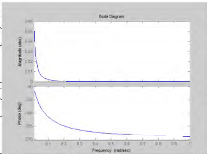
Рис. 3.16. Амплітудно-частотна характеристика автоматизованої системи керування вологістю
