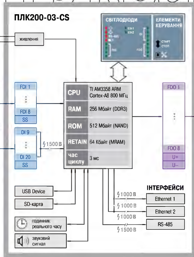
Рис. 3.23 Функціональна схема ПЛК200-03-CS
