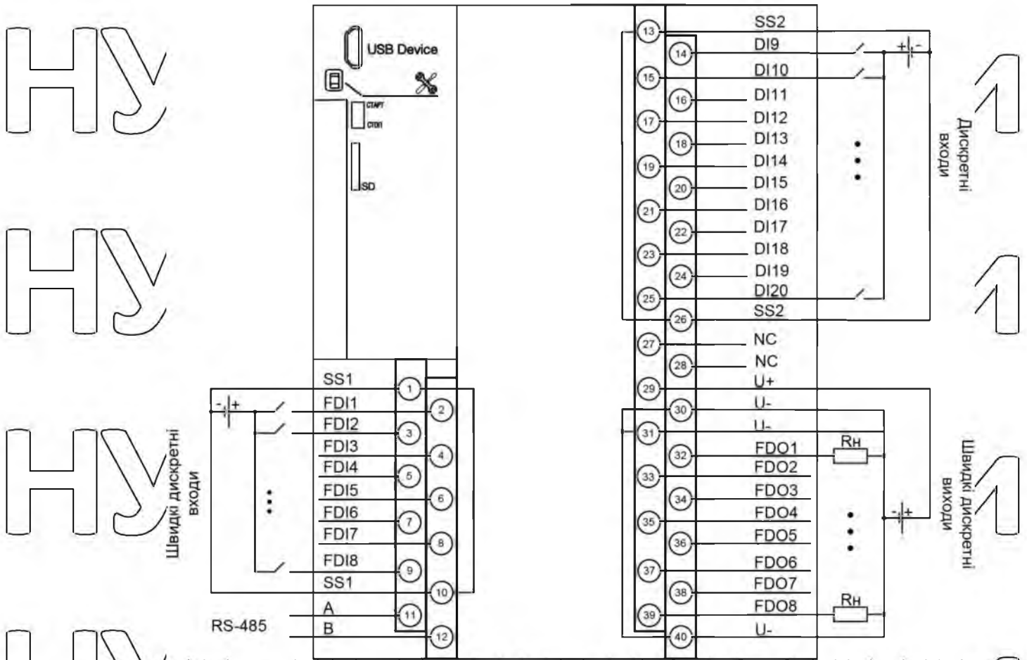
Рис. 3.25 Схеми входів і виходів в ПЛК200-03-CS
