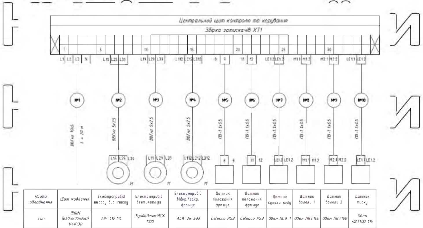
Рис. 4.3. Електрична схема підключень системи автоматичного керування вологісним режимом в теплиці
