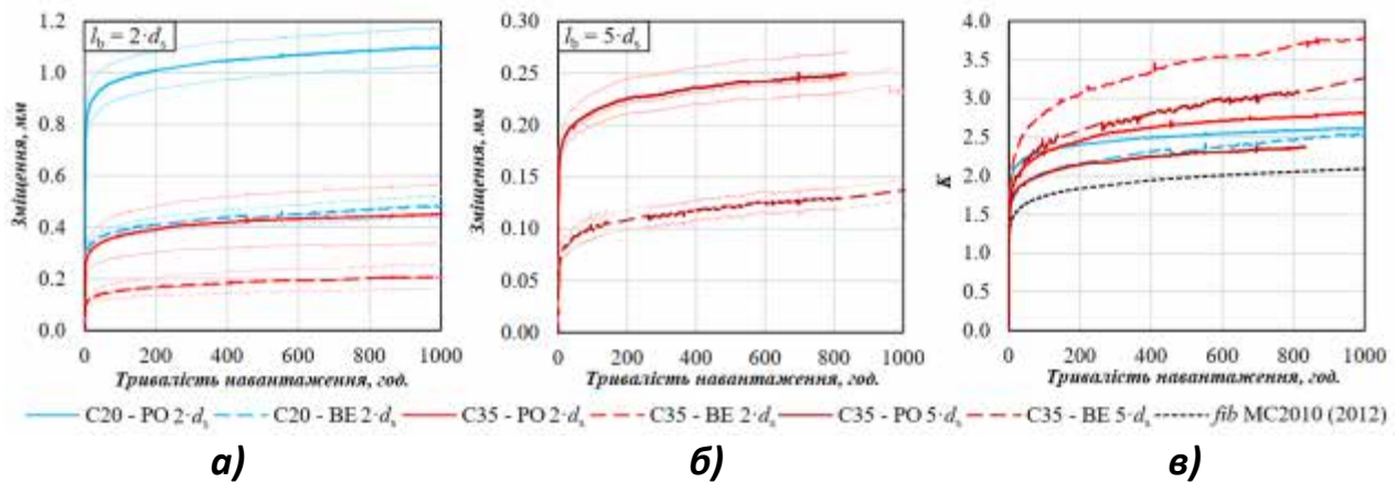
Рис. 3. Збільшення проковзування арматури при дії довготривалого навантаження для різних випробувань та класів бетону (PO – висмикування, BE - балочне) [5]:
