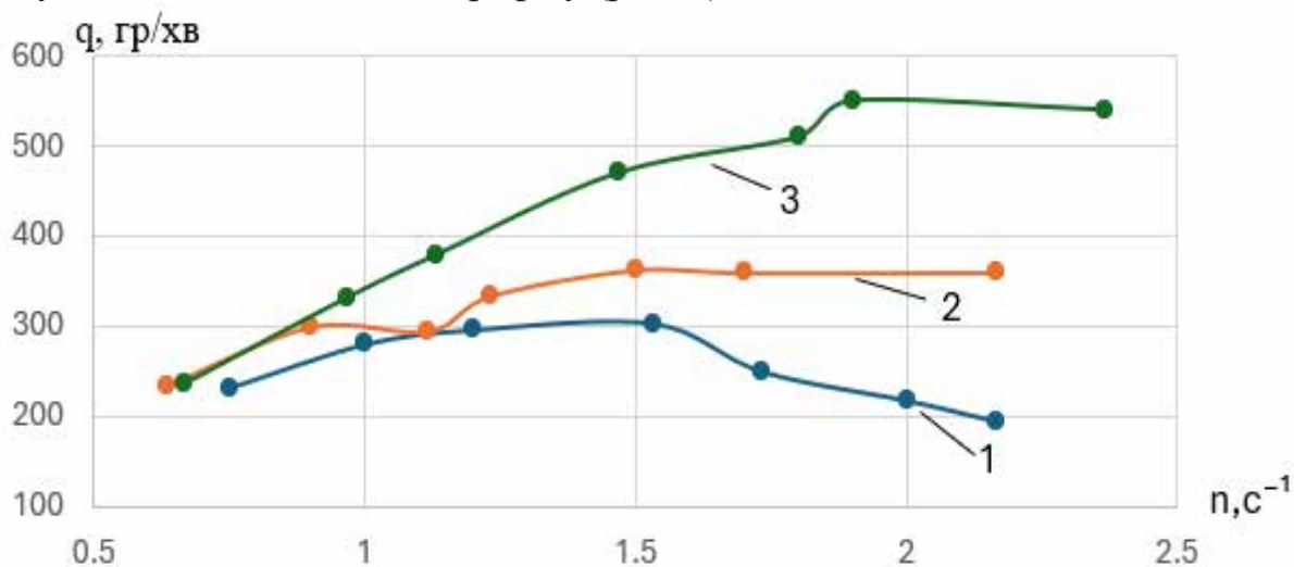
Рисунок 3 - Продуктивність дозатора залежно від розмірів вікон (1-впускне 35x17, випускне 35x17; 2- впускне 60x17, випускне 35x17; 3- впускне 60x17, випускне 60x17)
