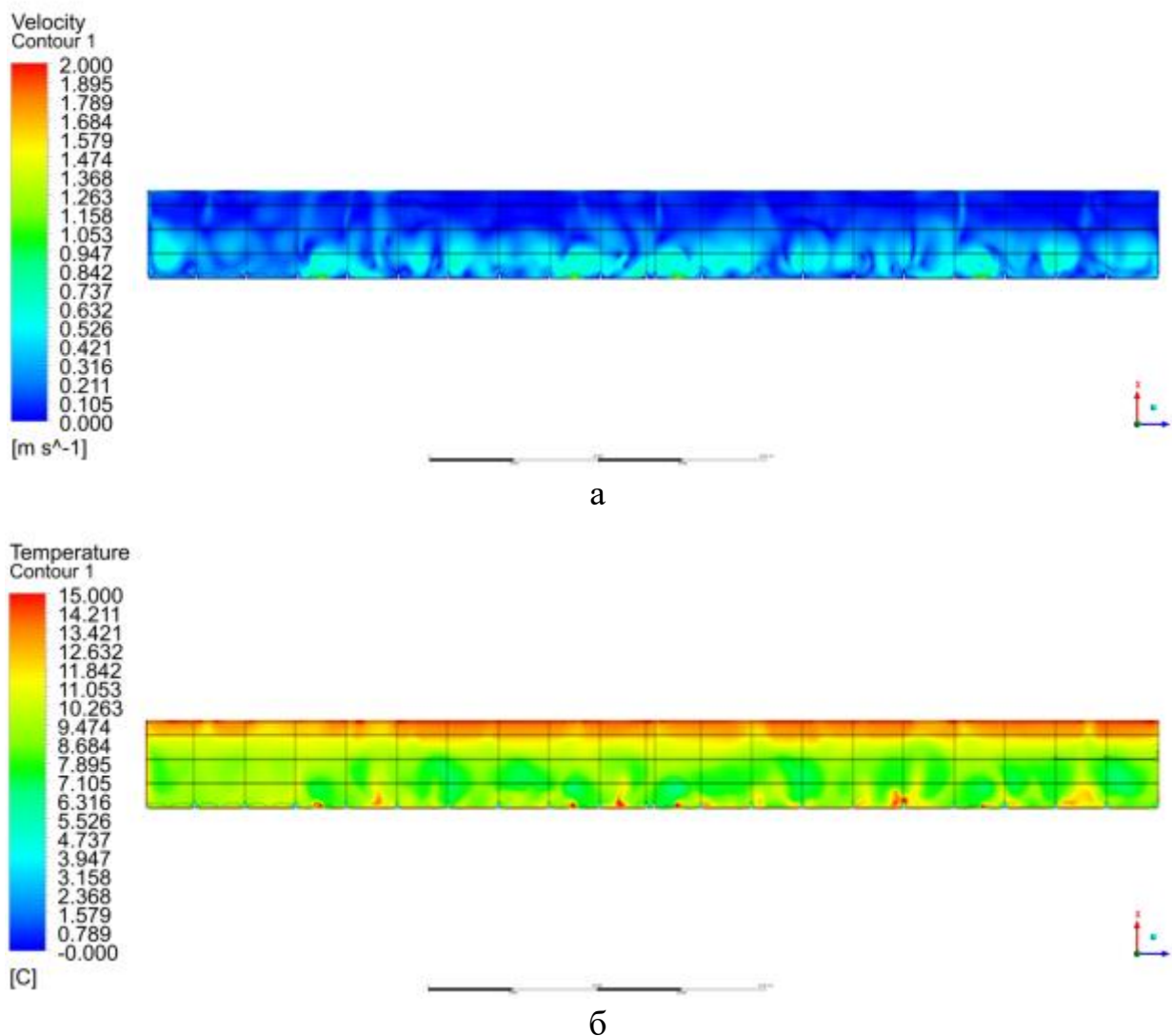
Рис. 2 – Поле швидкостей, м/с (а), та поле температур, °С (б) в приміщенні пташника на висоті 0,7 м від рівня підлоги
