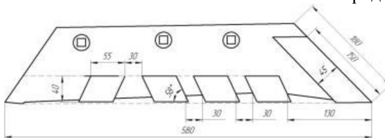
Рисунок 5 – Схема відновлення плужного лемішу постановкою компенсуючих вставок
