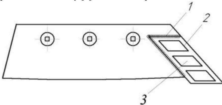
Рис. Спосіб відновлення і зміцнення носової частини плужного лемеша зі стертям і променевим зношенням:
