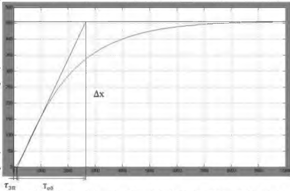
Рисунок 2.4 – Крива розгону по каналу регулювання температури
