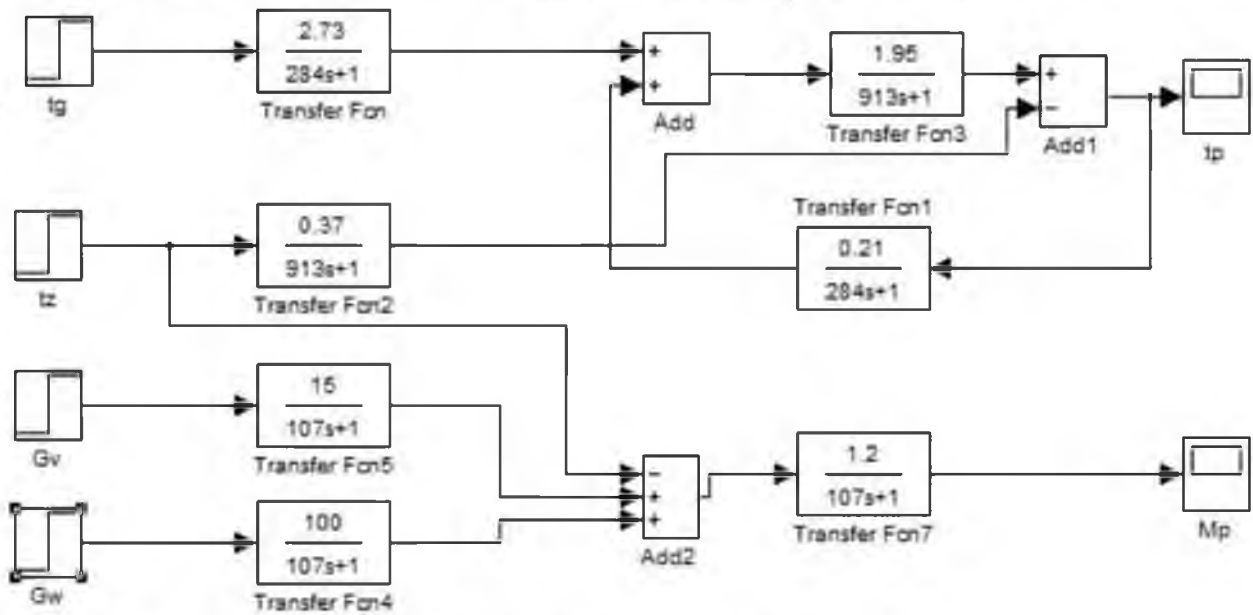
Рисунок 2.3 – Математична модель об'єкта
