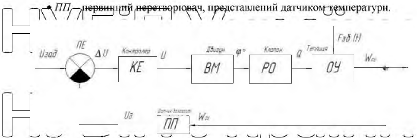
Рисунок 2.17 – Функціонально-структурна схема системи автоматичного керування по каналу вологості
