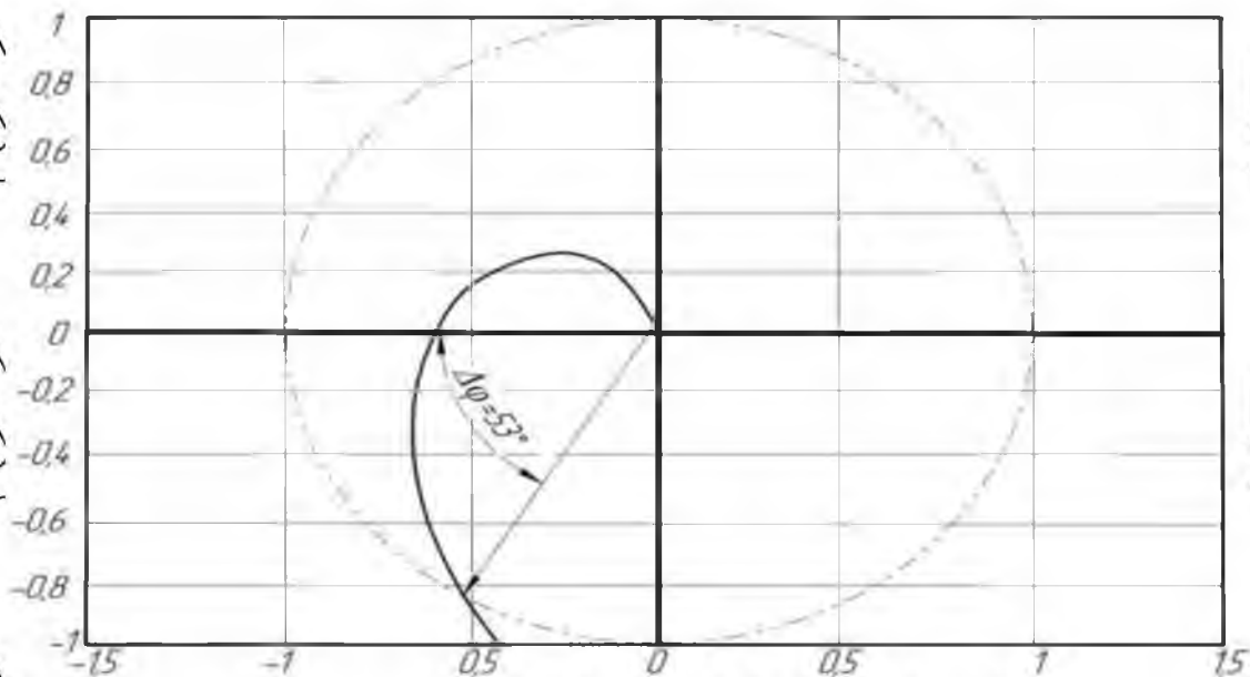
Рисунок 2.20. Голограф Найквіста за каналом регулювання температури
