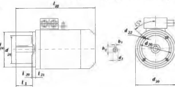
Рисунок 2.25 – Електродвигун AIP80B4
