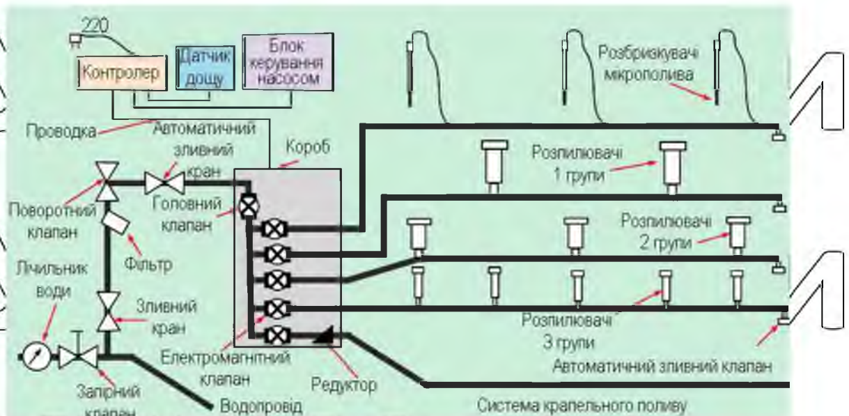
Рисунок 1.8 Технологічна схема крапельного поливу
