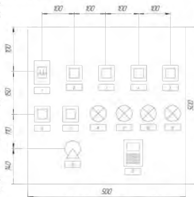
Рисунок 2.26 – Щит керування
