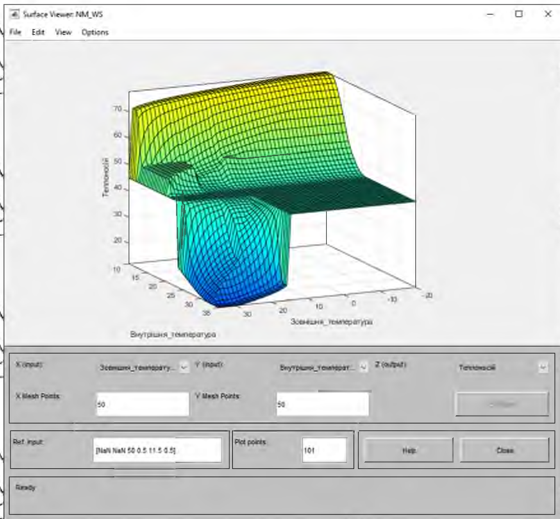
Рисунок 2.32 – Залежність температури теплоносія від зовнішньої і внутрішньої температури у теплиці
