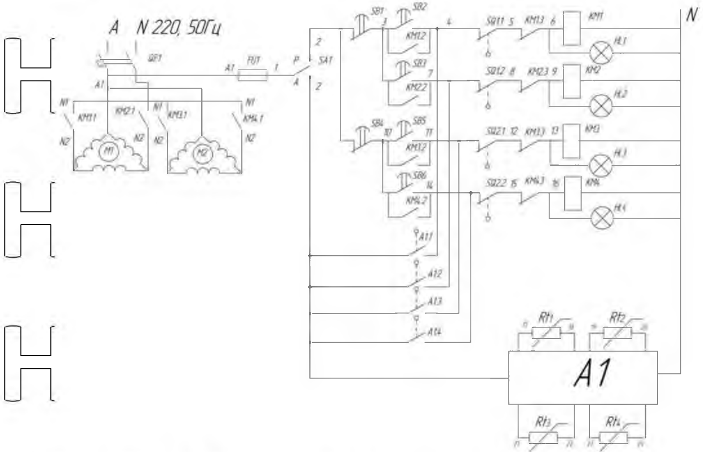
Рисунок 2.24 Принципова електрична схема досліджуваної системи
