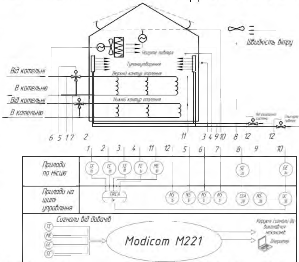
Рисунок 2.6 – Функціональна схема
