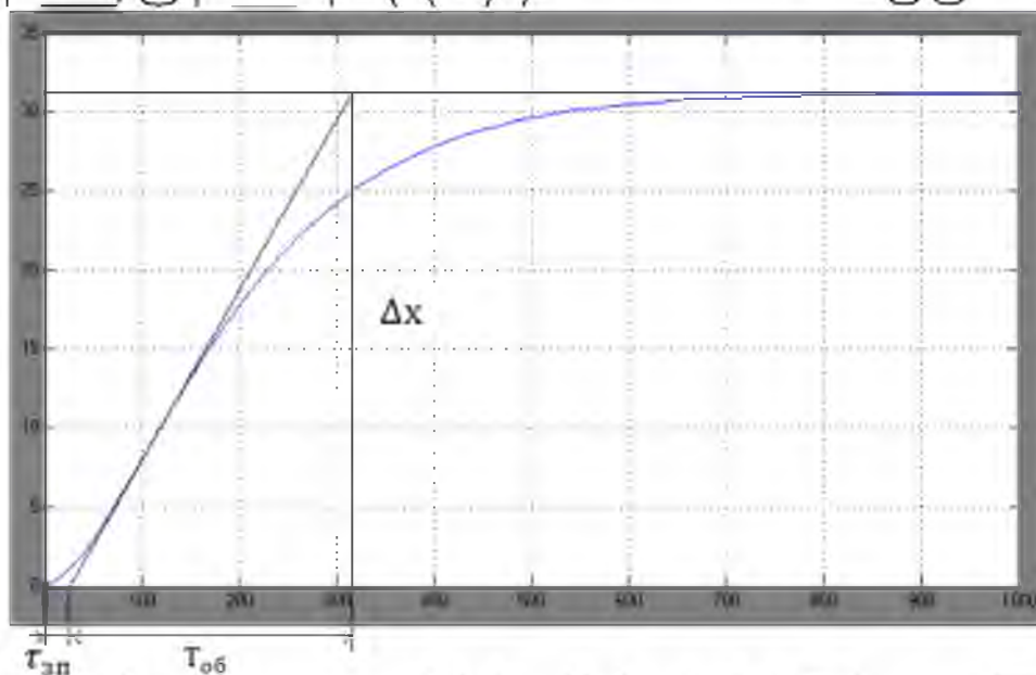
Рисунок 2.4 – Крива розгону по каналу регулювання вологості
