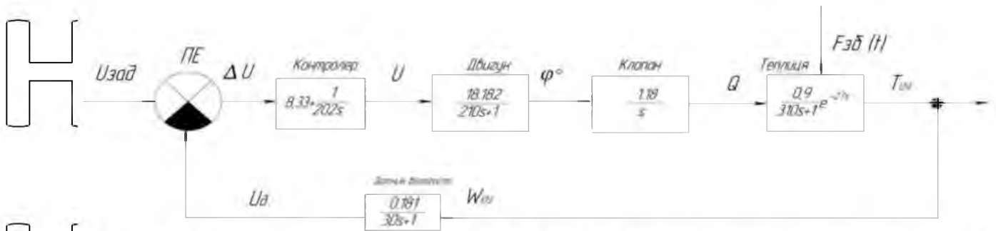
Рисунок 2.19. Структурно-алгоритмічна схема системи автоматичного керування по каналу вологості
