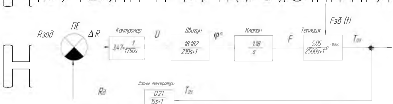
Рисунок 2.18 — Структурно-алгоритмічна схема системи автоматичного керування по каналу температури
