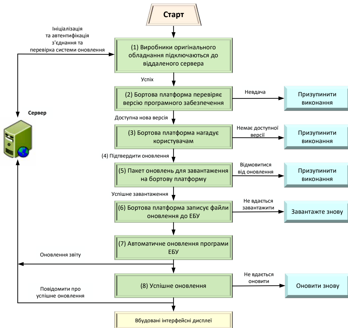
Рис. 3.1. Процес оновлення програмного забезпечення
