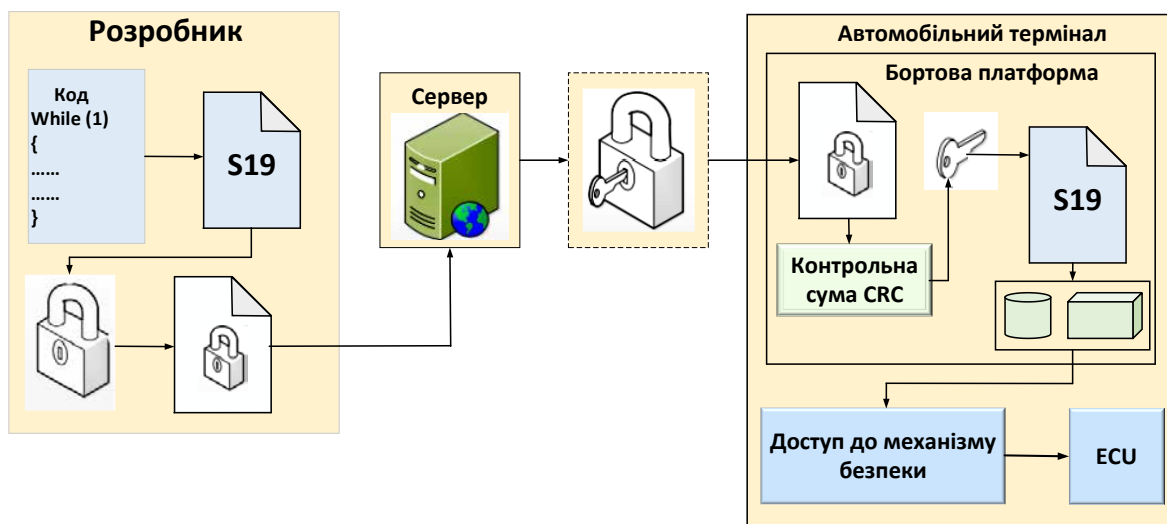
Рис. 3.2. Віддалене оновлення ПЗ з системою безпеки
