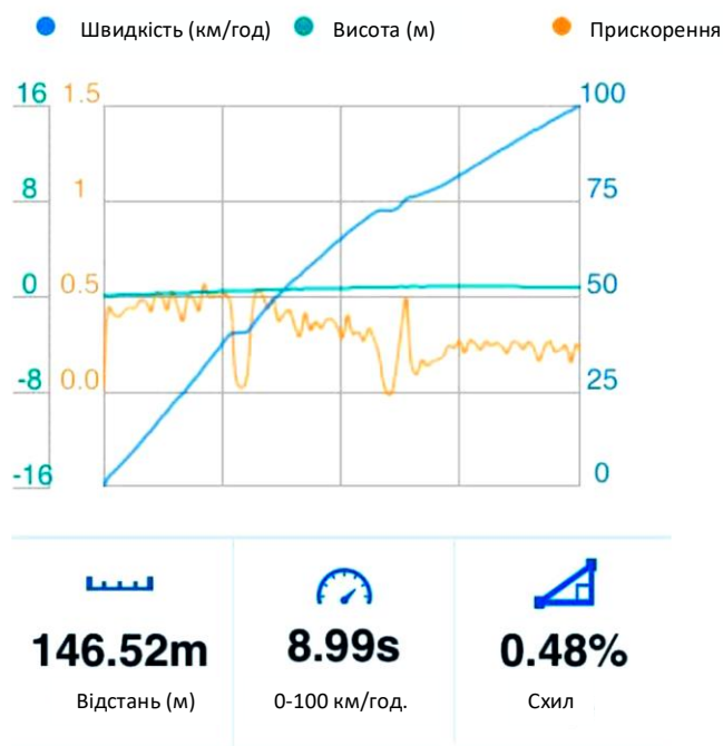
Рис. 5.7. Динаміка 0-100 км/год на програмному налаштуванні Superchips
