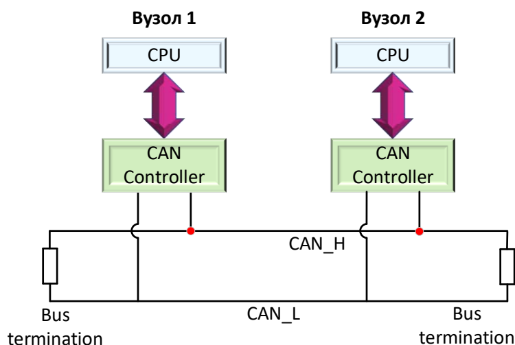
Рис. 4.1. Топологія мережі CAN
