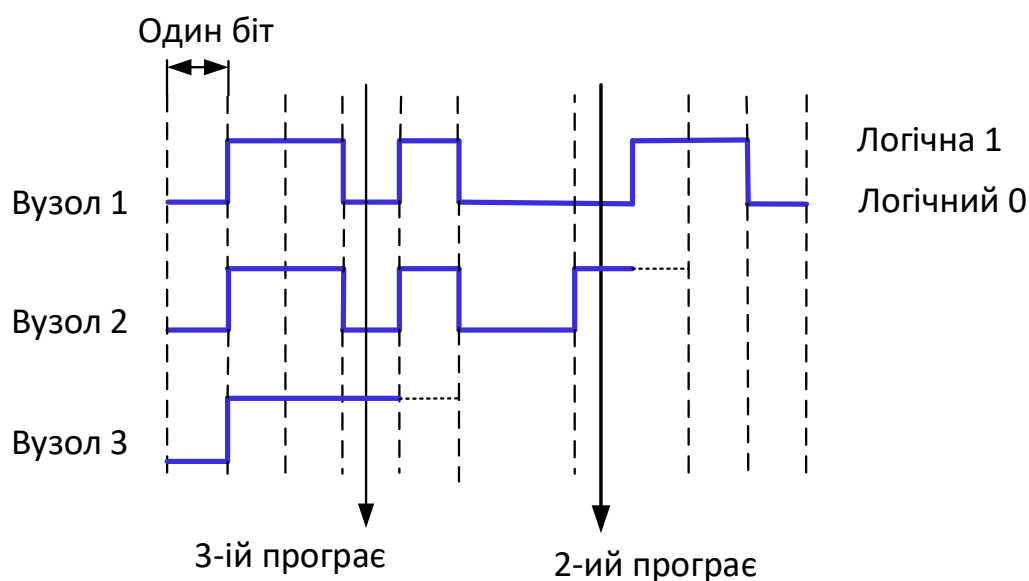
Рис. 4.3. Побітовий арбітраж на шині CAN
