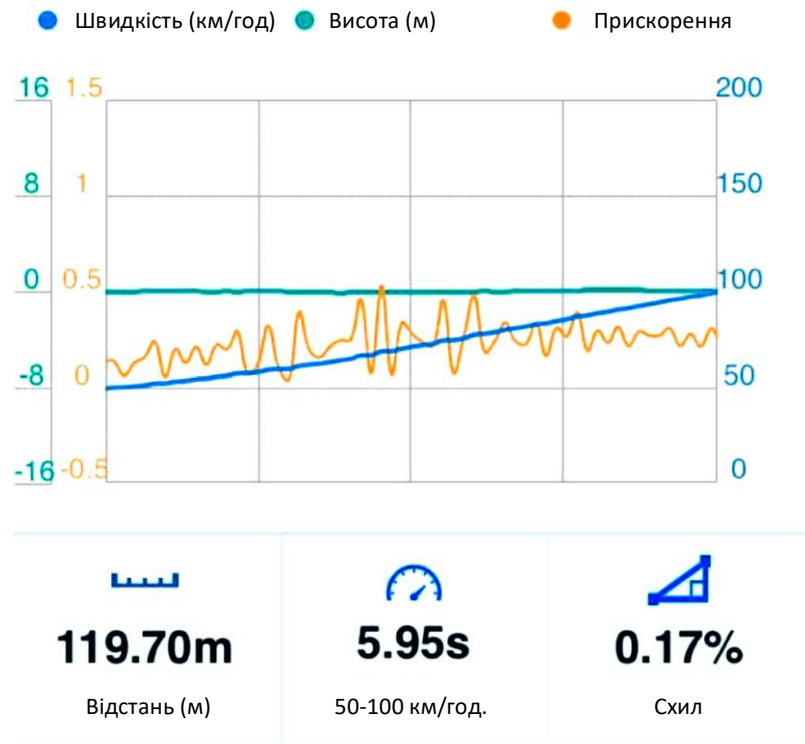
Рис. 5.5. Динаміка 50-100 км/год на покращеному програмному налаштуванні
