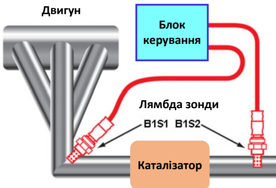
Рис. 2.2. Розміщення лямбда зондів та каталізатора
