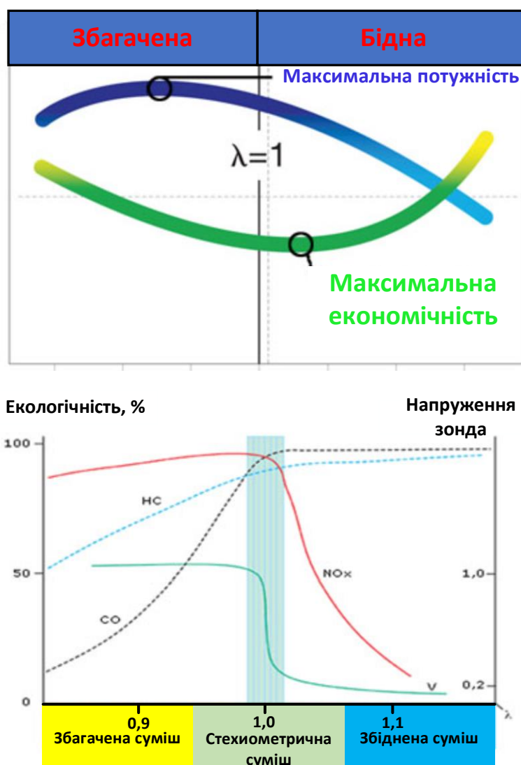
Рис. 2.1. Стехиометрична суміш.
