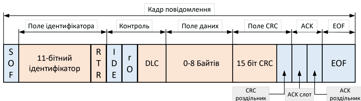
Рис. 4.2. Кадр даних стандарту CAN 2.0A
