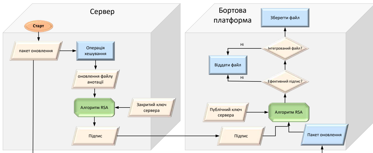
Рис. 3.3. Аутентифікація та перевірка цілісності ПЗ. Блох-схема алгоритму.
