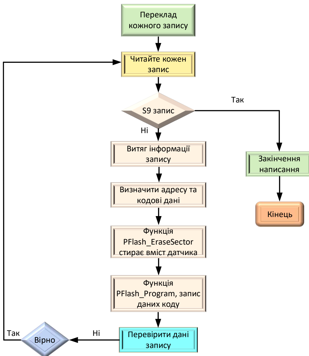
Рис. 3.7. Процес завантаження пакету оновлення сервера. Блок-схема алгоритму
