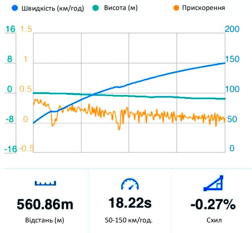
Рис. 5.6. Динаміка 50-150 км/год на покращеному програмному налаштуванні
