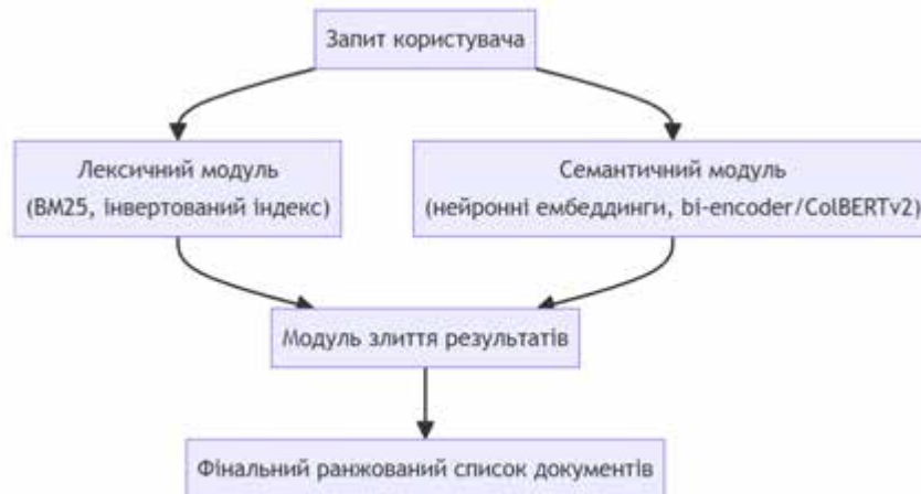
Рис. 1. Узагальнена архітектура гібридної моделі нейронного пошуку
