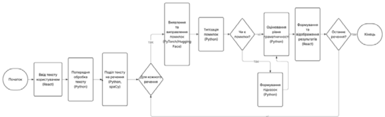
Рисунок 1. Алгоритм, що реалізує запропонований підхід до перевірки та коригування тексту з використанням штучного інтелекту
