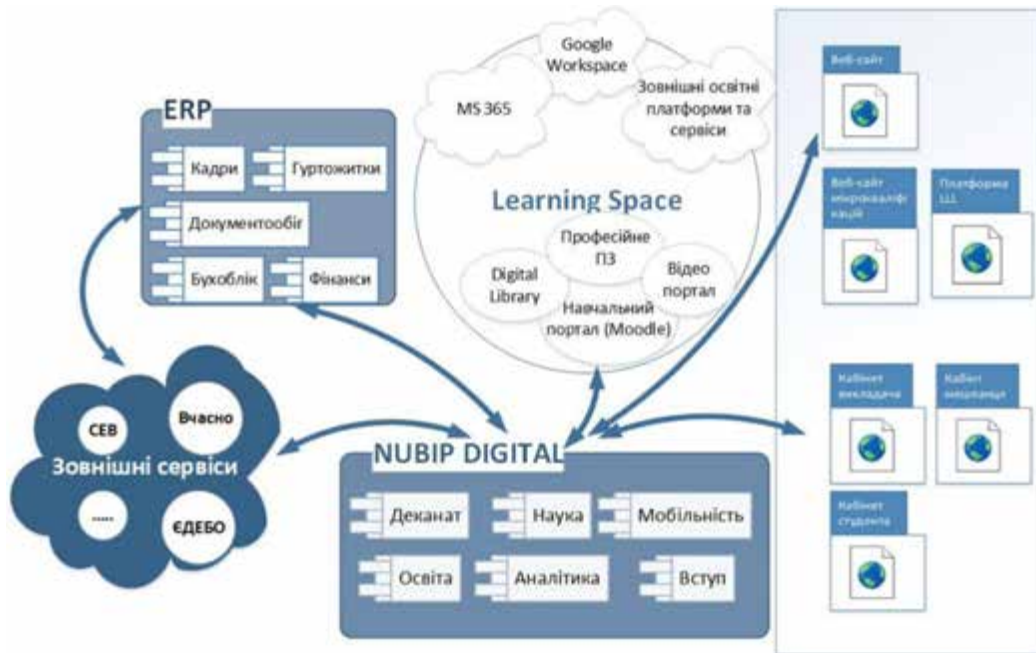
Рис. 1. Архітектура цифрового освітнього середовища НУБіП України
