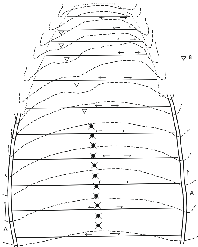
Рис. 13.2. При слабовипуклих горизонталях на міжулоговинно-міжбалковій частині орного земельного масиву безпечне відведення стоку забезпечується прямолінійними (або близькими до прямолінійних) рубежами.
