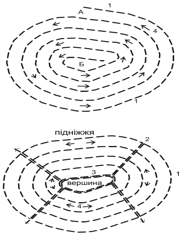
Рис. 13.10. Організація території поверхні куполоподібного підвищення (без істотного вздовжсхилового розчленування): вгорі — контурно-спіральна; внизу — у вигляді схилових блоків контурно-смугових робочих ділянок:
