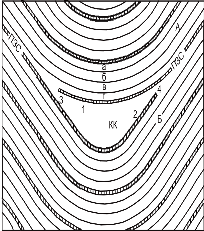
Рис. 13.12. Розміщення полежахисних лісосмуг (ПЗС), які обмежують контурно-смугові робочі ділянки (А, Б та ін.) з коректуючим клином (КК) поміж ними (у даному випадку між ділянками А і Б).
