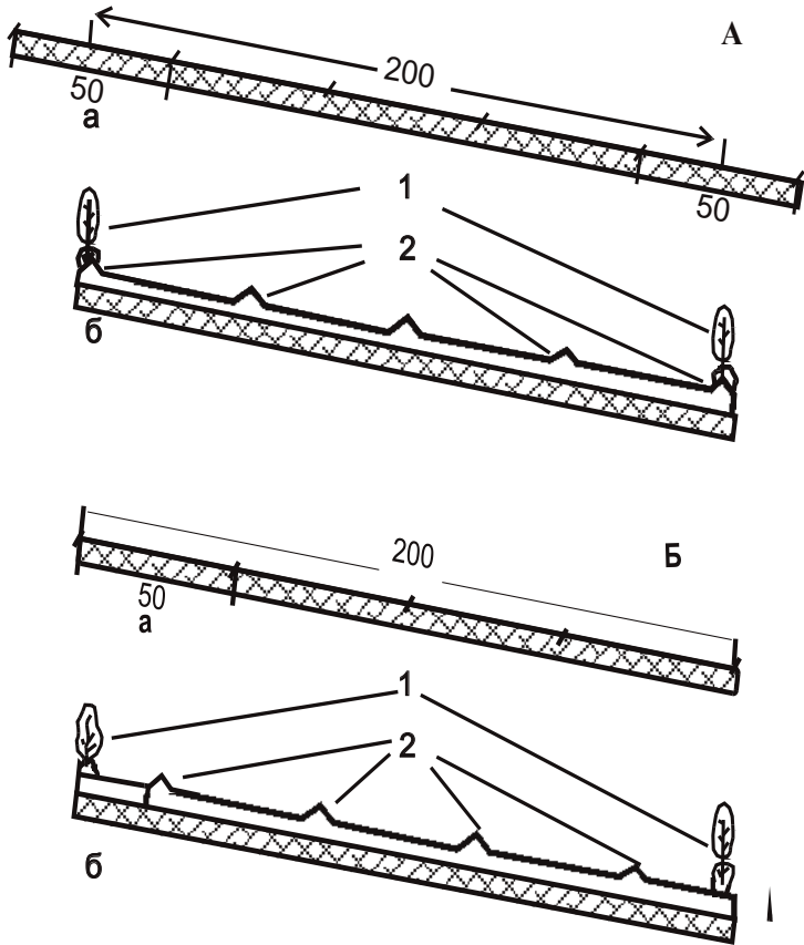
Рис.13.11. Схеми двох варіантів (А і Б) поділу 200-метрової ширини контурно-смугової робочої ділянки для розміщення поздовжніх смуг (кожна завширшки 50 м) з метою докорінної меліорації мікрорельєфу поля з попереднім зняттям гумусованого шару ґрунту й поверненням після планування поверхні та створення валів-терас (а), а також відповідного розміщення валів-терас (б).
