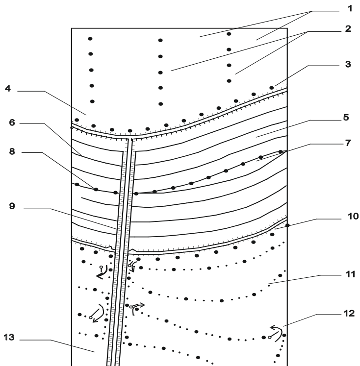
Рис. 13.5. Ілюстративний приклад деталізованого плану розміщення заходів постійної дії на місці стику мікрозони А з двома схилливими блоками контурно-смугових робочих ділянок, орних і пасовищних
