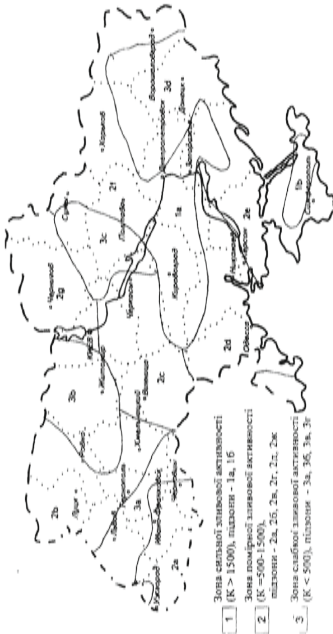
Рис.11.1. Зливової небезпека на території України
