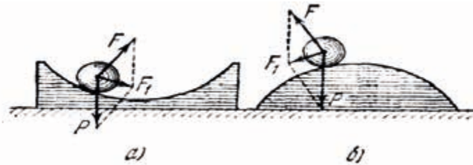
Рис 3.1. Стійка (а) та нестійка (б) рівновага кульки на поверхні
