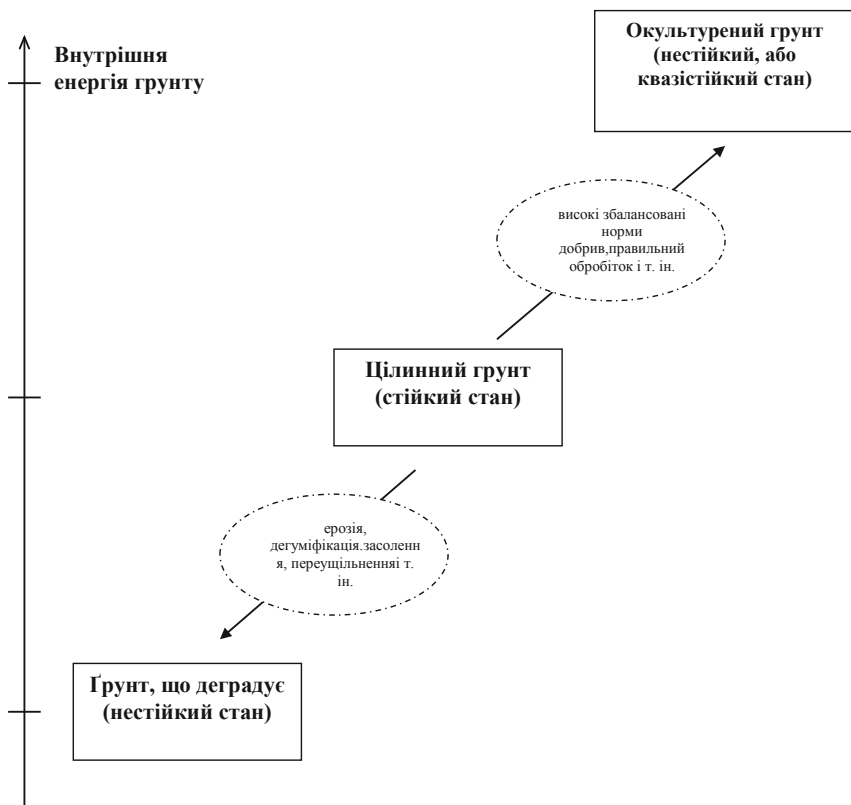
Рис. 3.2. – Схема зміни станів ґрунту
