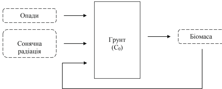
Рис. 3.4. – Схема основних статей енергетичного балансу в цілному автоматичному ґрунті
