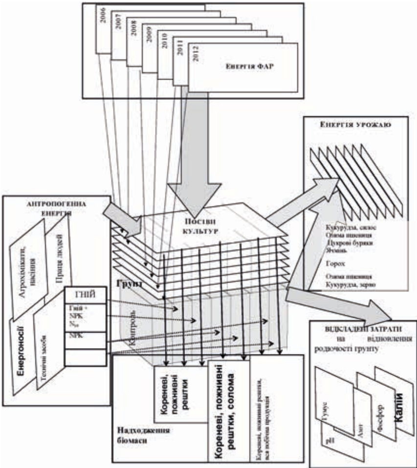
Рис. 15.1 Методичні принципи визначення енергетичної ефективності систем землеробства (на прикладі стаціонарного дослідження Полтавського ІАПВ)
