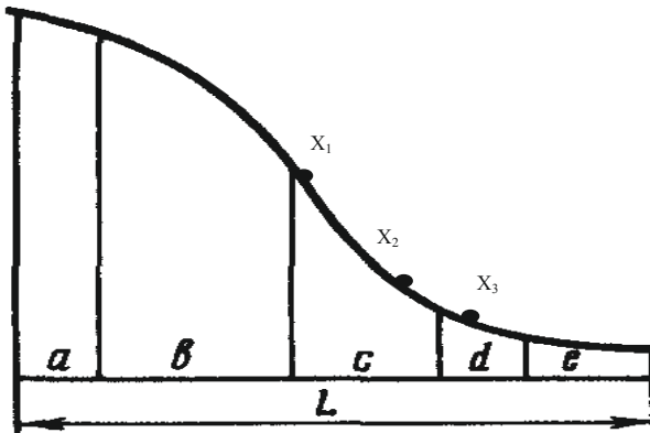
Рис.14.1. Схилувий ряд місцеположень (складено за Боковим В.О.) Частина схилу: а - привододільна; b - верхня; c - середня; d - нижня; e - підніжжя. Відстань L відповідає п'яти позиційним одиницям.
