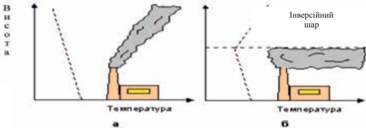
Рис. 14.8. Розсіювання викидів у нормальних умовах (а) і при інверсії (б)
