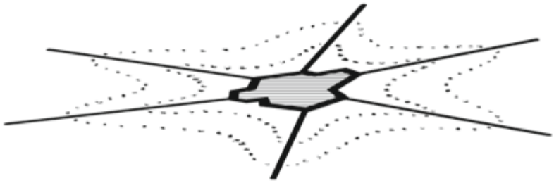
Рис.14.6. Схематична карта ізохрон (пунктир) навколо міста (заштриховане), витягнутих уздовж транспортних магістралей (суцільні лінії).
