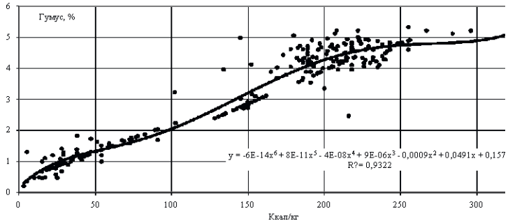
Рис. 15.2 – Залежність між питомою теплою горіння різних типів ґрунтів
