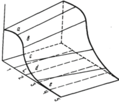
Рис.14.2. Співвідношення метричних мір (1,2,3,4,5) і позиційних мір (а,b,c,d,e) нахилі (складено за В.А. Боковим)
