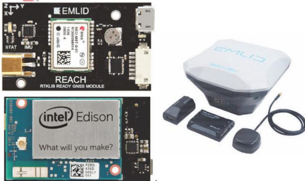
Рис. 7.2.10 Плати та повний комплект системи Reach RTK
