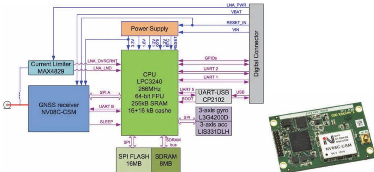
Рис. 7.2.7 Прецензійний навігаційний модуль NV08C-RTK
