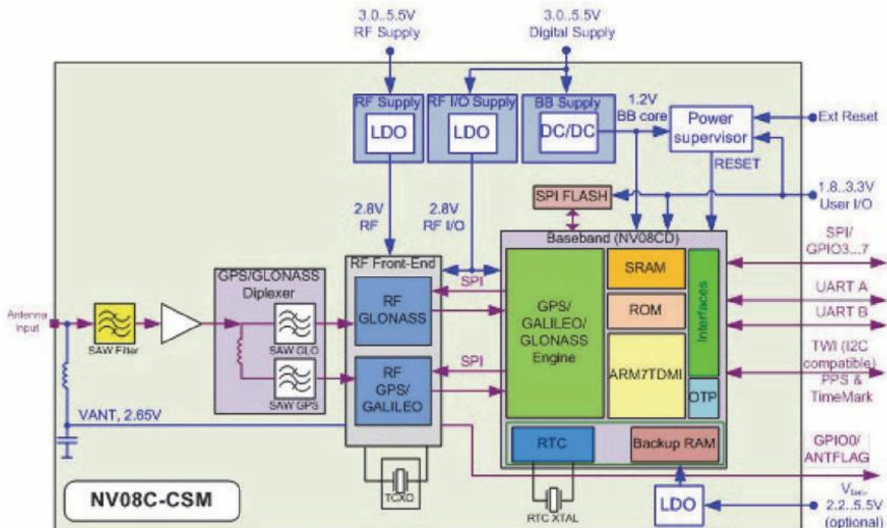
Рис. 7.2.6. Схема плати модуля з позначенням основних вузлів GPS/GLONASS-NV08C-CSM
