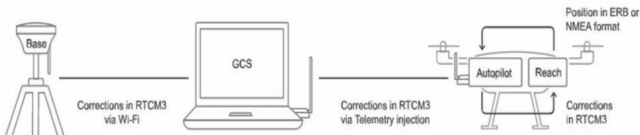
Рис. 7.2.8 Система RTK для БПЛА
