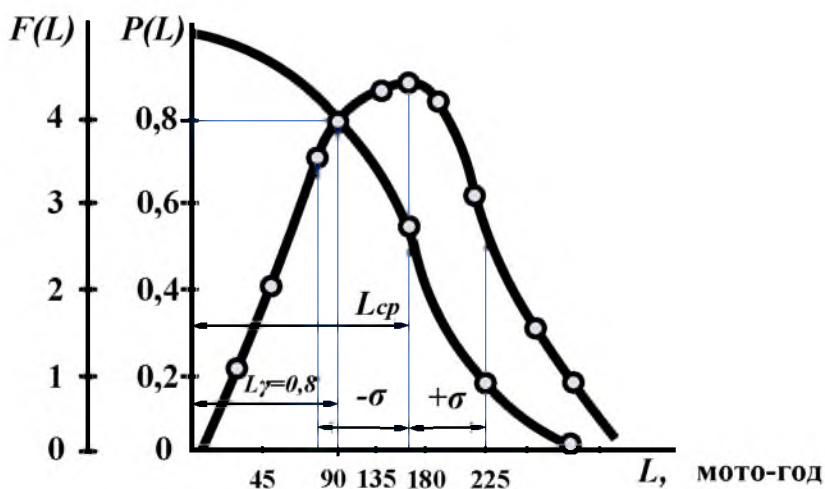
Рис. 2. Графік ймовірності характеристик ресурсу двигунів Д-260.9 до першого капітального ремонту в умовах третьої категорії експлуатації: P(L) – ймовірність роботи без капітальних ремонтів; F(L) – щільність розподілу капітальних ремонтів; \sigma – параметр нормального закону розподілу
