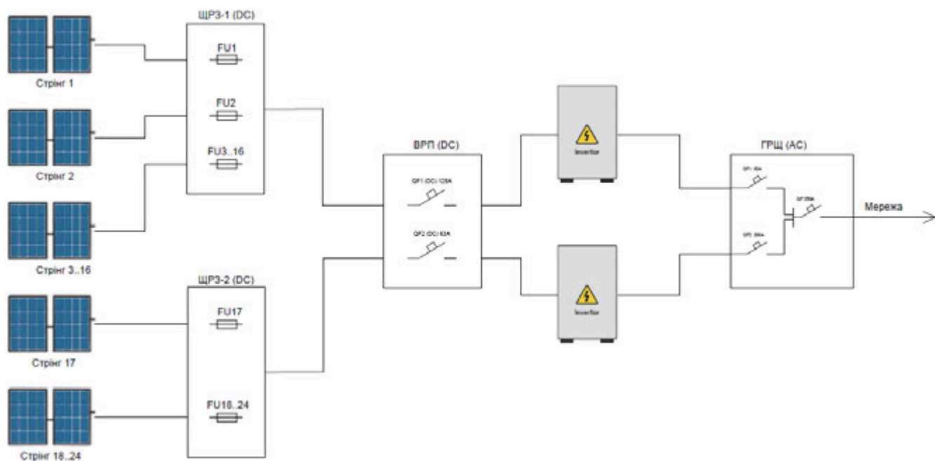
Рис. 3.3 Принципова електрична схема функціонування СЕС
