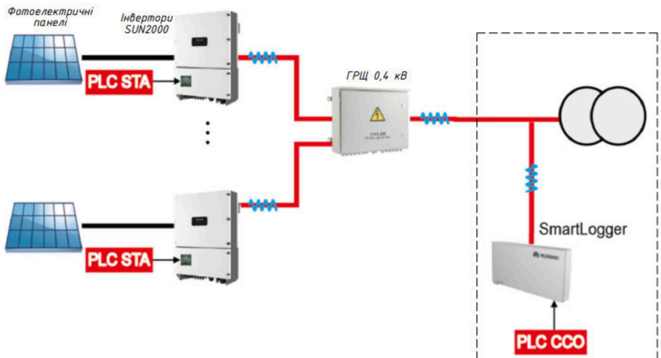
Рис. 3.4. Схема мережевого зв'язку по силовим кабелям
