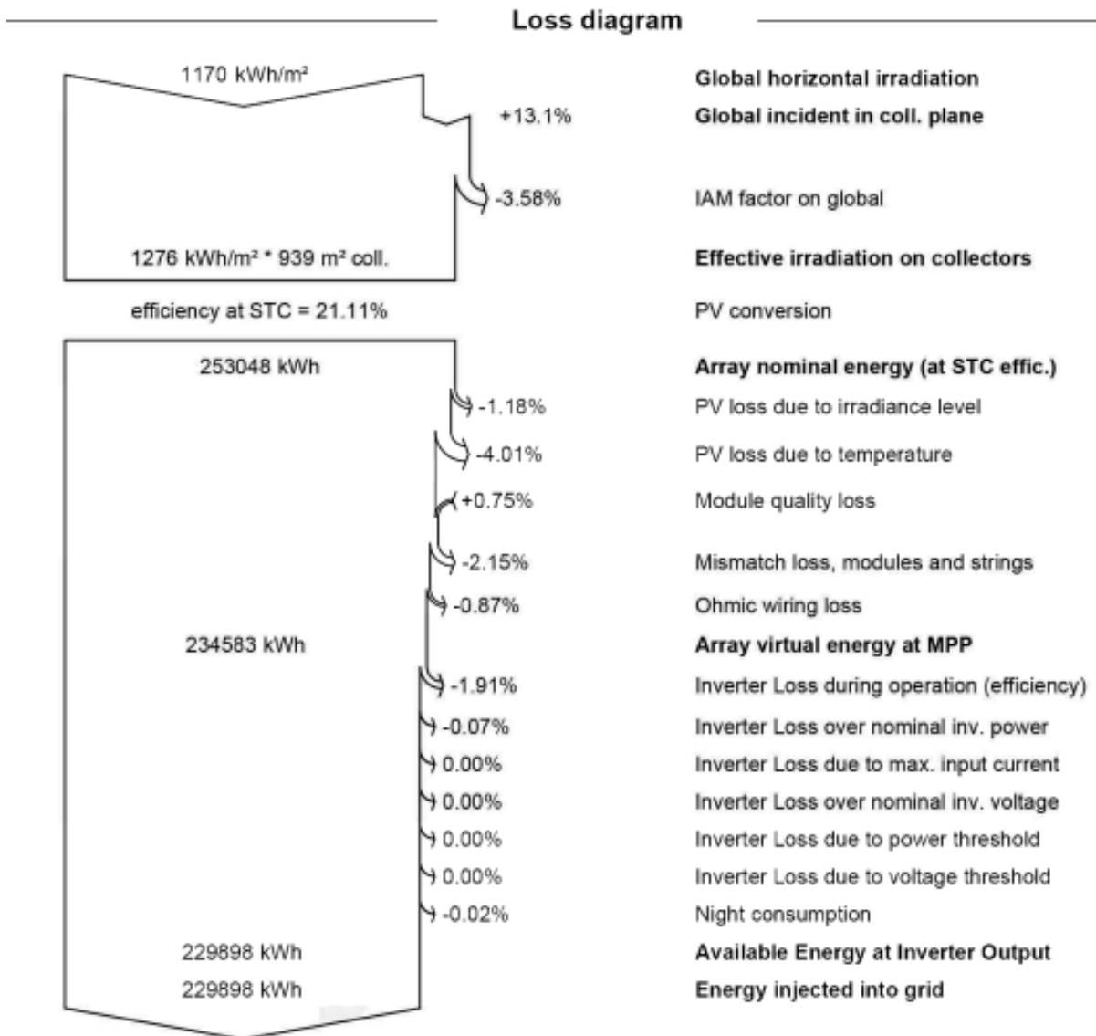
Рис. 5.4. Діаграма втрат
