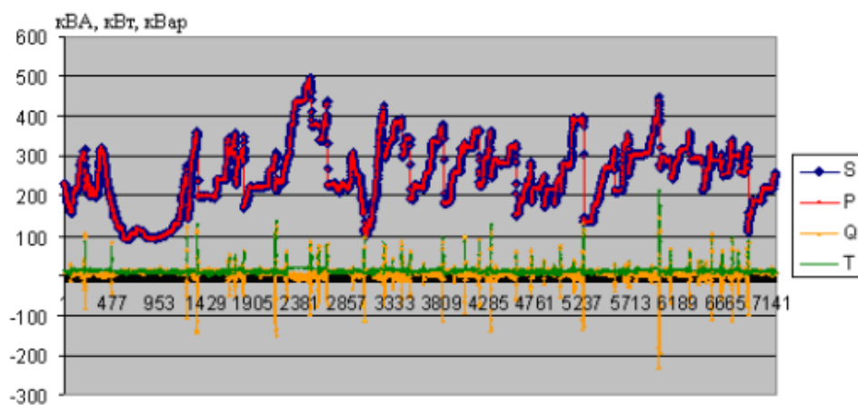
Рис. 2.5. Динаміка зміни активної та реактивної потужностей на затискачах ТП СЕС
