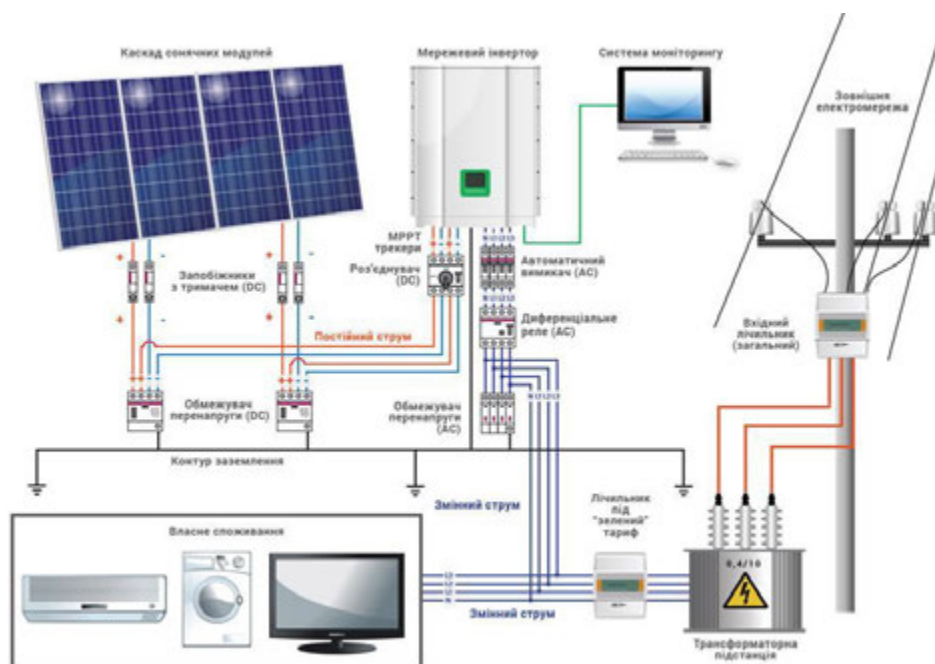
Рис. 2.2. Функціональна схема роботи СЕС
