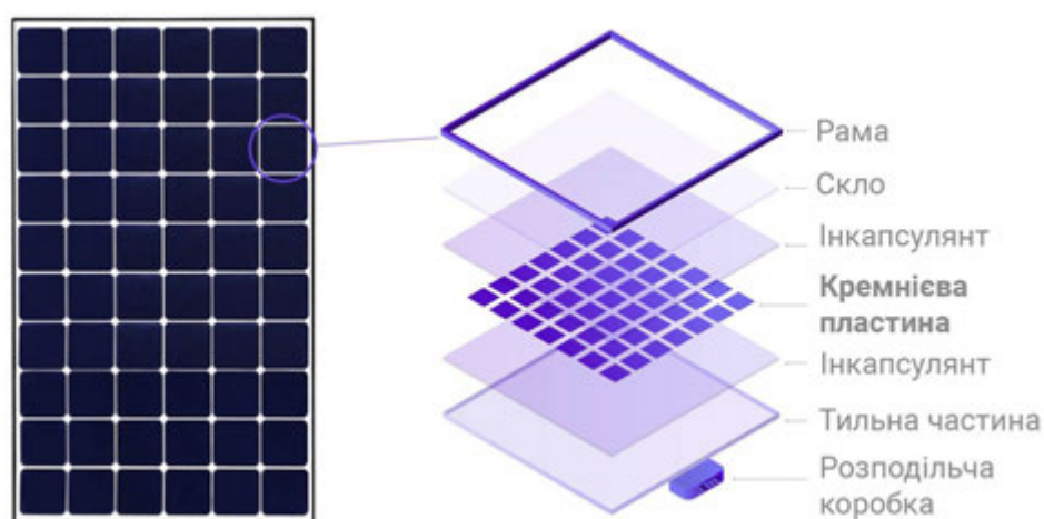
Рис. 2.3. Будова фотомодуля
