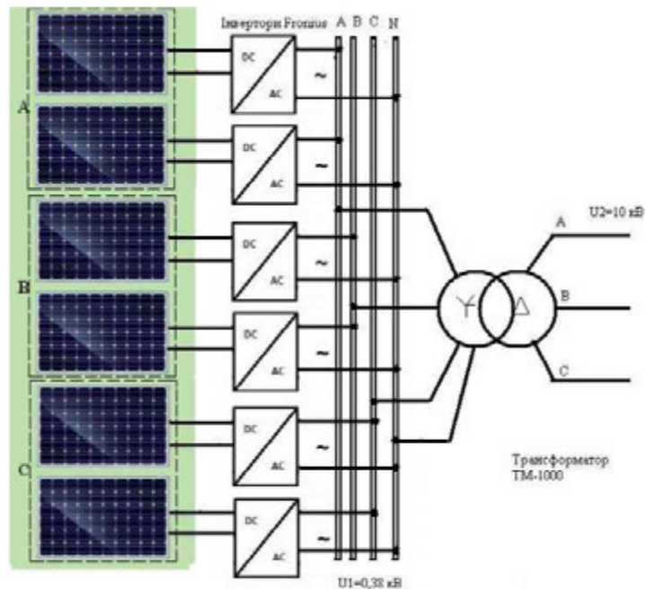
Рис. 2.4. Принципова схема підключення інверторів Fronius
