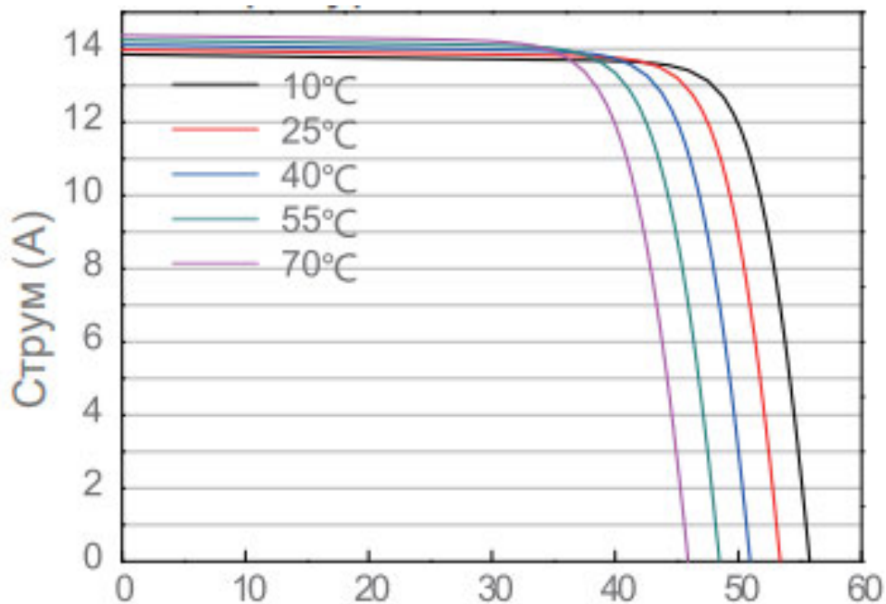
Рис. 5.7. ВАХ в залежності від температури JAM72S30-595/MR
