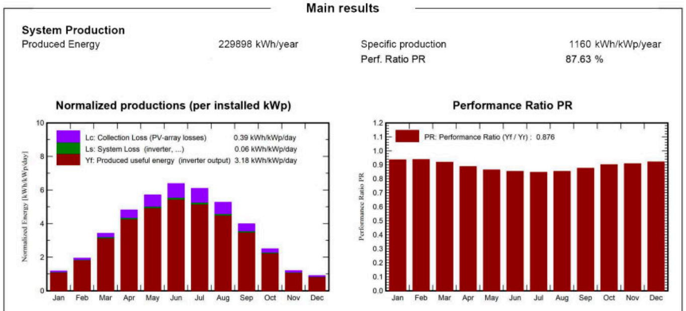
Рис. 5.5. Графіки виробітку електричної енергії
