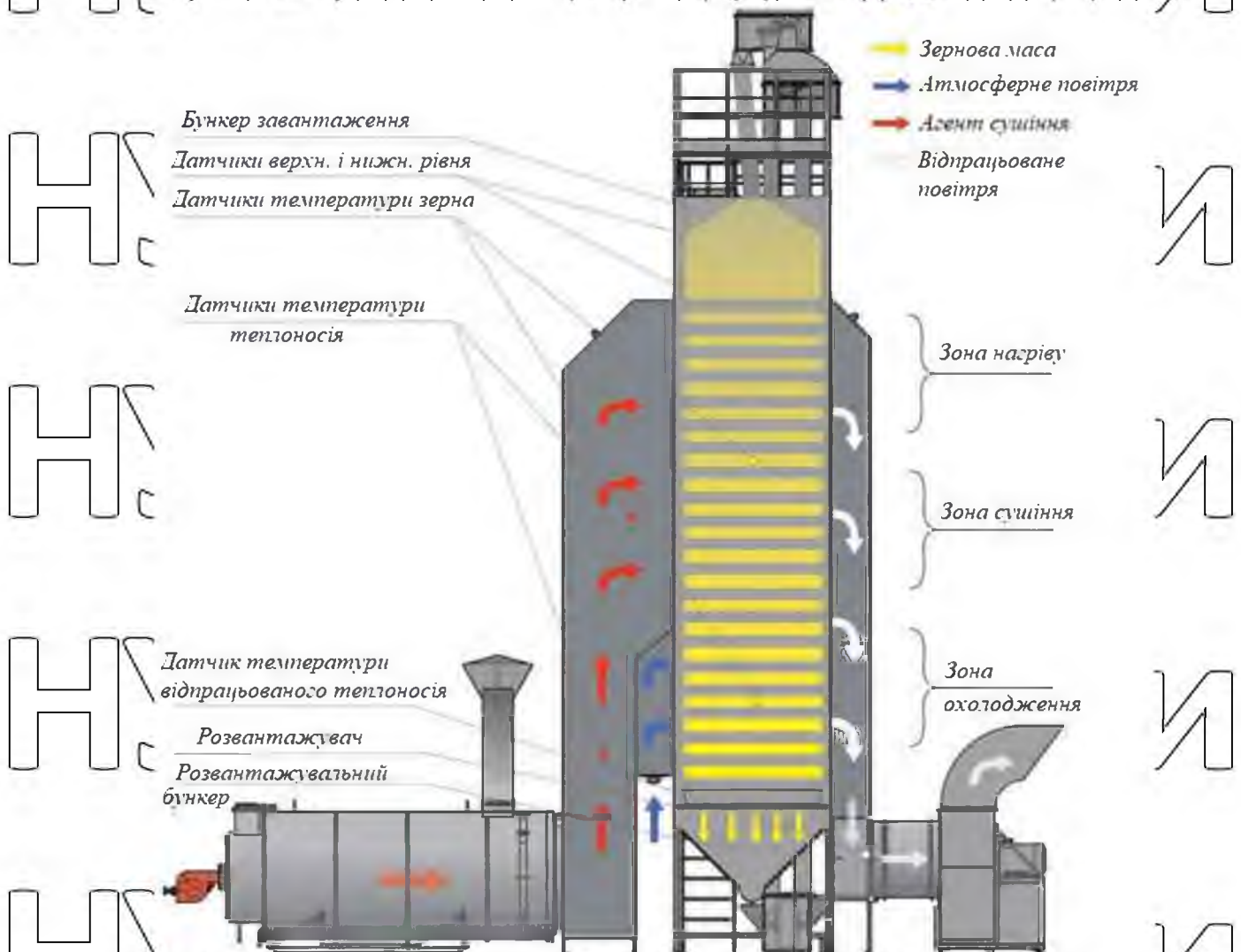
Рис. 1.4. Конструкція шахтної зерносушарки
