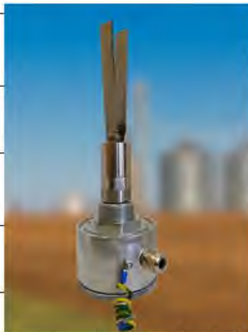
Рис. 3.5 Датчик граничного рівня сипких матеріалів ДПУ-10
