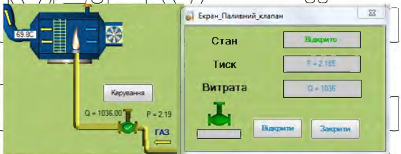
Рис. 6.5. Вікно керування пальником теплогенератора в ручному режимі
