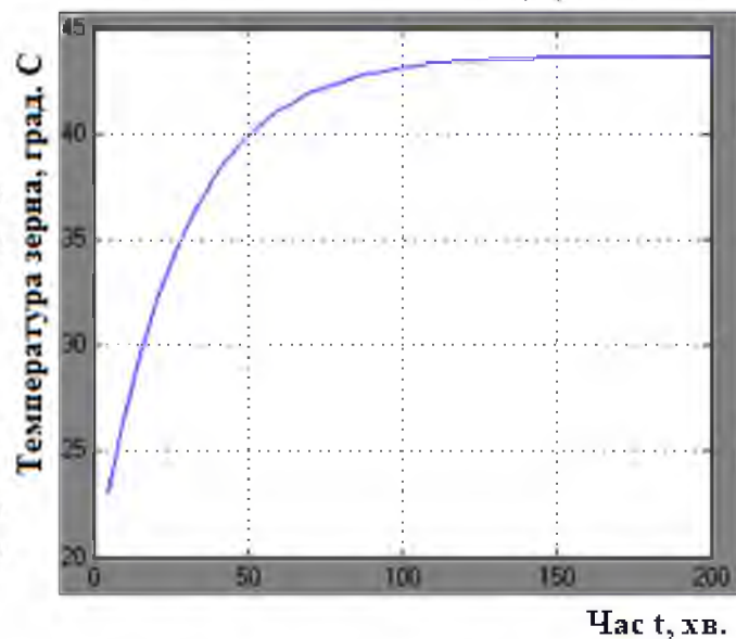
Рис. 2.4. Зміна температури зерна під час сушіння
