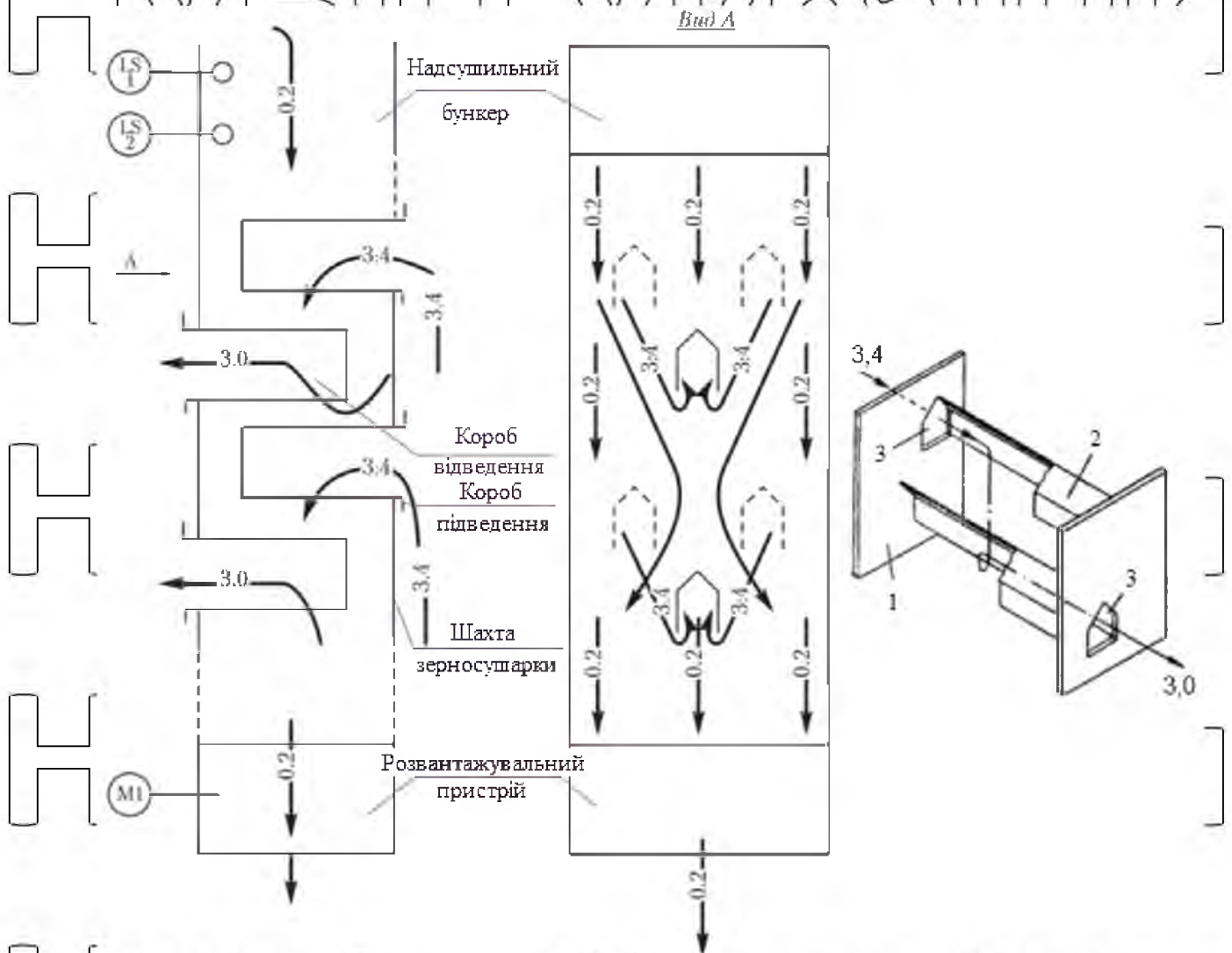
Рис. 1.3. Технологічна схема сушіння зерна у шахтній зерносушарці
