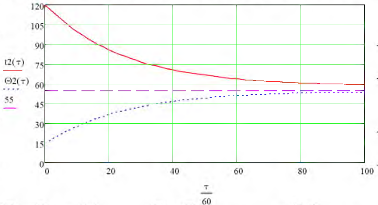
Рис. 2.10. Зміна температури агента сушіння та шпаканій зерносушарки при нагріванні зерна від 15^{\circ}\text{C} до 54^{\circ}\text{C}
