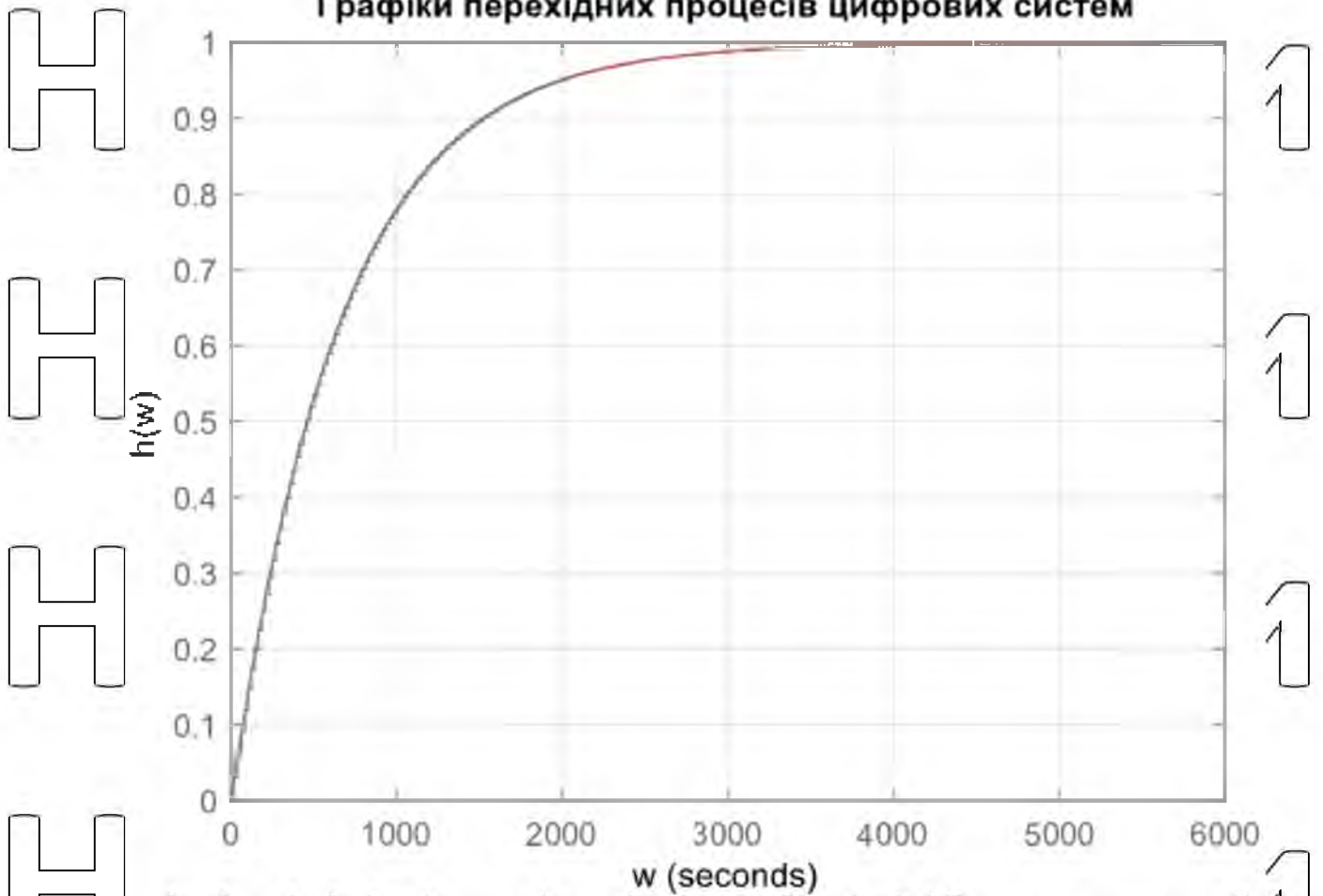
Рис. 4.3. Перехідний процес САК температурним режимом сушіння зерна у шахтній зерносушарці
