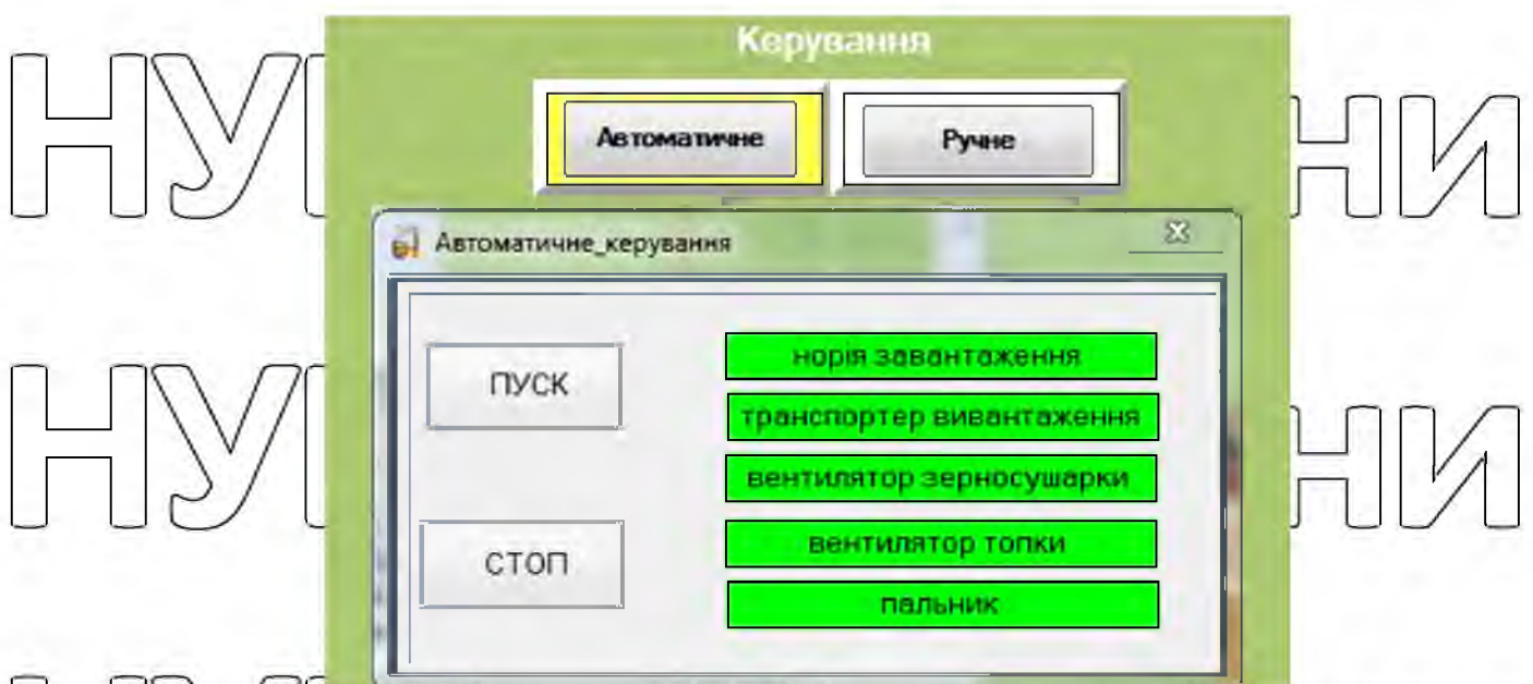
Рис. 6.3. Перемикач режимів роботи (автоматичний/ручний)
