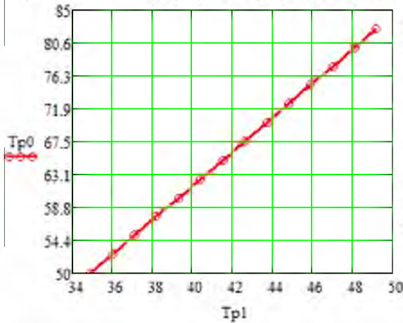
Рис. 2.8. Зміна температури сушильного агента під час сушіння при постійній витраті вологого зерна G_z = 2,1 \text{ кг/с}
