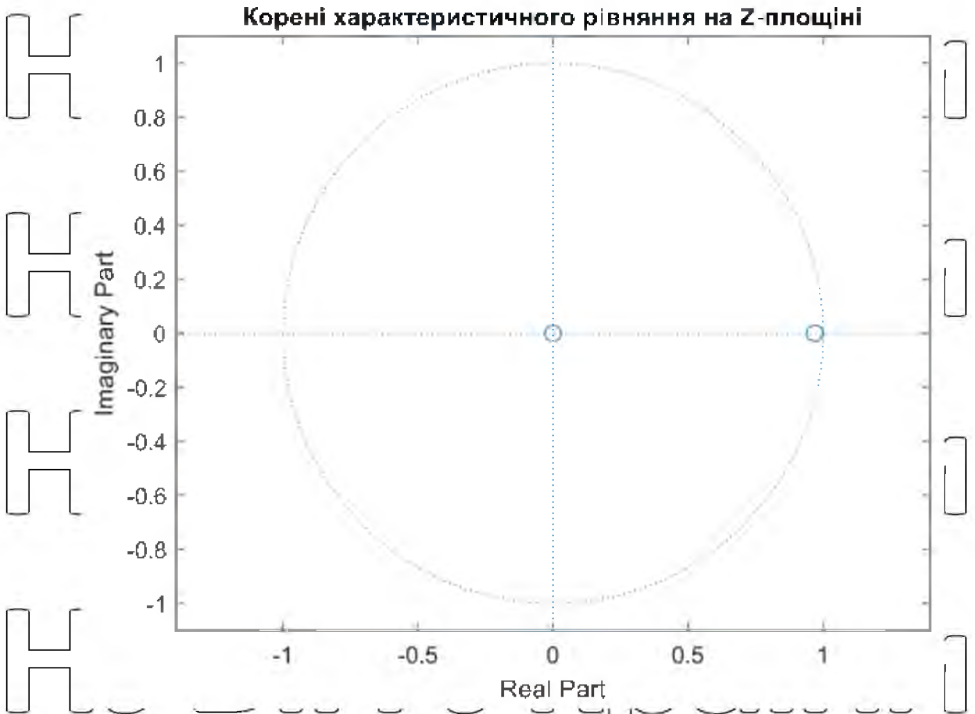
Рис. 4.2. Корені характеристичного рівняння на z-площині
