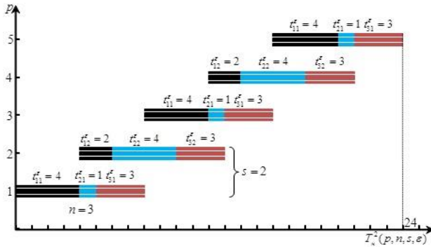
Рис. 3.10 – Функціонування micro grid при p=5 , n=3 , s=2
