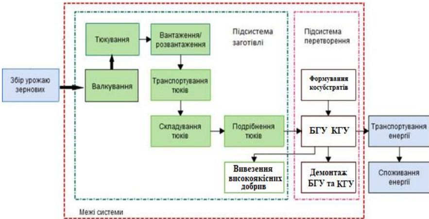
Рисунку 4.16 – Узагальнена схема життєвого циклу використання СВ у тюках для їх зброджування у БГУ та виробництва електричної та теплової енергії у КГУ
