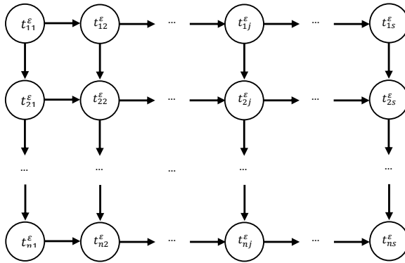
Рис. 3.5. Мережевий вершинно-зважений граф G_1^{ac}
