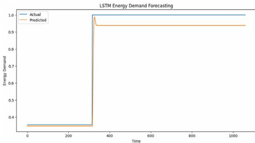
Рисунок 5.21 –Візуальне представлення різниці між фактичним та прогнозованим попитом на теплову енергію для моделі довгої короткочасної пам’яті в Смілянській громаді
