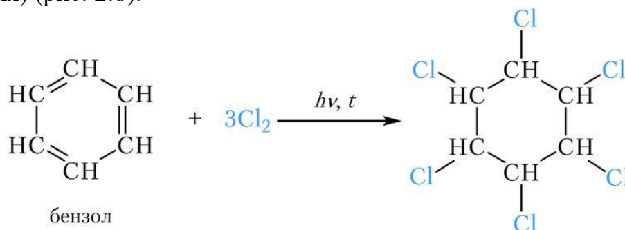
Рис. 2.8. Структурна формула 1,2,3,4,5,6-гексахлорциклогексан (ГХЦГ)
