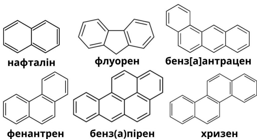
Рис. 2.9. Структурні формули найбільш небезпечних поліадерних ароматичних вуглеводнів
