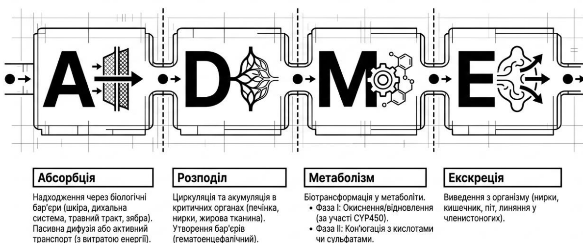
Рис. 1.4. Модель ADME
