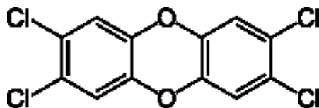
Рис. 2.6. Структурна формула 2,3,7,8-тетрахлордibenзо-пара-діоксина (2,3,7,8-ТХДД)
