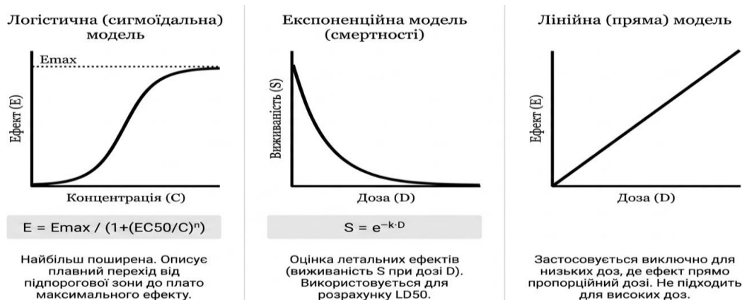
Рис. 1.10. Найбільш поширені моделі в екотоксикології
