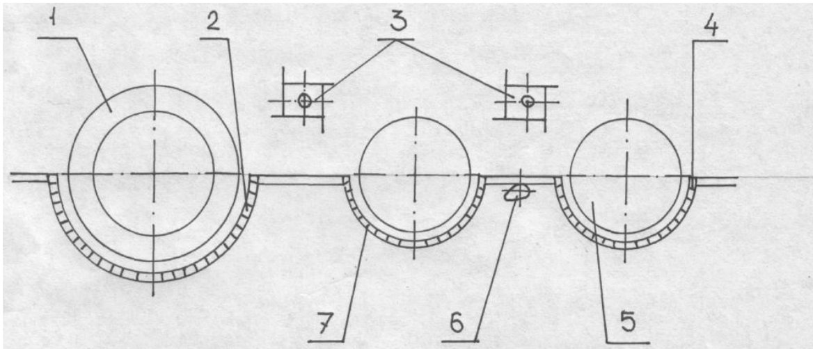
Рисунок 4.3 - Схема молотильно-сепаруючого пристрою роторного типу: 1 - молотильний барабан; 2 - підбарабання; 3 - відбійний бітер; 4 - решітка; 5 - ротор; 6 - кулачковий вал; 7 - решітка
