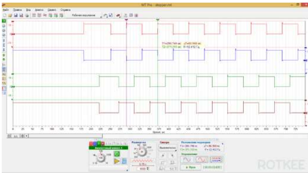
Рис. 4.4 Вторинна напруга.
