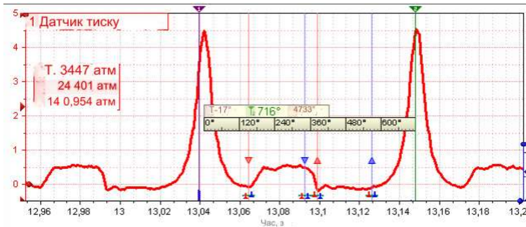
Рис. 4.13 Той самий сигнал з використанням настройки (всі значення в Атм, кут випередження запалення 17^\circ )
