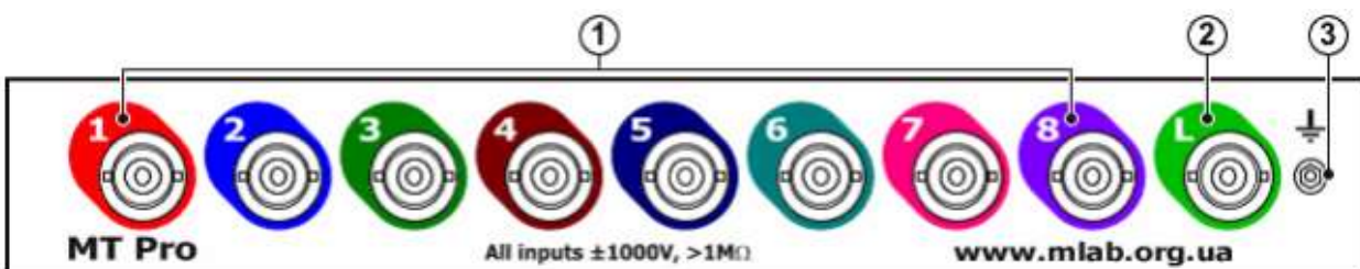
Рис. 3.1 Підключення передньої панелі вимірювального блоку MT Pro.
