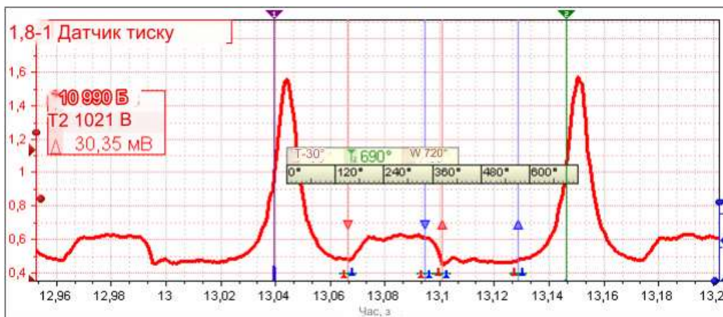
Рис. 4.12 Сигнал з датчика тиску без використання налаштування аналогового каналу.
