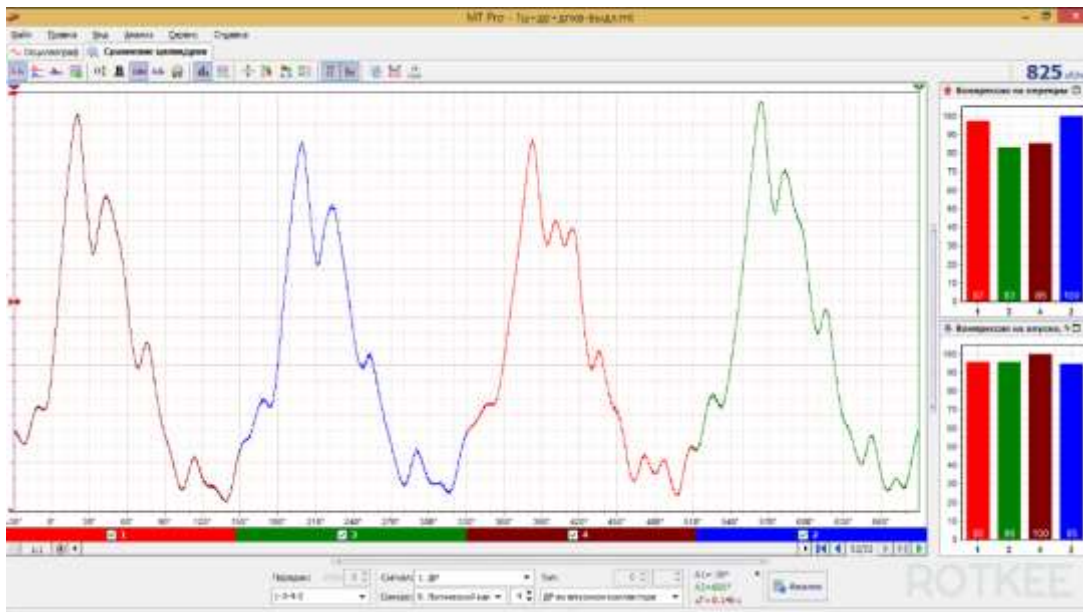
Рис. 4.7 Порівняння циліндрів.
