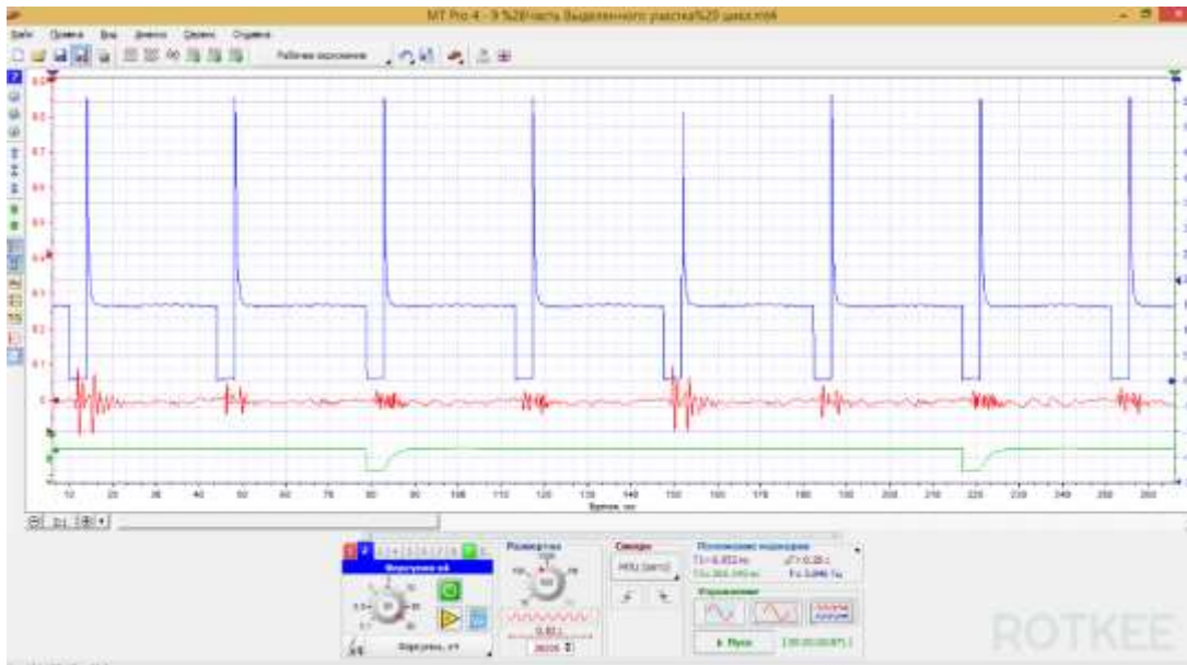
Рис. 4.3 Осциллограф
